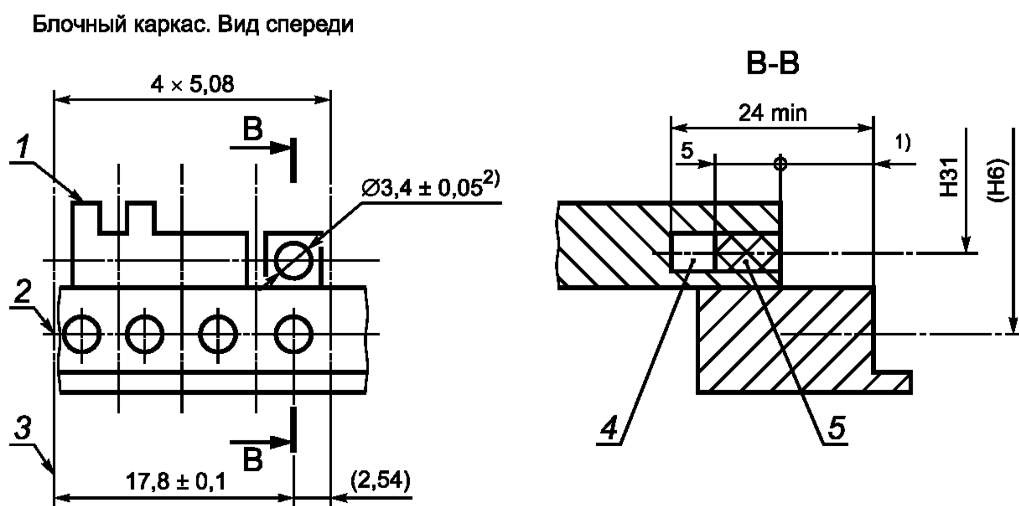
1 — типовая направляющая; 2 — горизонтальная деталь блочного каркаса; 3 — линия шага выводов; 4 — гнездо для установки центрирующего ловителя; 5 — область контакта
