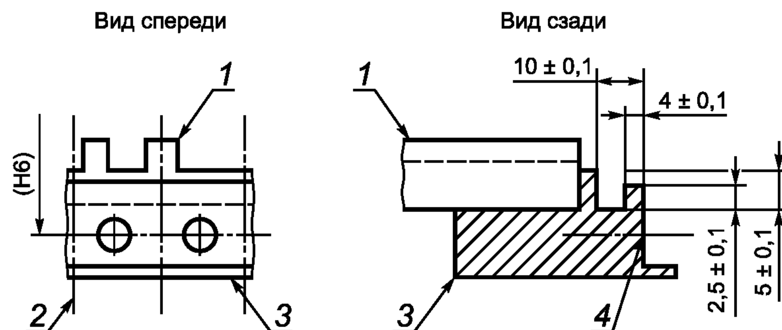
1 — направляющая; 2 — горизонтальная линия шага выводов; 3 — горизонтальная деталь блочного каркаса; 4 — передняя плоскость закрепления
