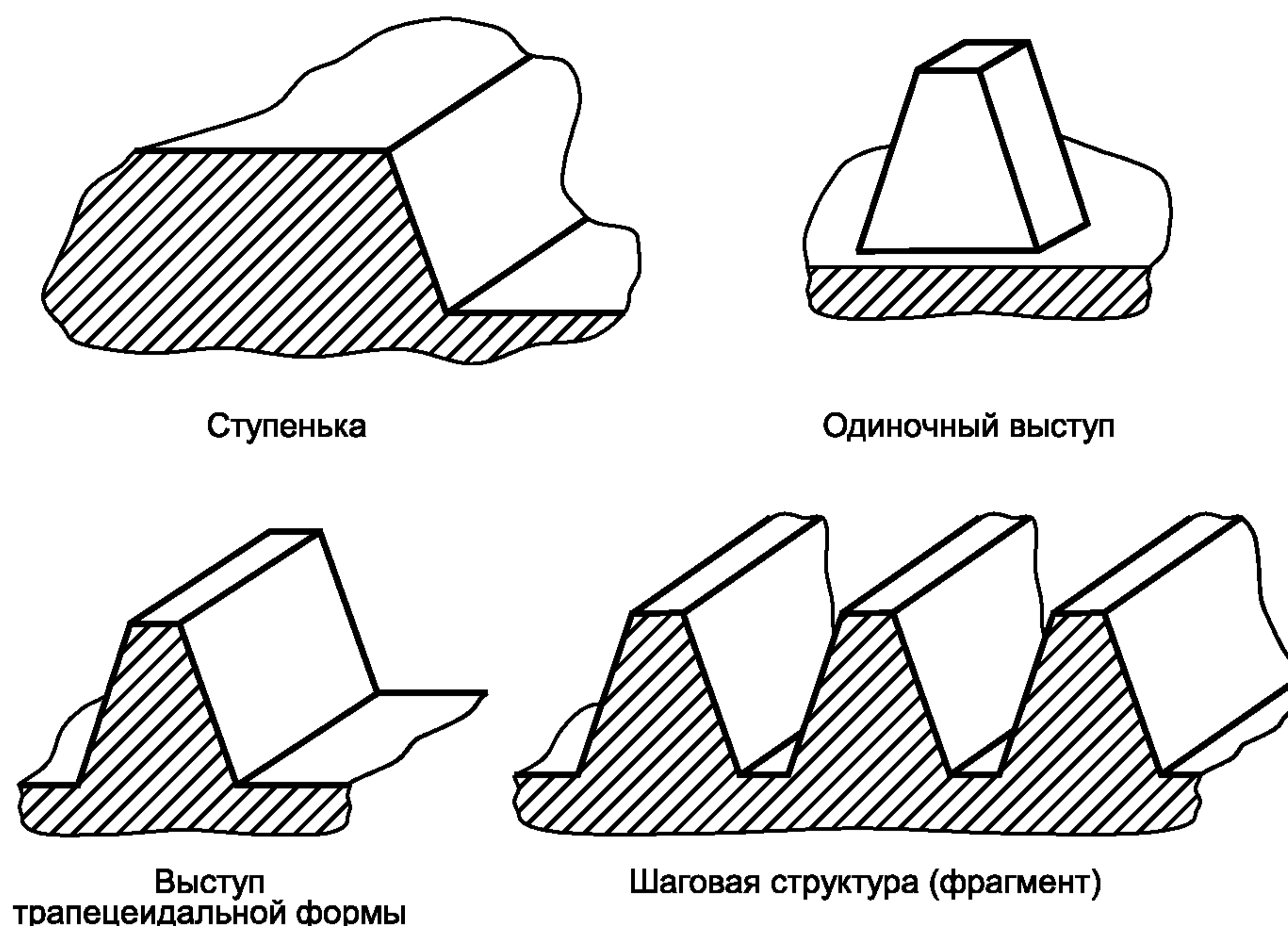
Рисунок 1 — Типовые элементы рельефа рельефной меры
