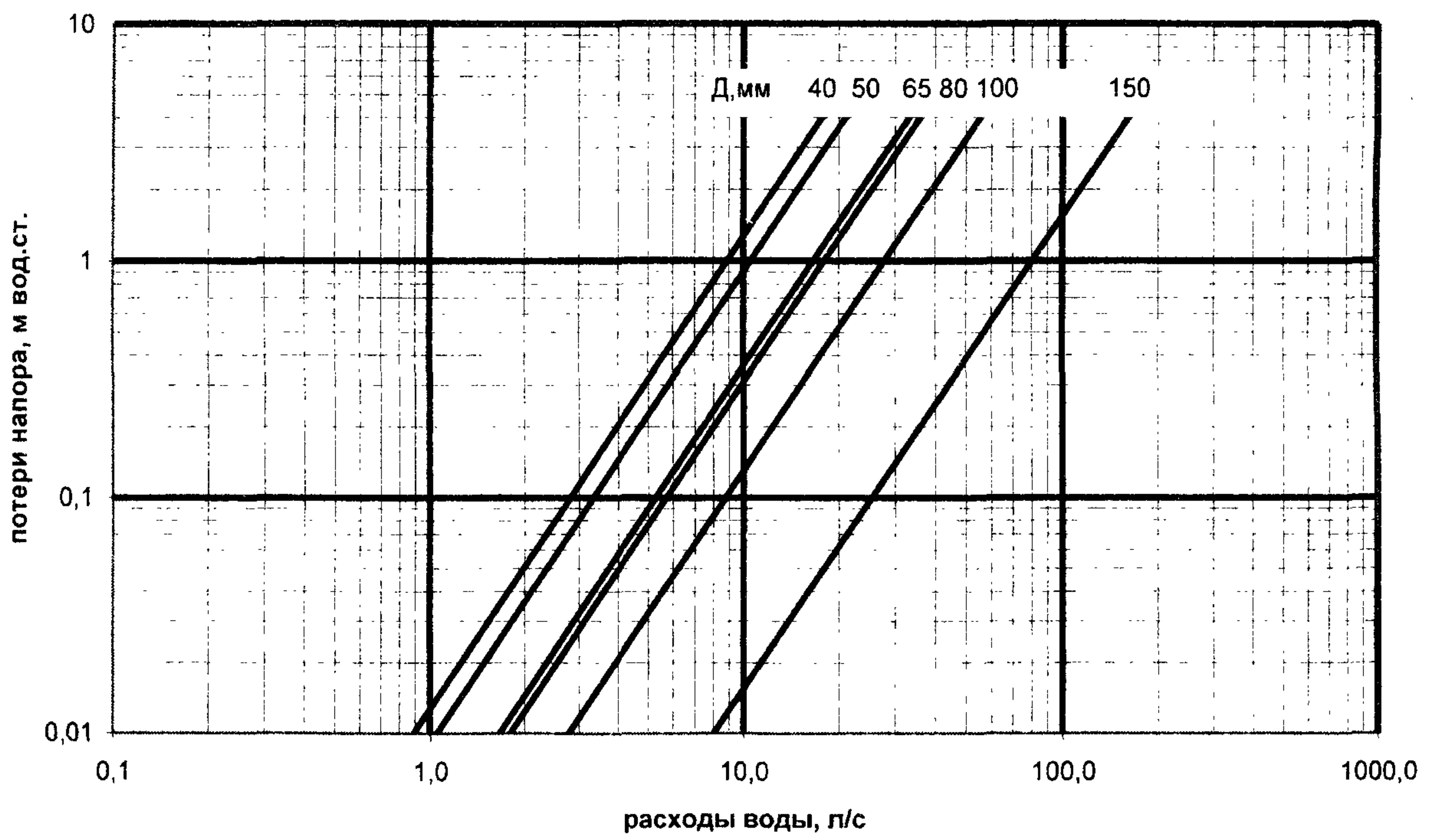
потери напора в турбинных счетчиках воды
