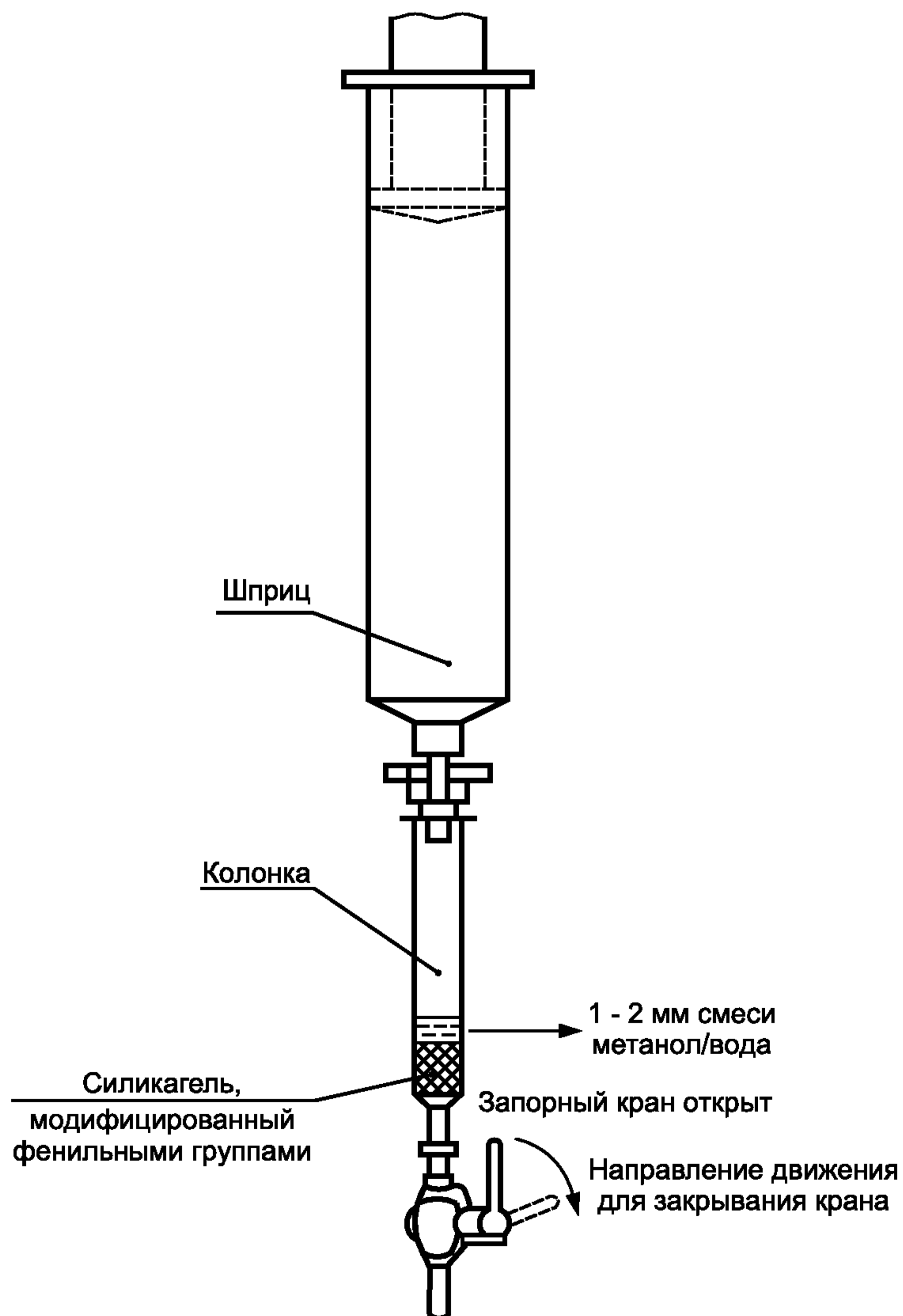
Рисунок 1 — Подготовка очистительной колонки
