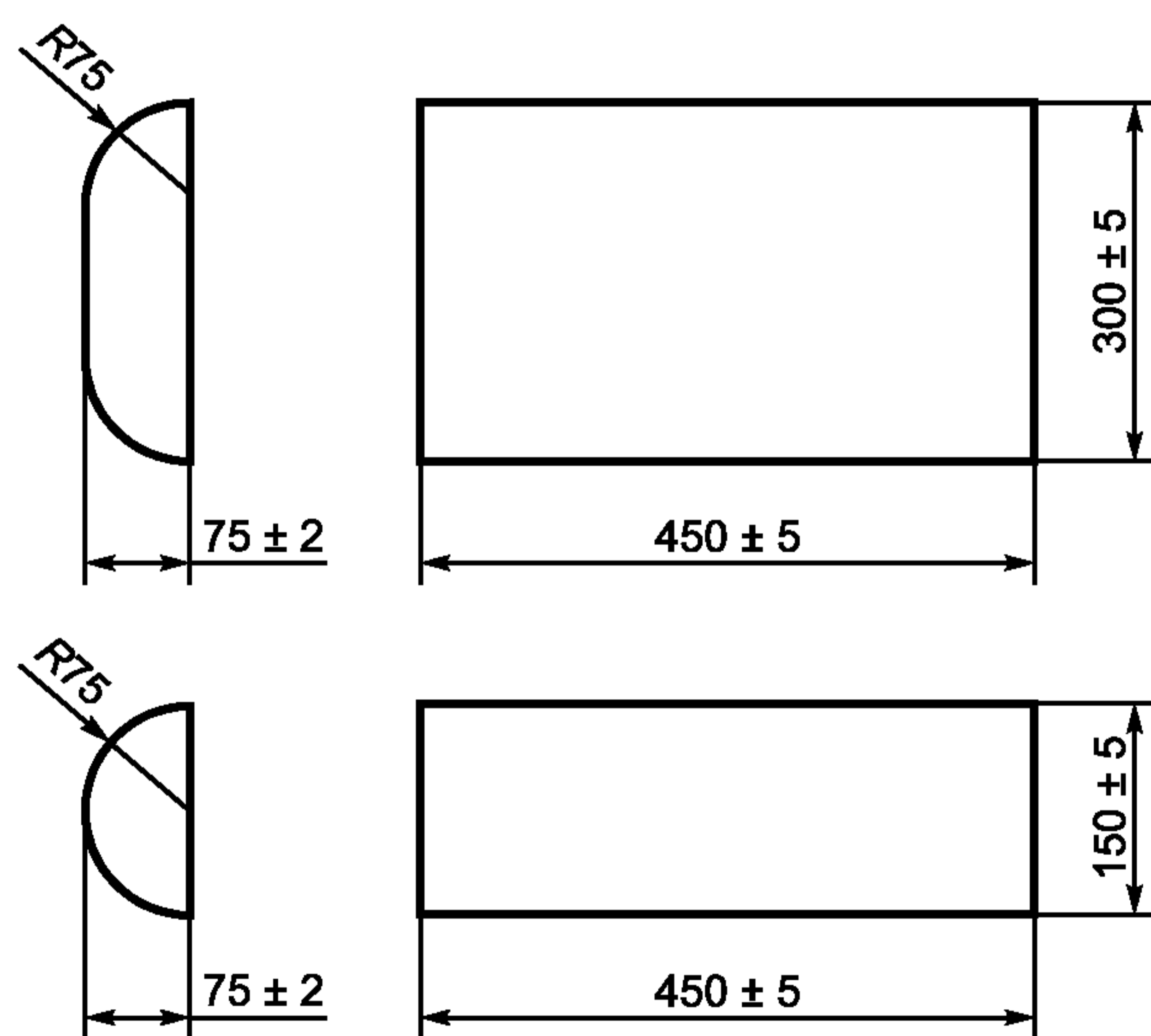
Рисунок 1 — Размеры образца
