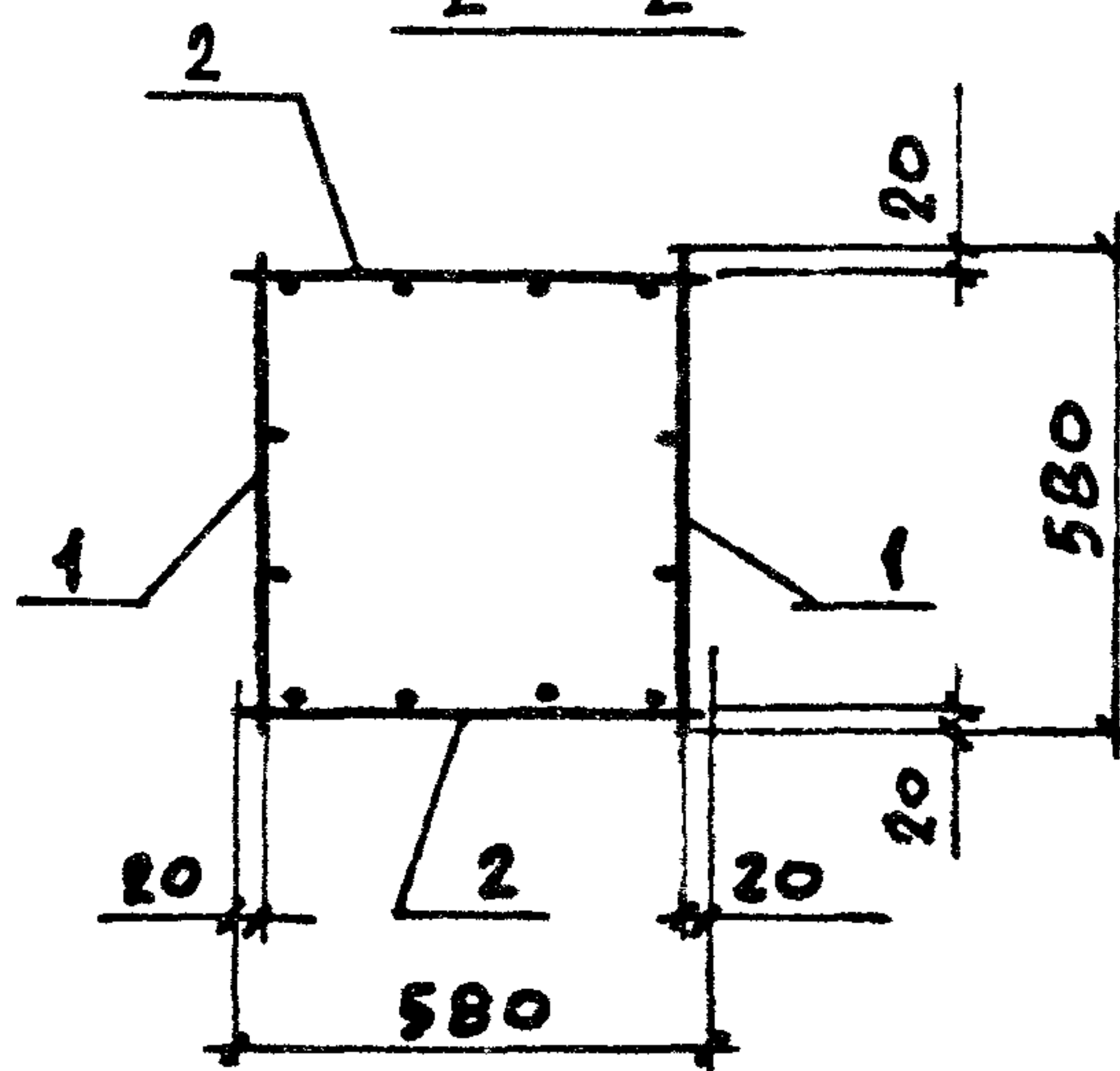
2 - 2
