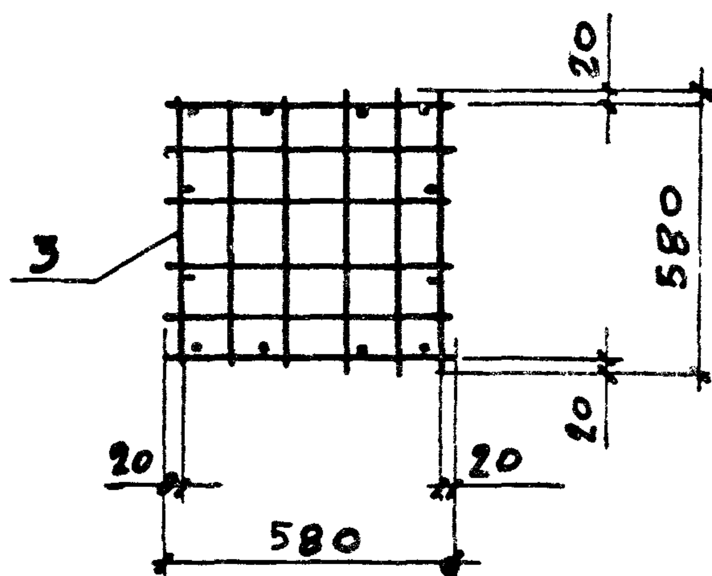
1 - 1
