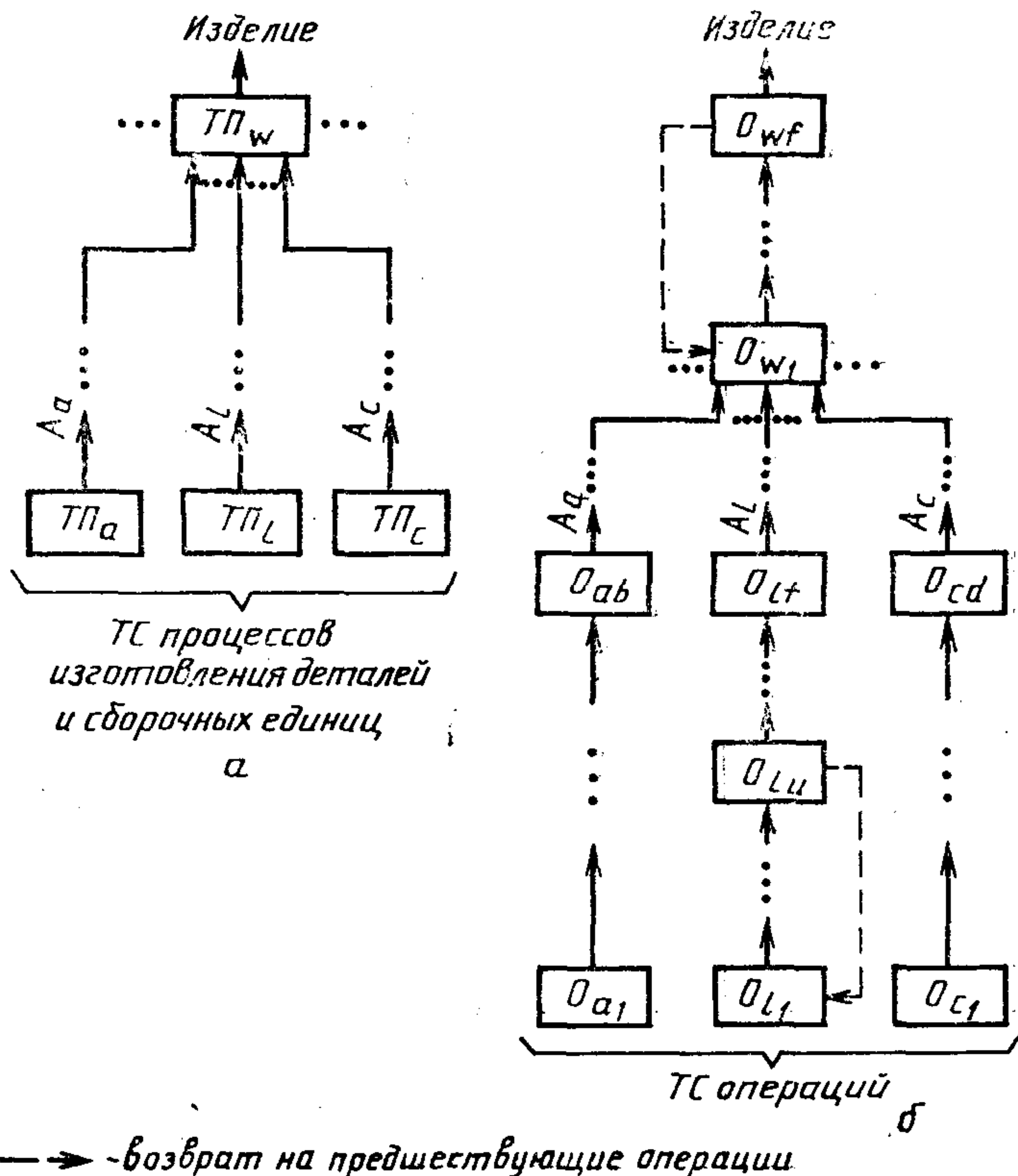
Черт. 1. Структурная схема ТС процесса изготовления изделия:
