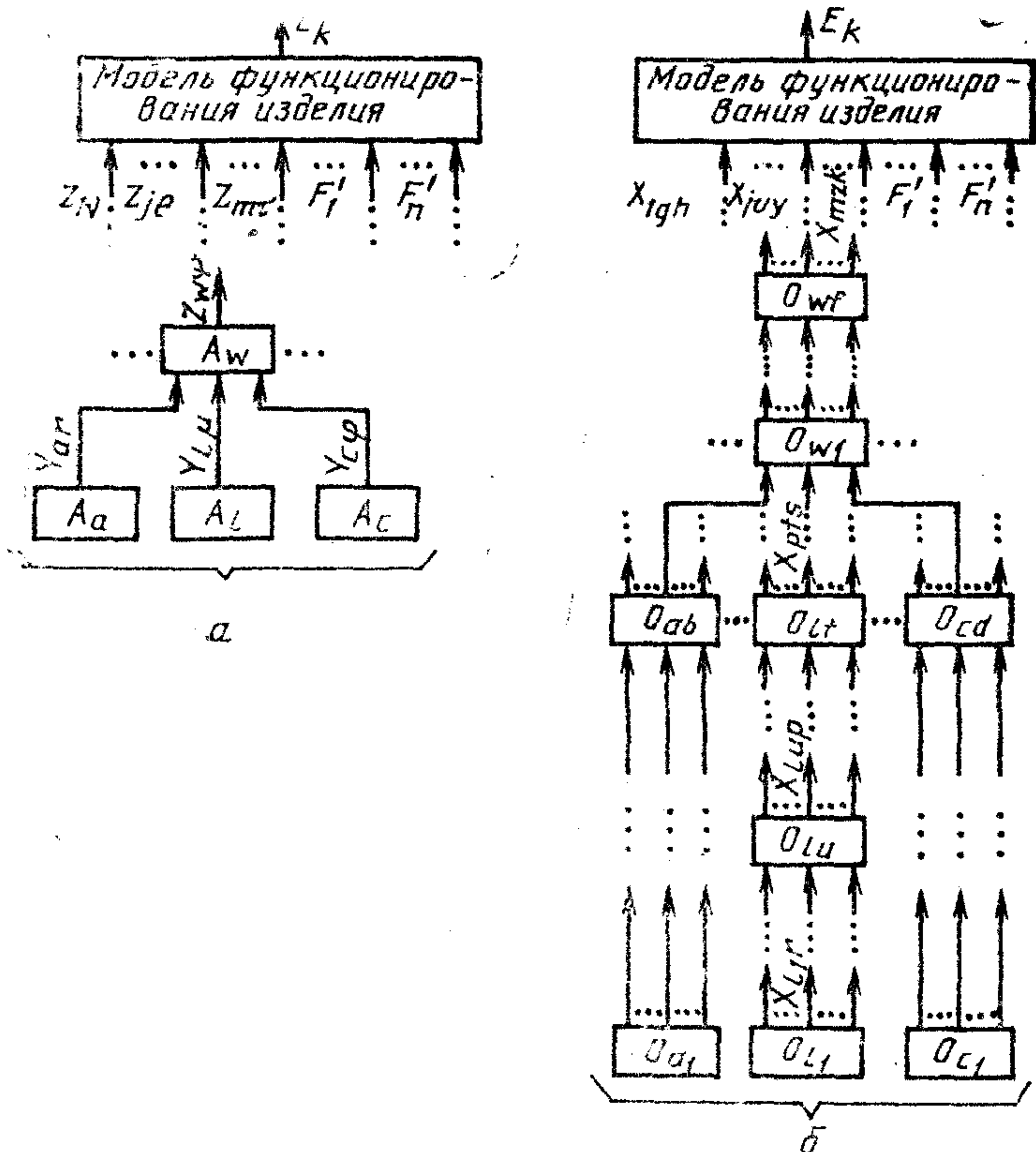
Черт. 3. Схема формирования k -го эксплуатационного параметра: а—на уровне деталей и сборочных единиц; б—на уровне операций; F'_1 \dots F'_n —функциональные параметры, не зависящие от выполнения ТП; A_l — l -я деталь; Y_{l\mu} — \mu -й параметр l -й детали; Z_{\psi\phi} — \psi -й параметр \omega -й сборочной единицы; O_{lu} — u -я операция обработки l -й детали ( l= =1 \dots t ); X_{lpr} — r -й параметр u -й операции обработки l -й детали
