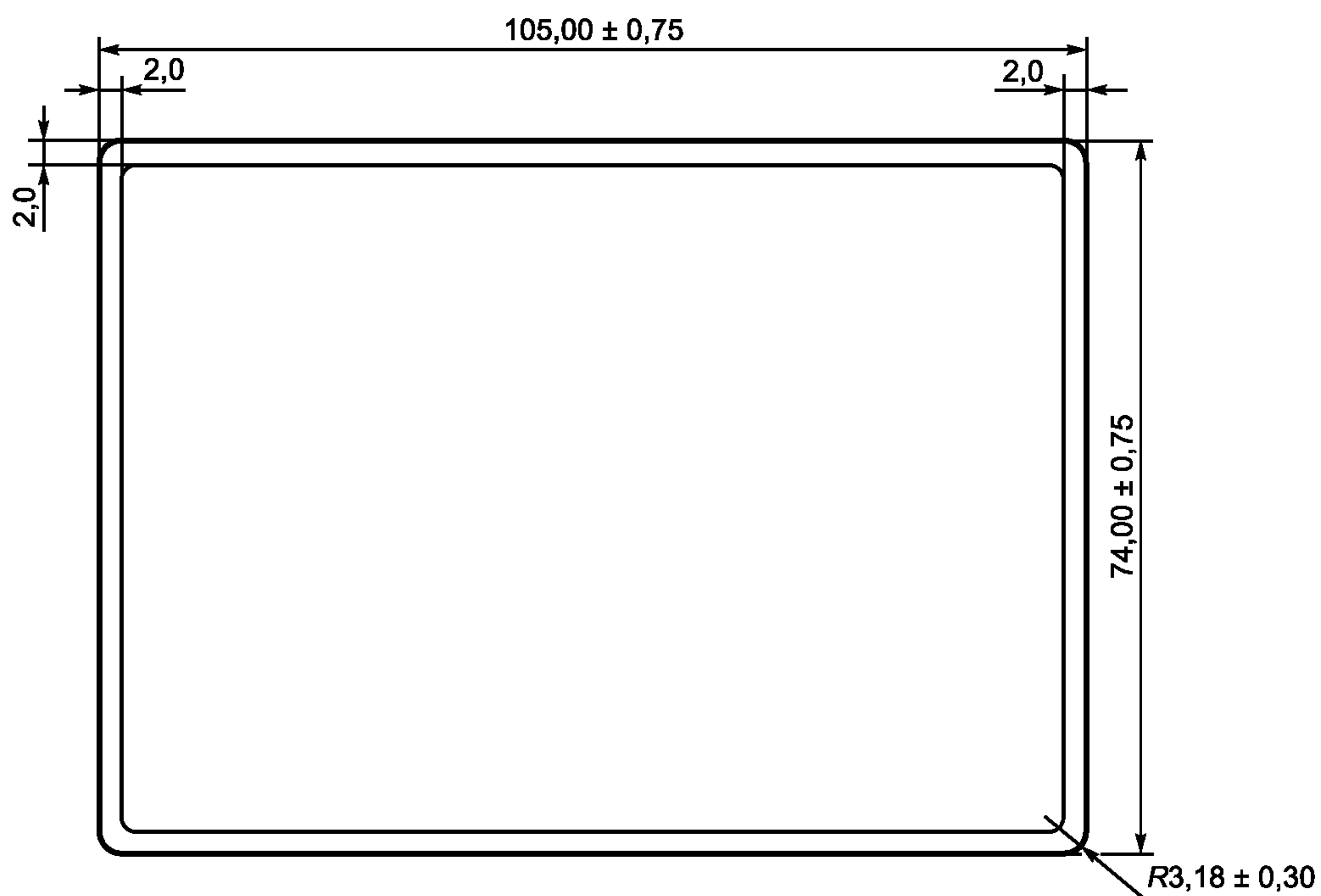
Рисунок 5 — Размеры и допуски документа ПД-2
