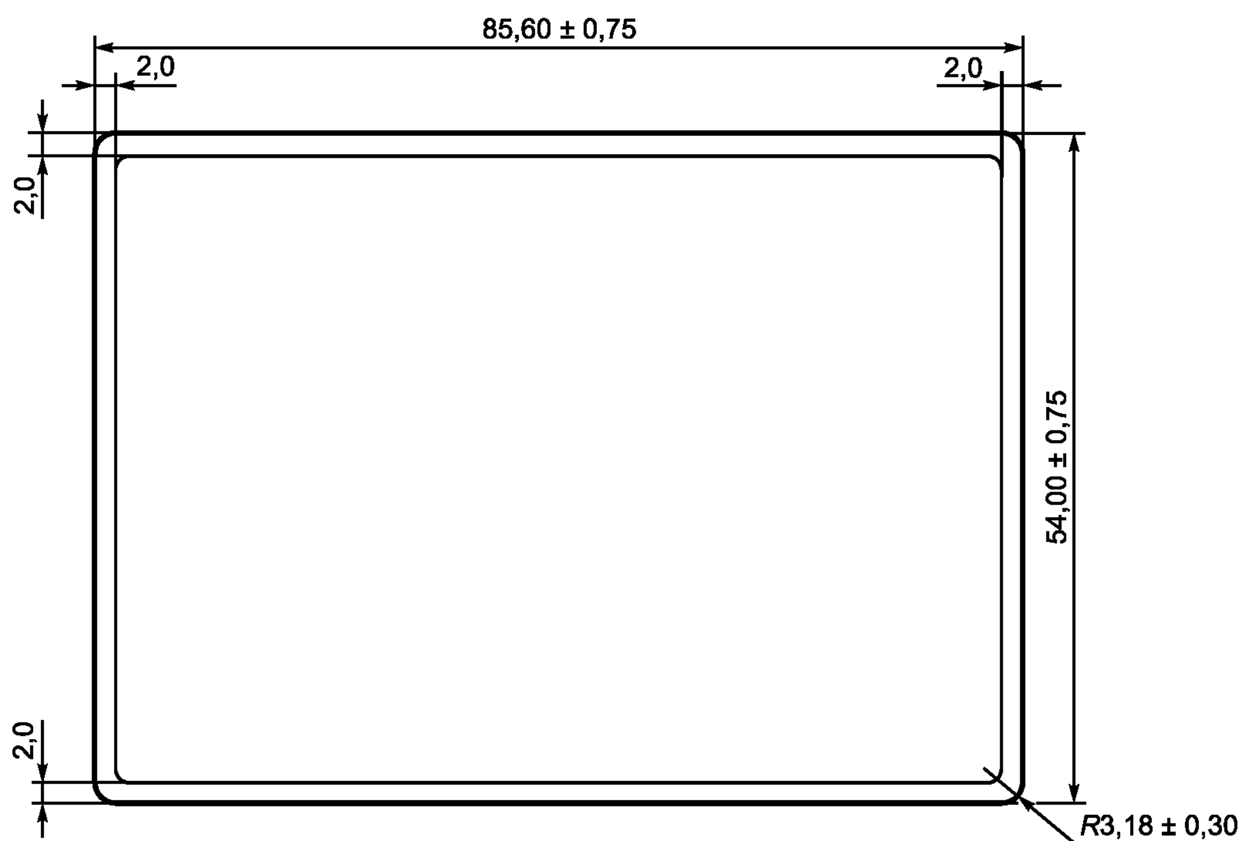
Рисунок 2 — Размеры и допуски документа ПД-1
