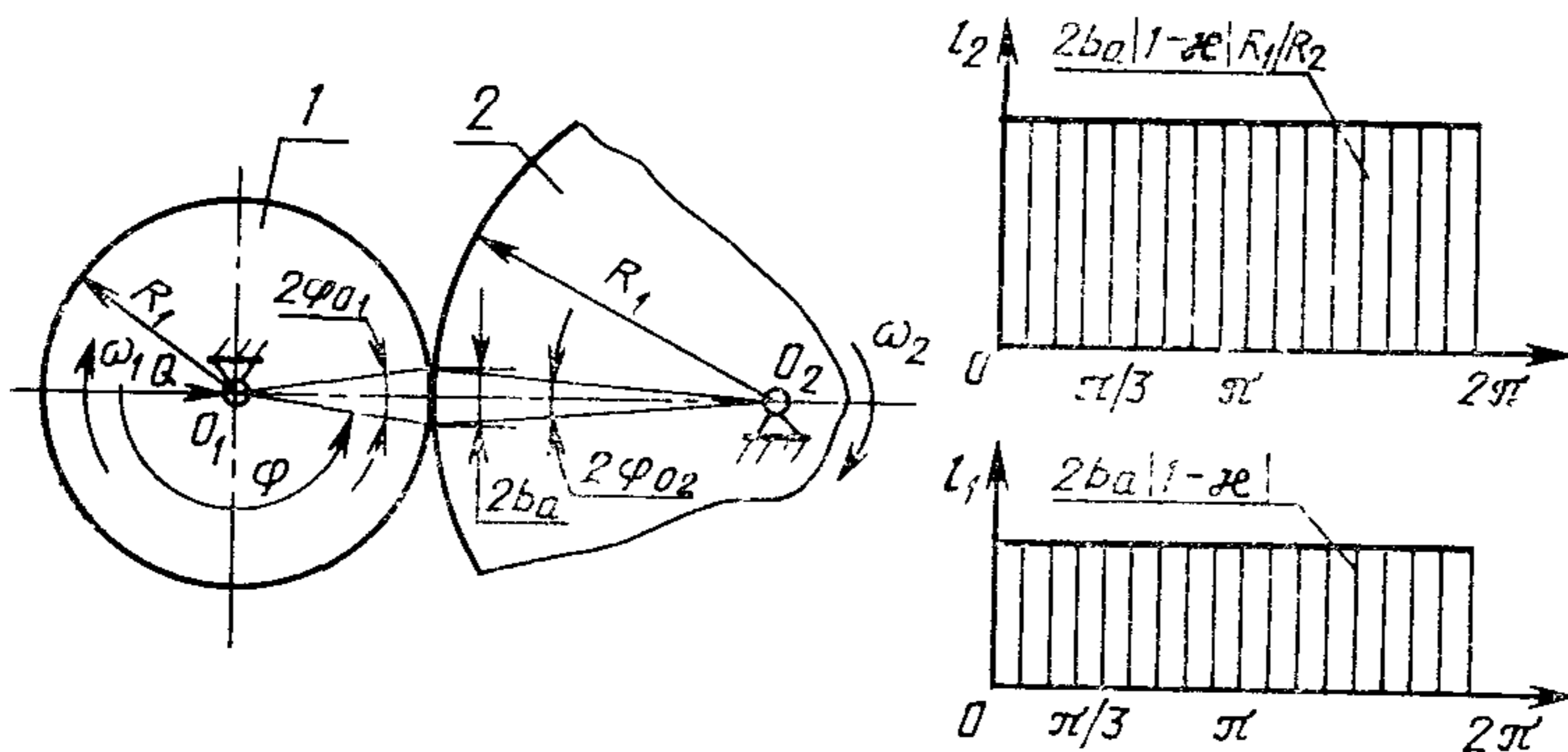
1—ведущий ролик (деталь 1); 2—ведомый ролик (деталь 2)
