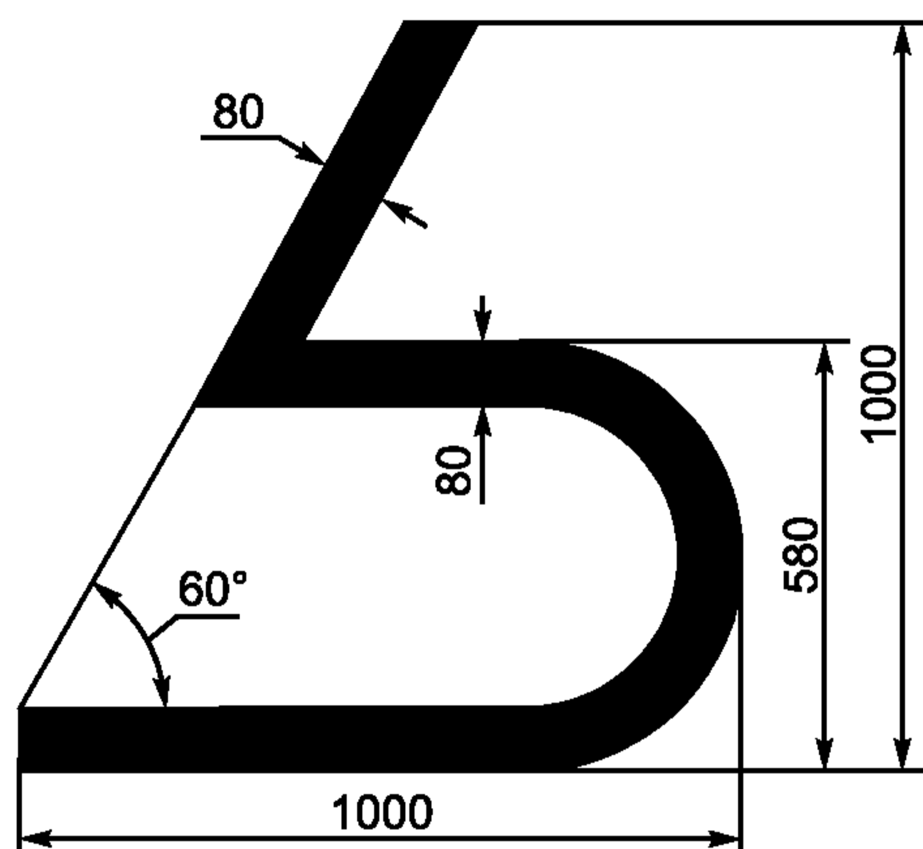
Рисунок 1 — Условное обозначение бульбообразного носа
