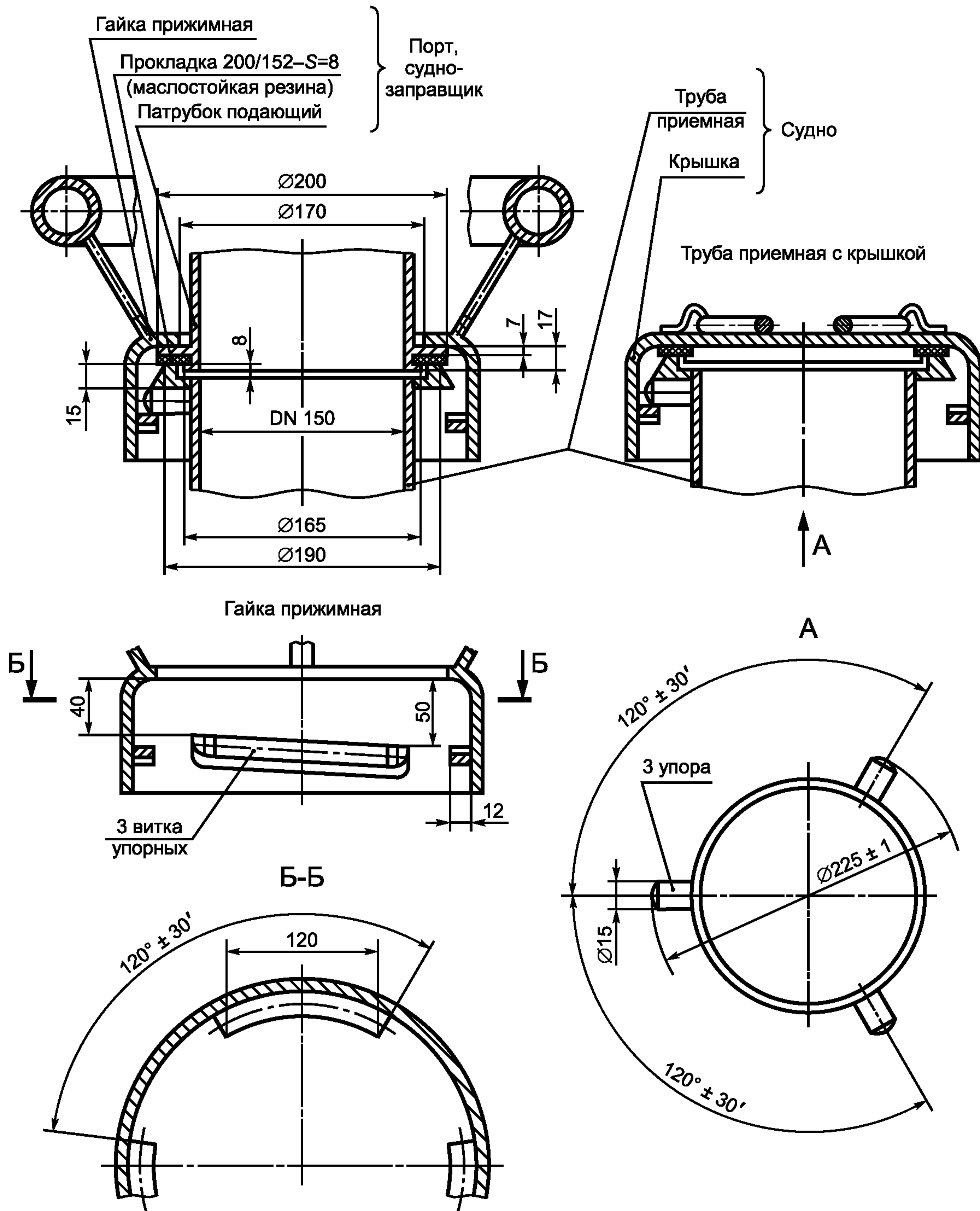
Рисунок 2 — Устройство для приема топлива номинальным диаметром 150 мм
