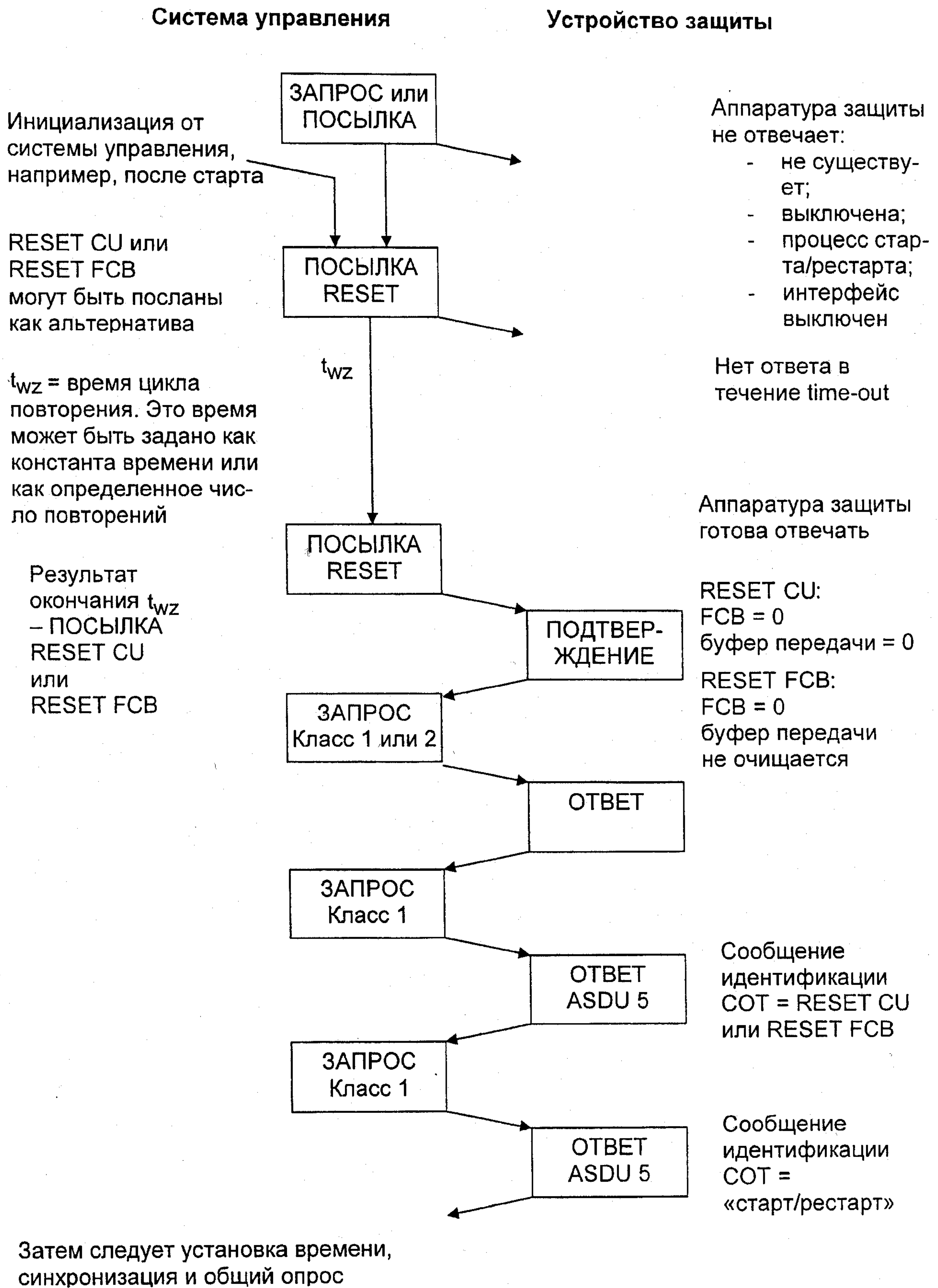
Рисунок 3 — Основная процедура инициализации
