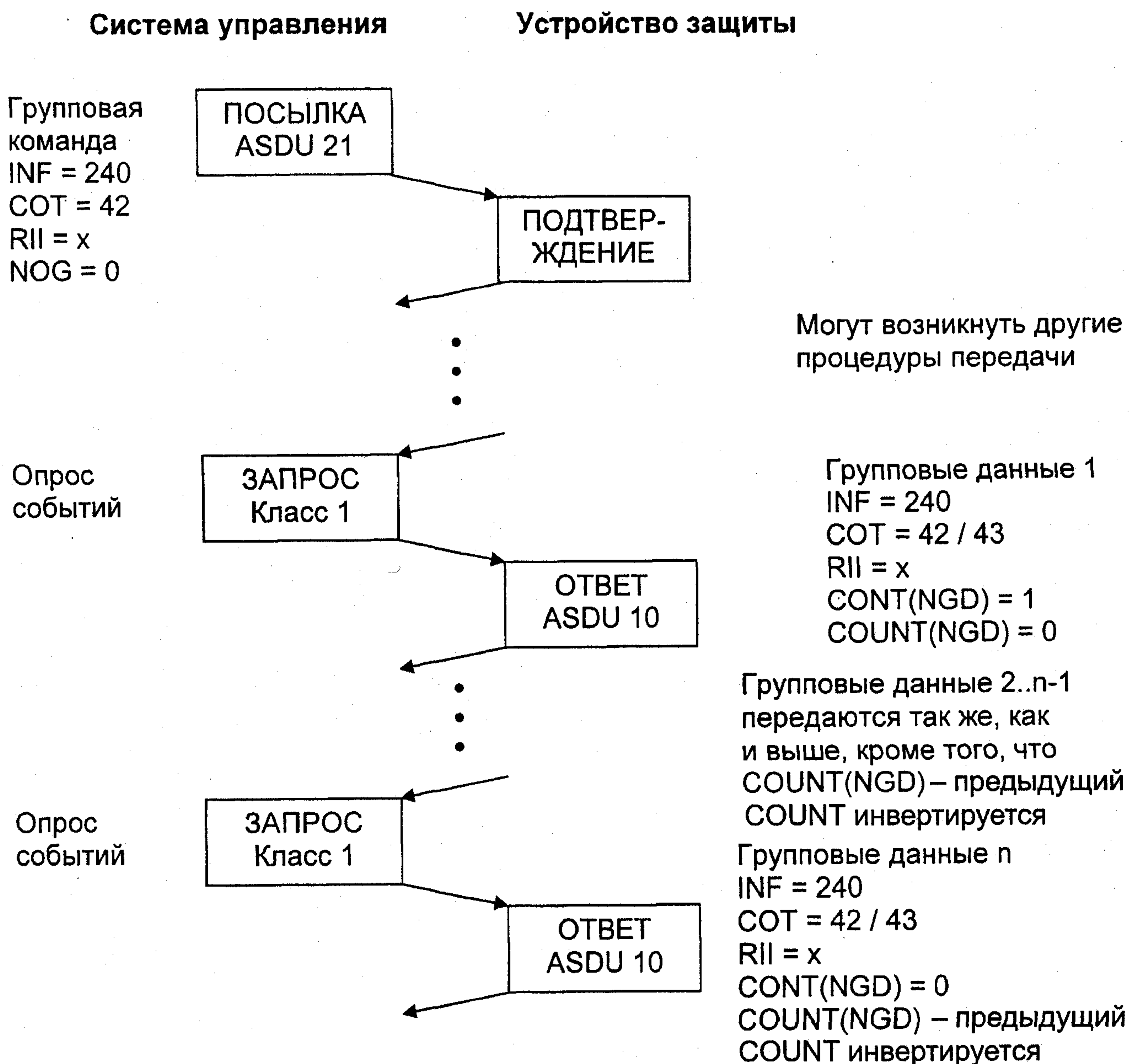
Рисунок 13 — Чтение заголовков всех определенных групп
