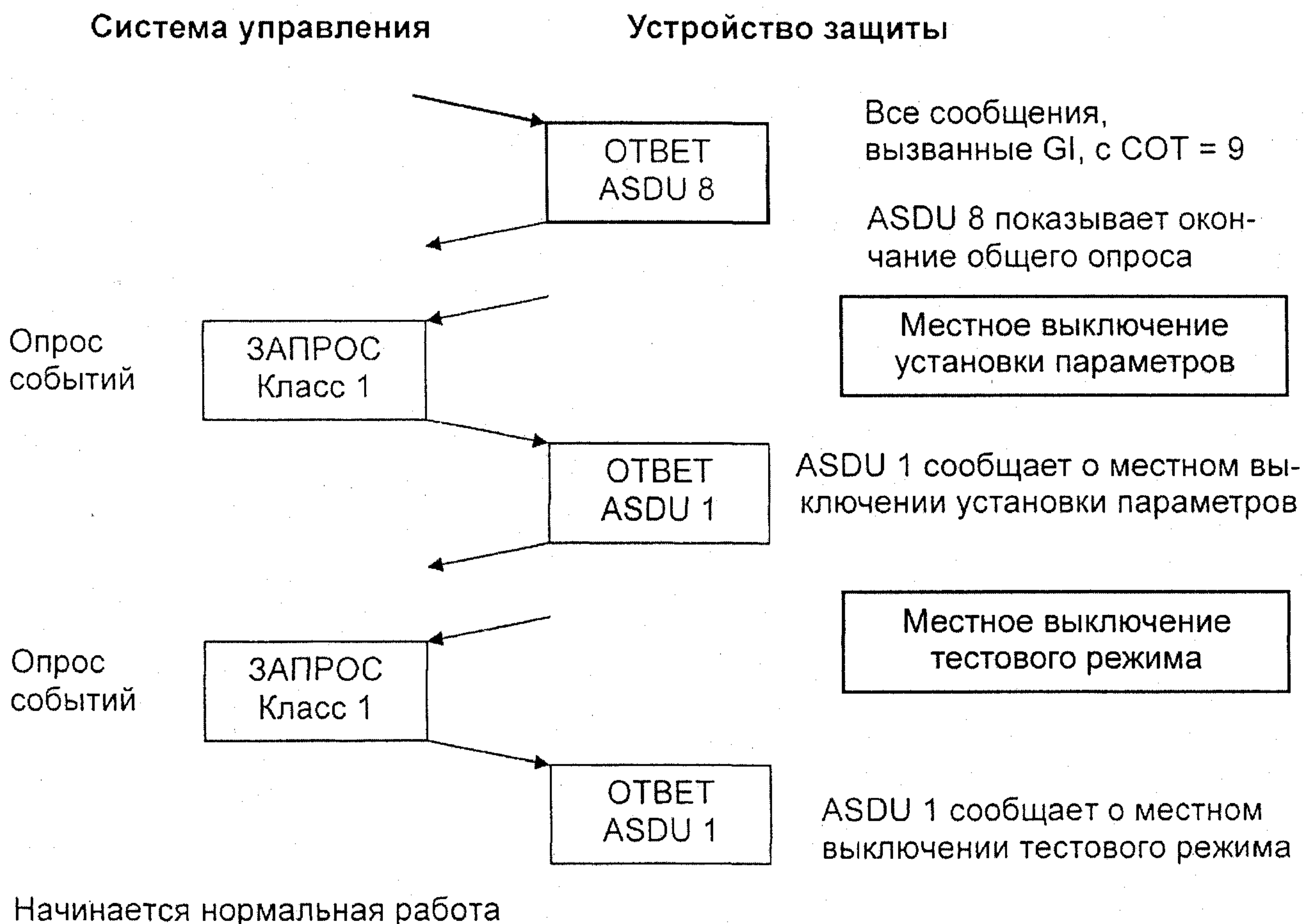
Рисунок 8 — Тестовый режим (лист 2)
