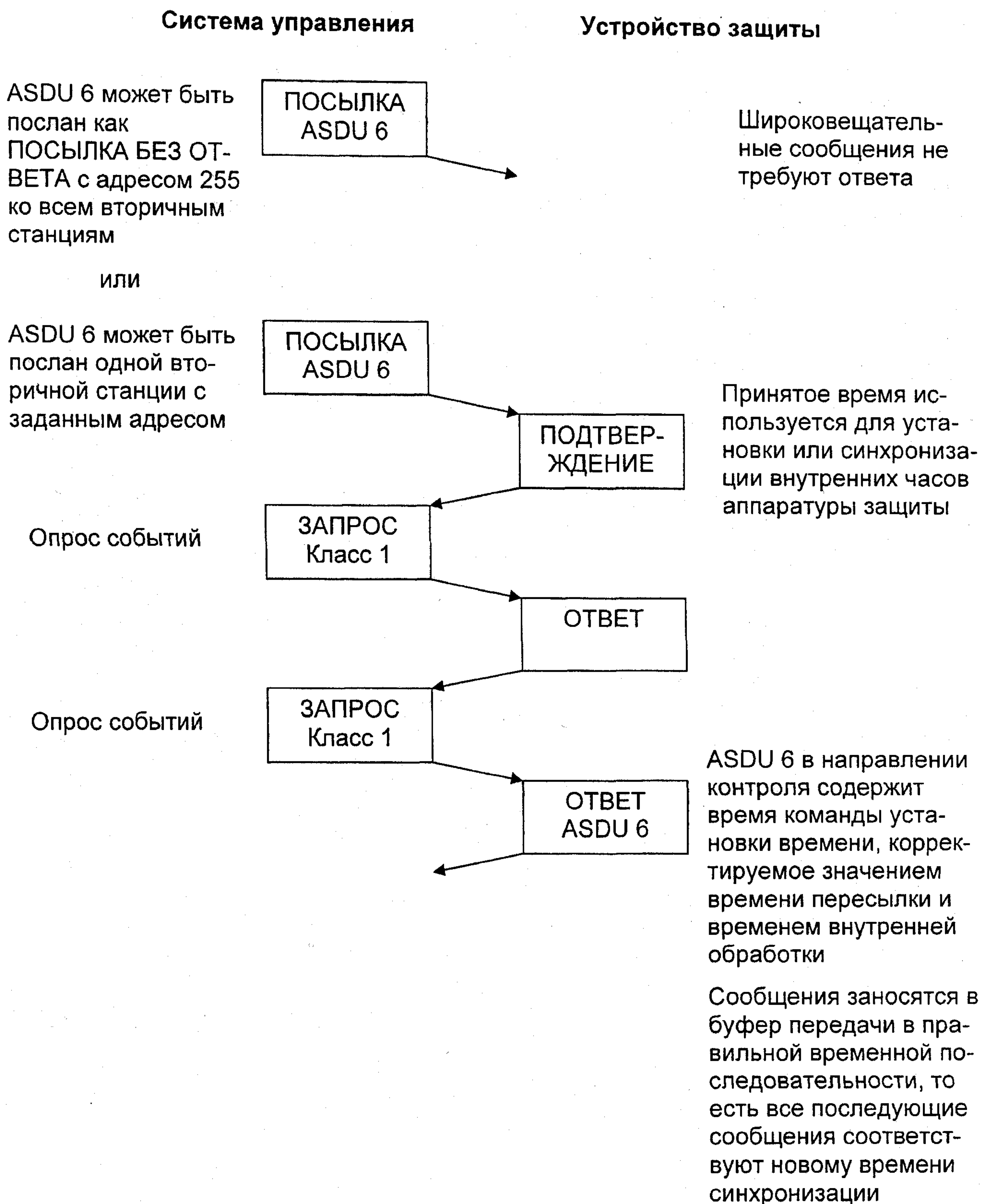
Рисунок 5 — Синхронизация времени
