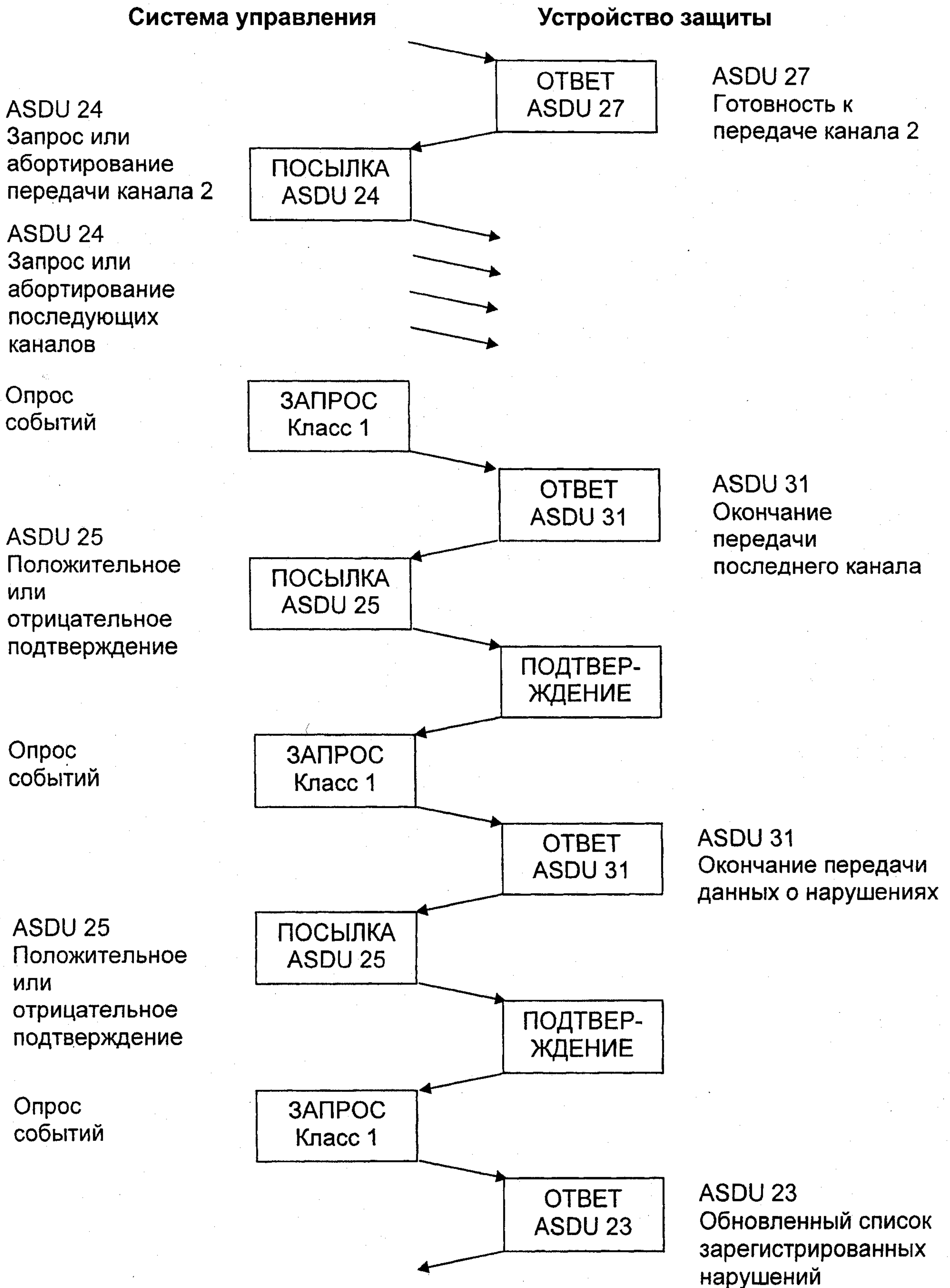
Рисунок 10 — Передача данных о нарушениях (лист 4)
