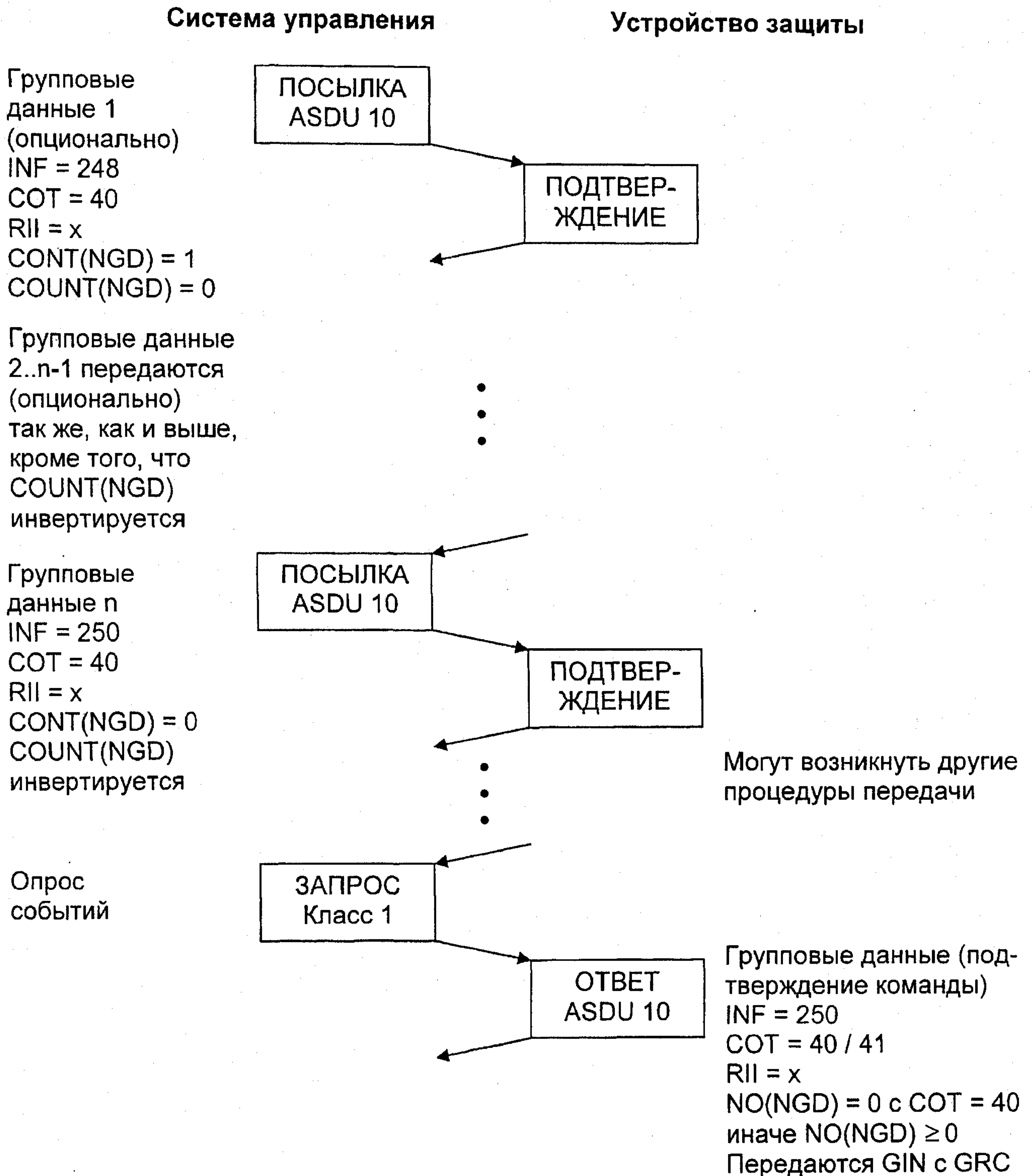
Рисунок 17 — Запись значений одиночных элементов
