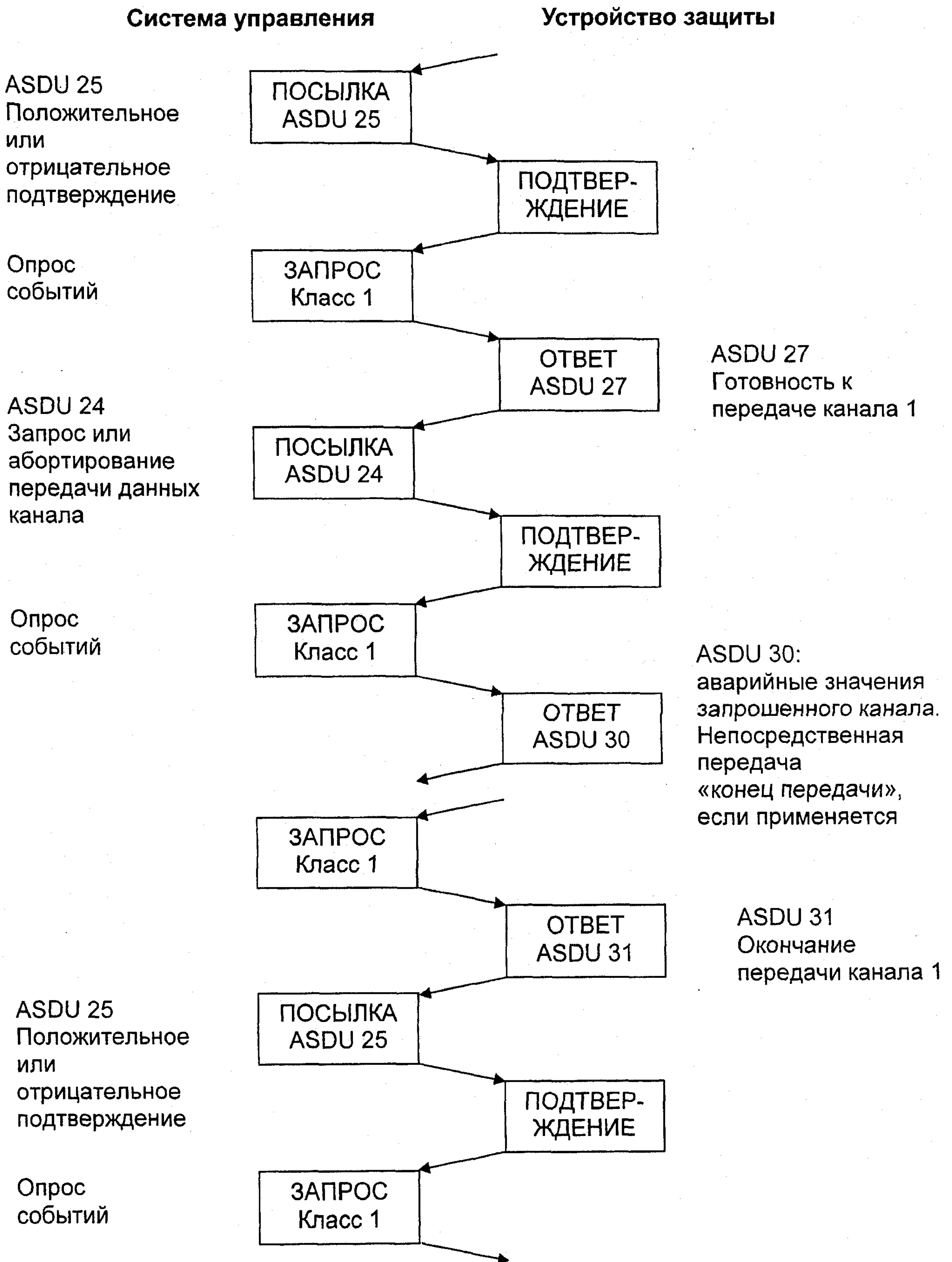
Рисунок 10 — Передача данных о нарушениях (лист 3)
