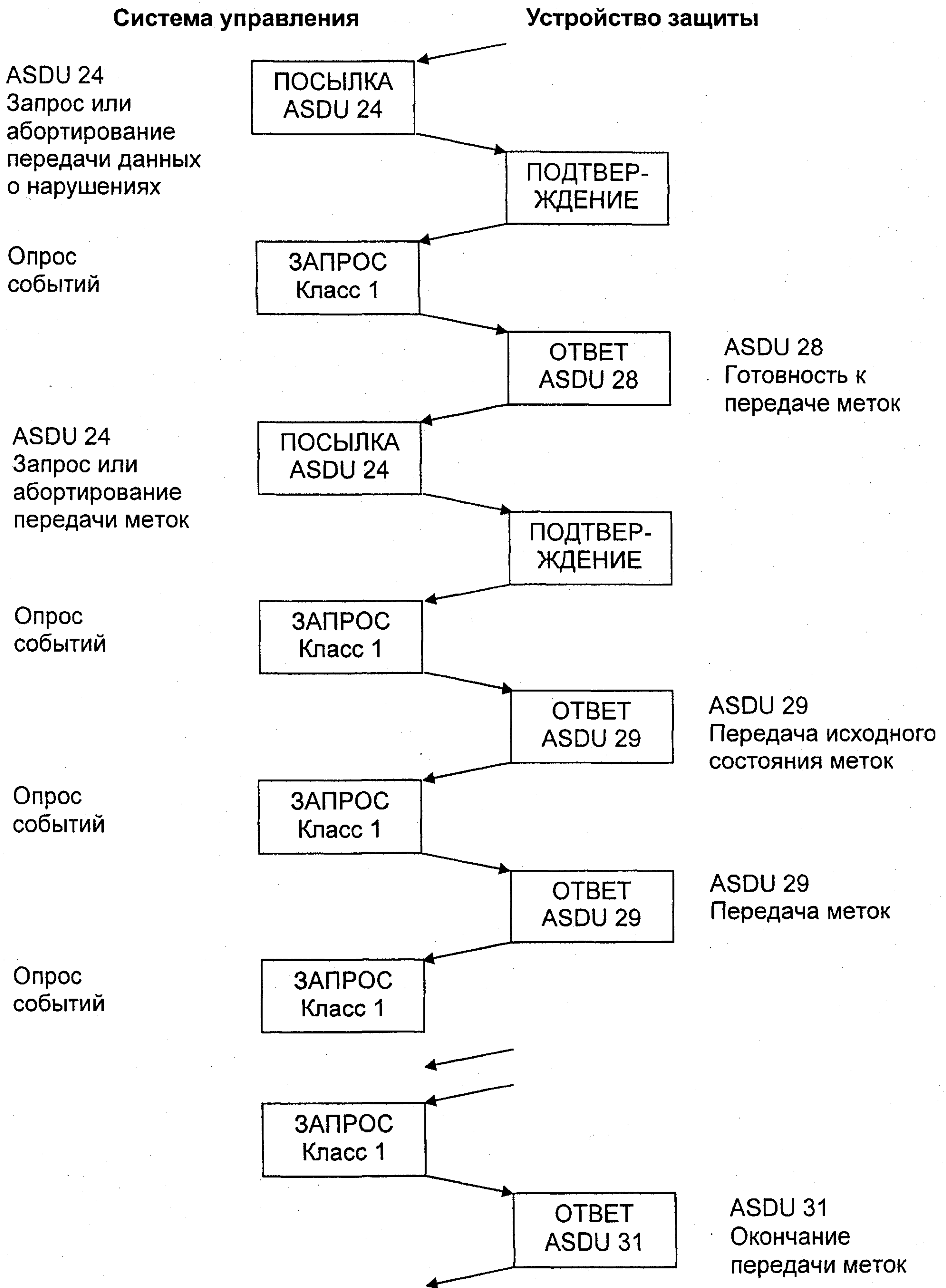
Рисунок 10 — Передача данных о нарушениях (лист 2)
