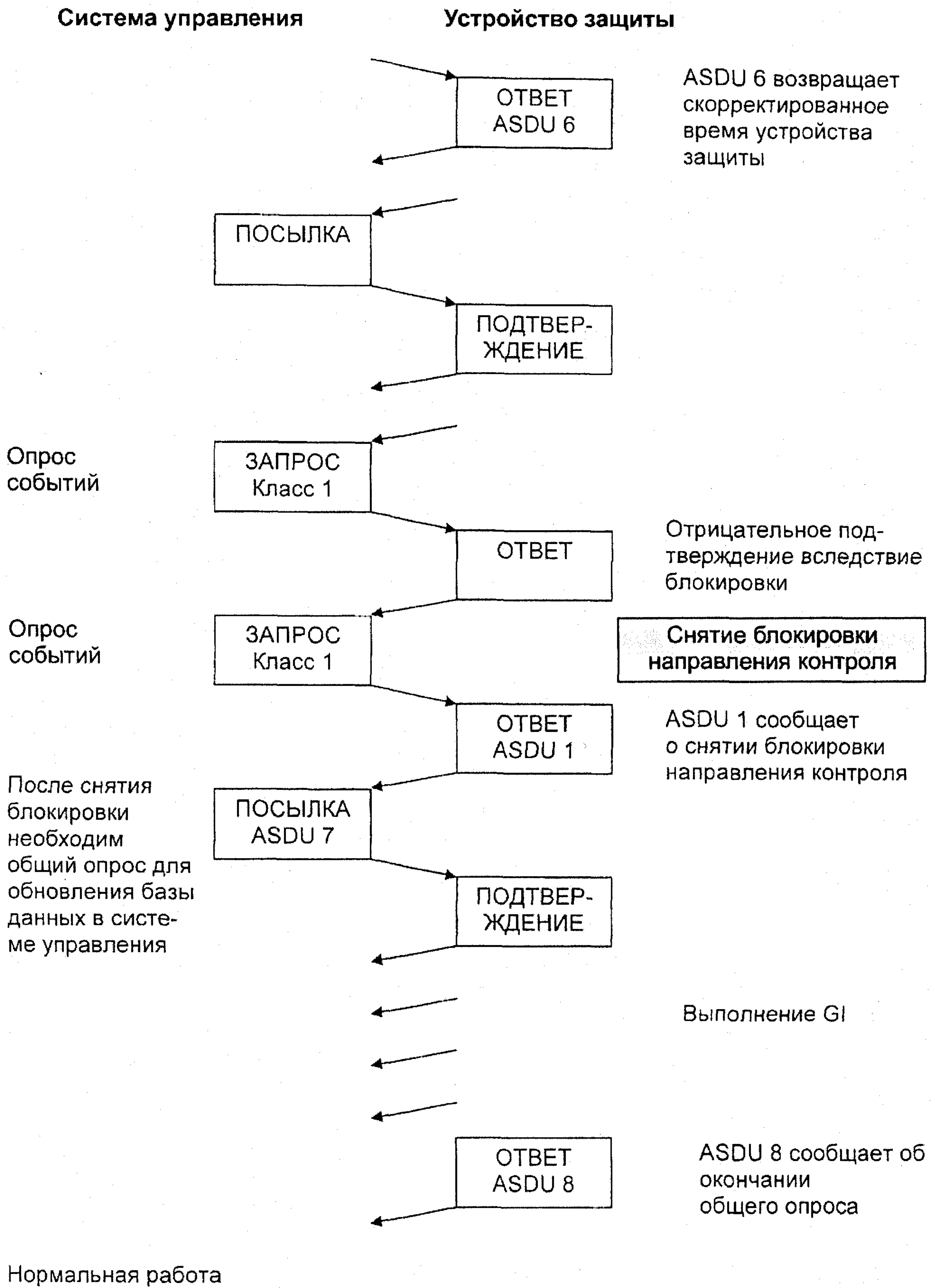
Рисунок 9 — Блокировка направления контроля (лист 2)
