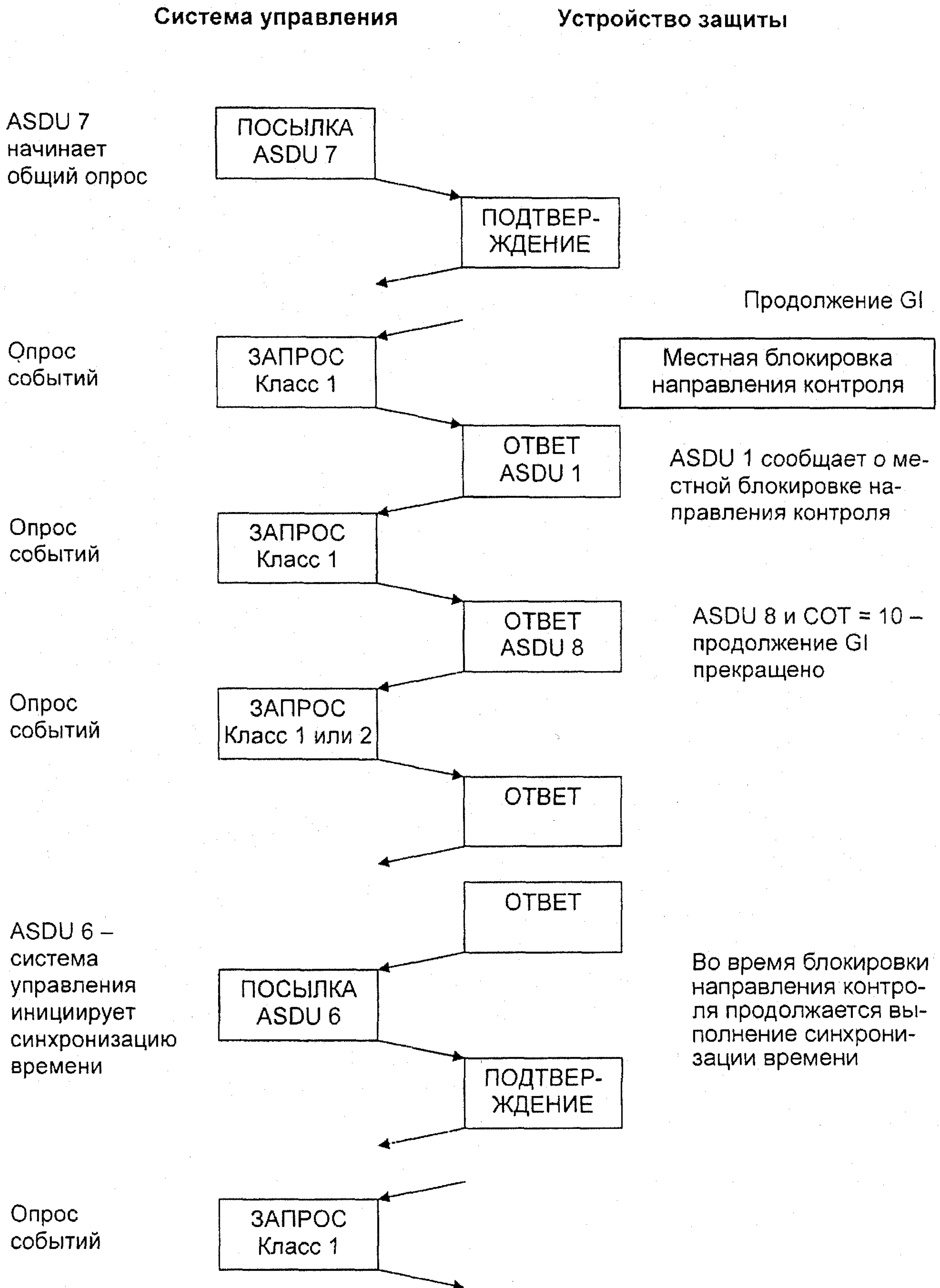
Рисунок 9 — Блокировка направления контроля (лист 1)
