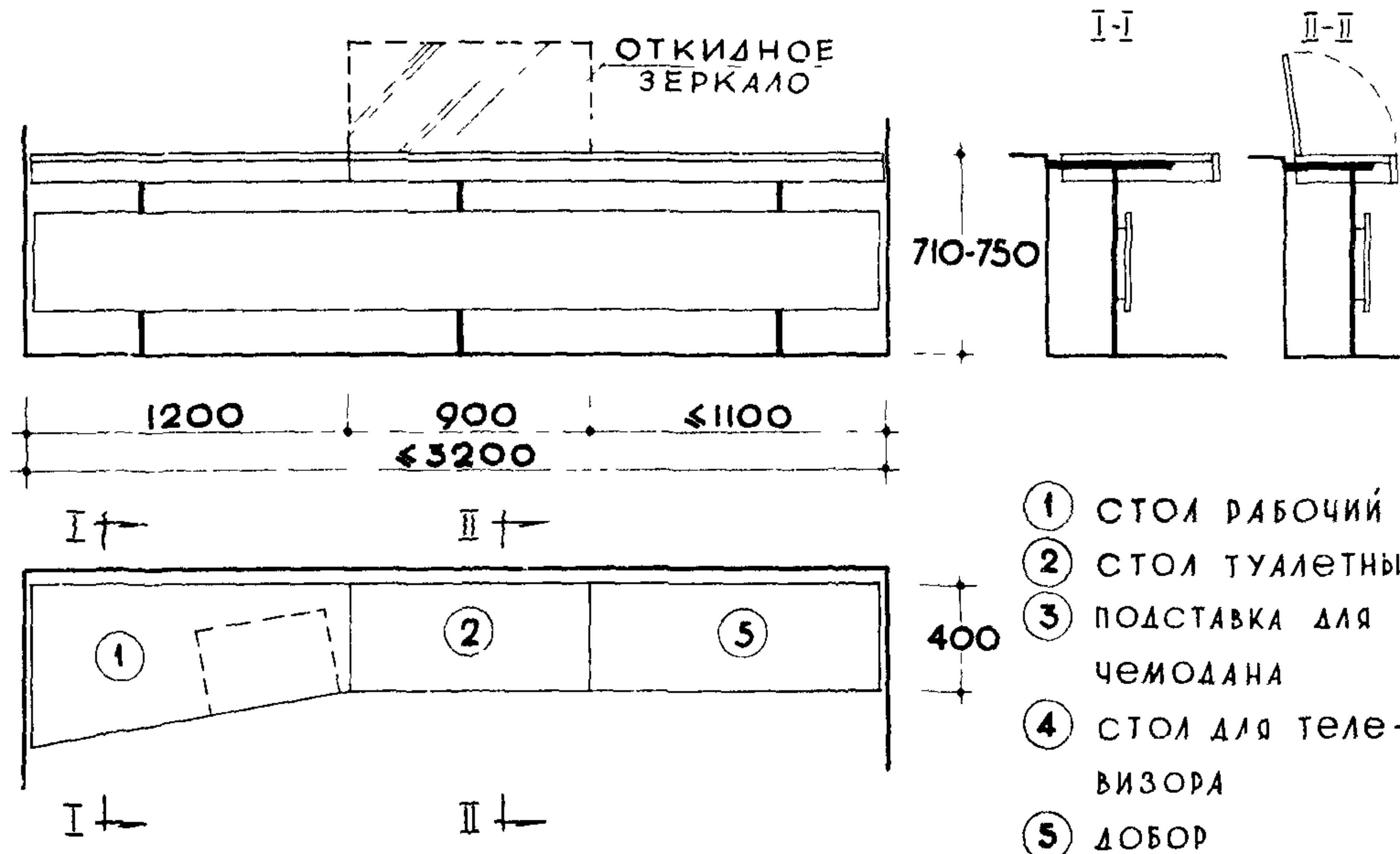
СТОЛ КОМБИНИРОВАННЫЙ /ПОДОКОННЫЙ/
