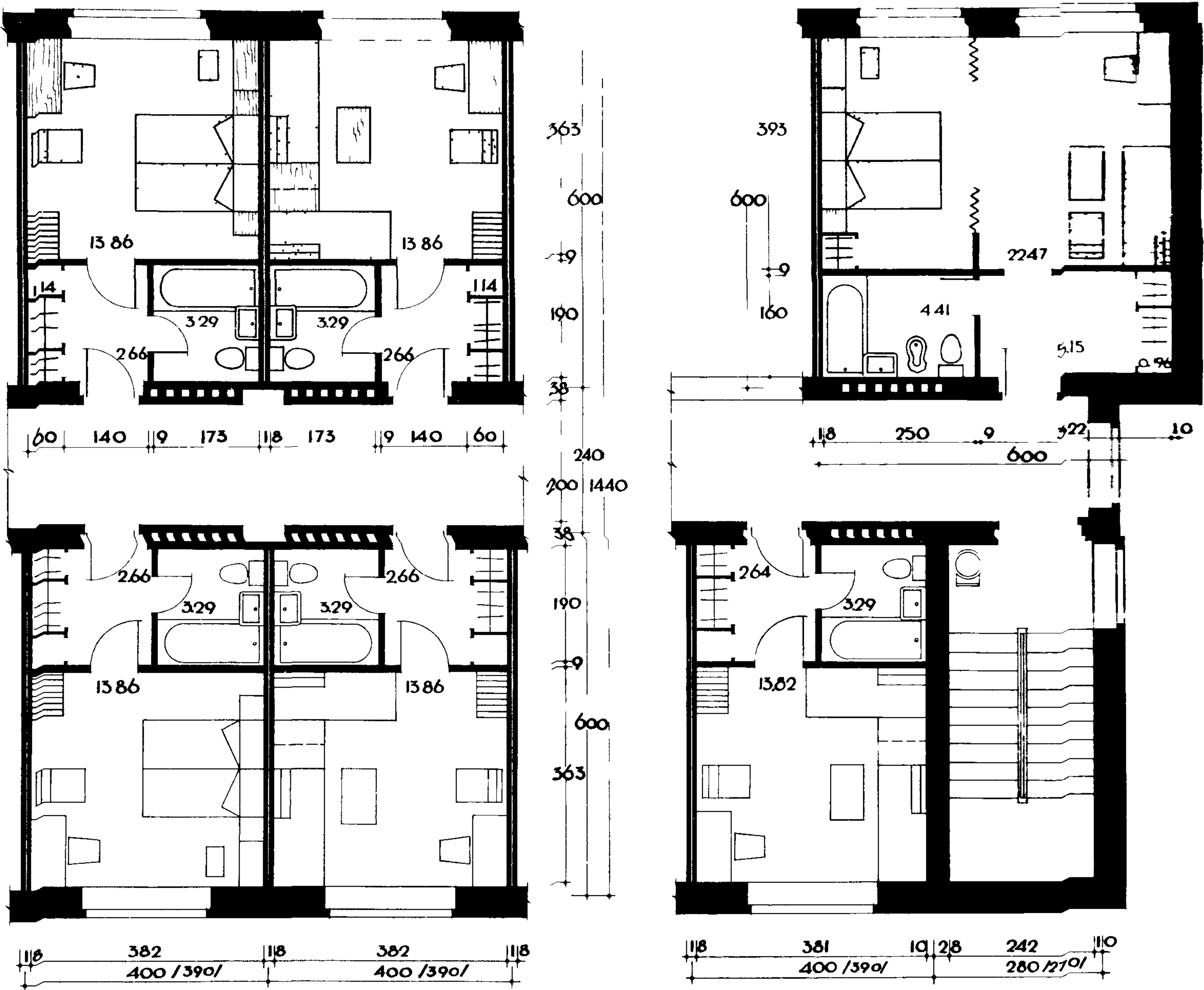
ПРОДОЛЬНЫЕ НЕСУЩИЕ СТЕНЫ
