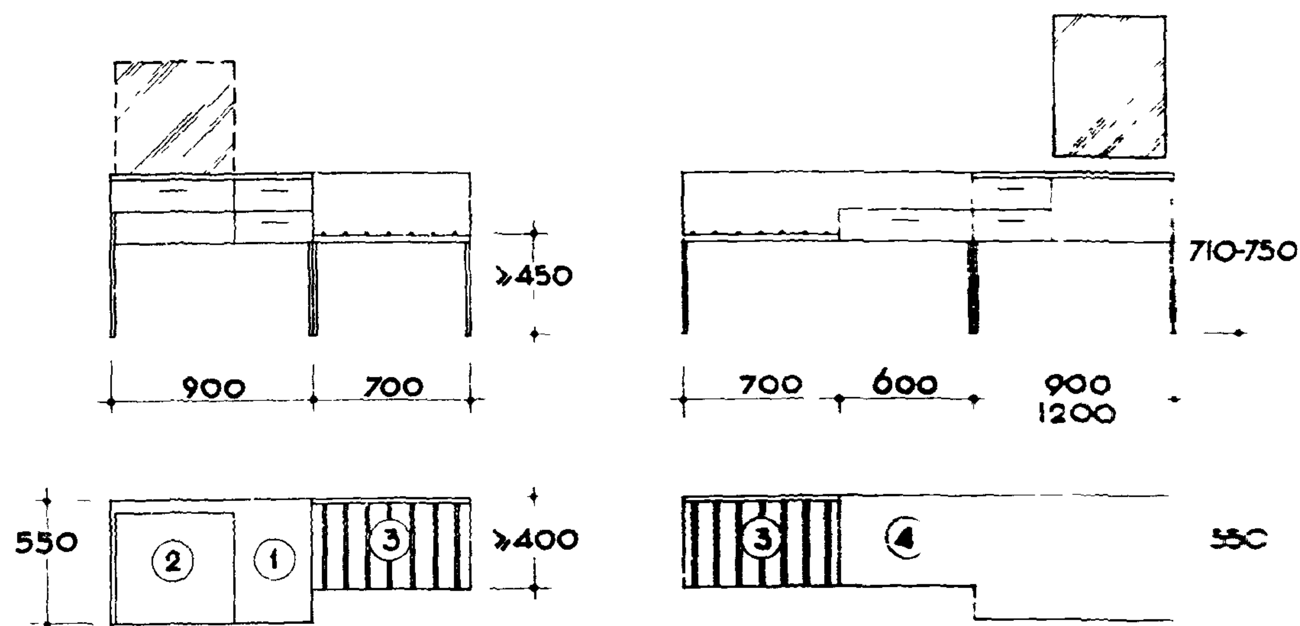
СТОЛ КОМБИНИРОВАННЫЙ /ПОДОКОННЫЙ/
