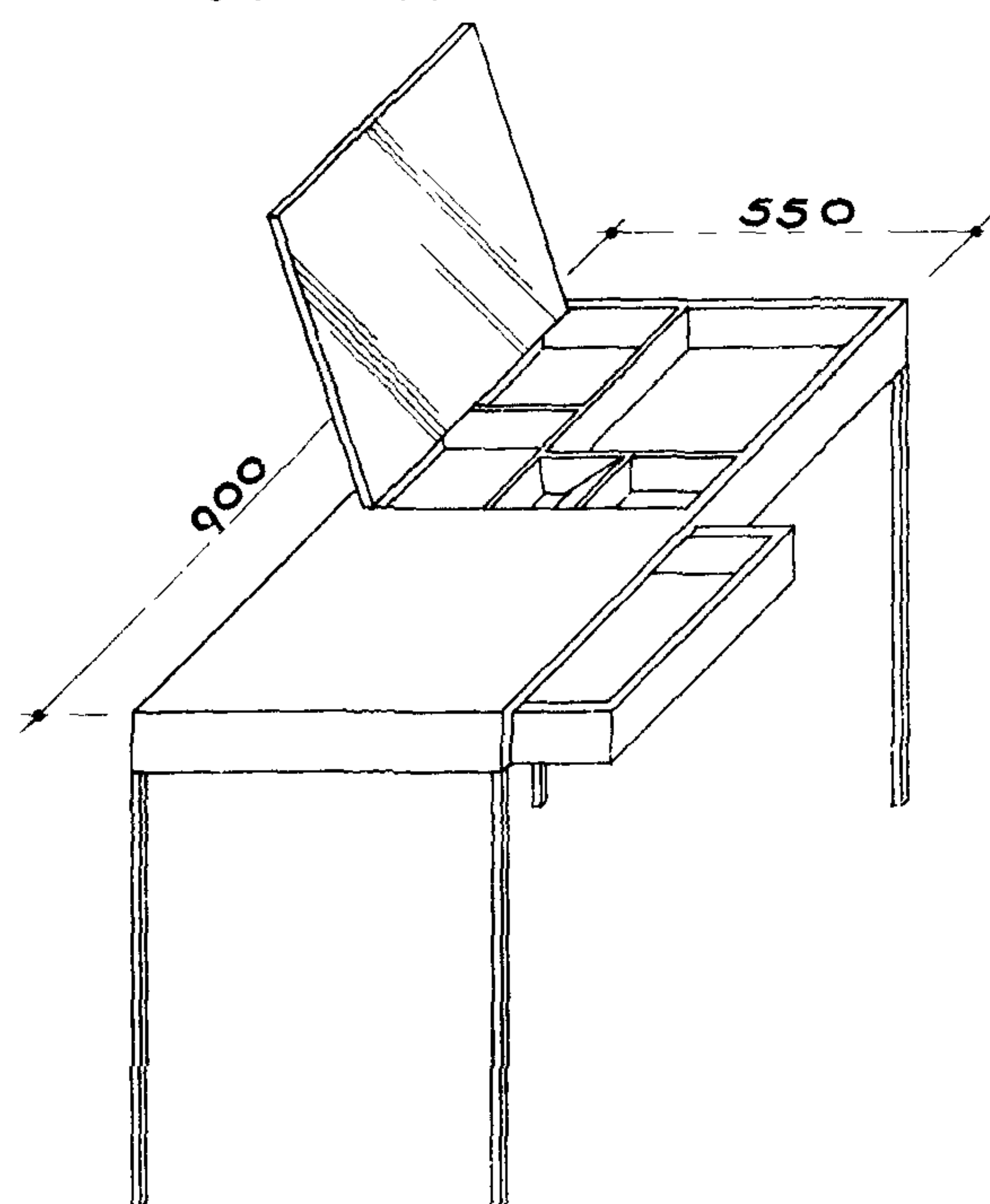
СТОЛ РАБОЧИЙ И ТУАЛЕТНЫЙ С ОТКИДНЫМ ЗЕРКАЛОМ
