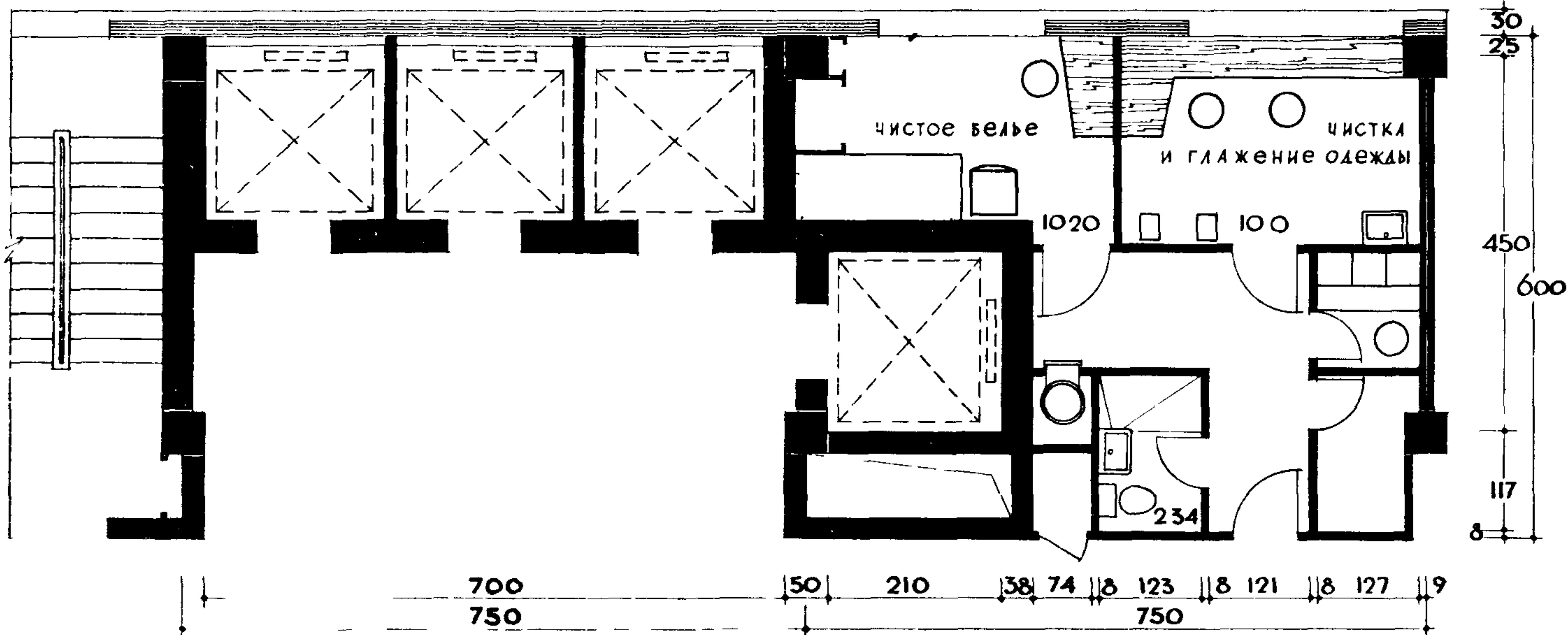
СБОРНЫЙ КАРКАС С ШАГОМ 750 см - для экспериментального строительства
