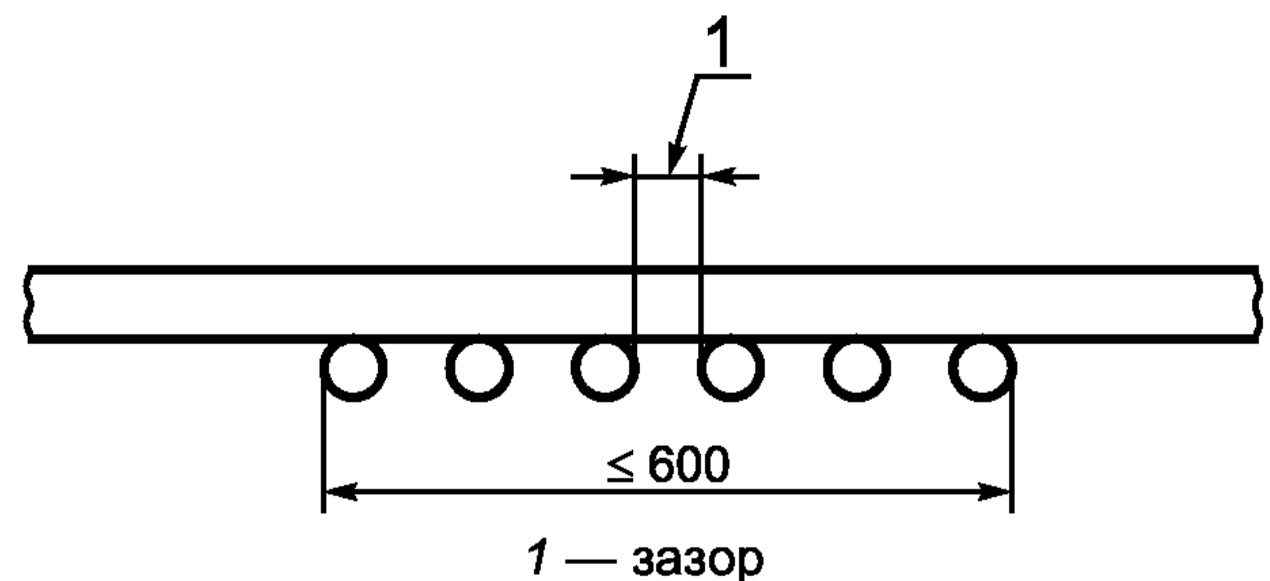
Рисунок 2 — Кабели, закрепленные на передней стороне широкой лестницы с зазором
