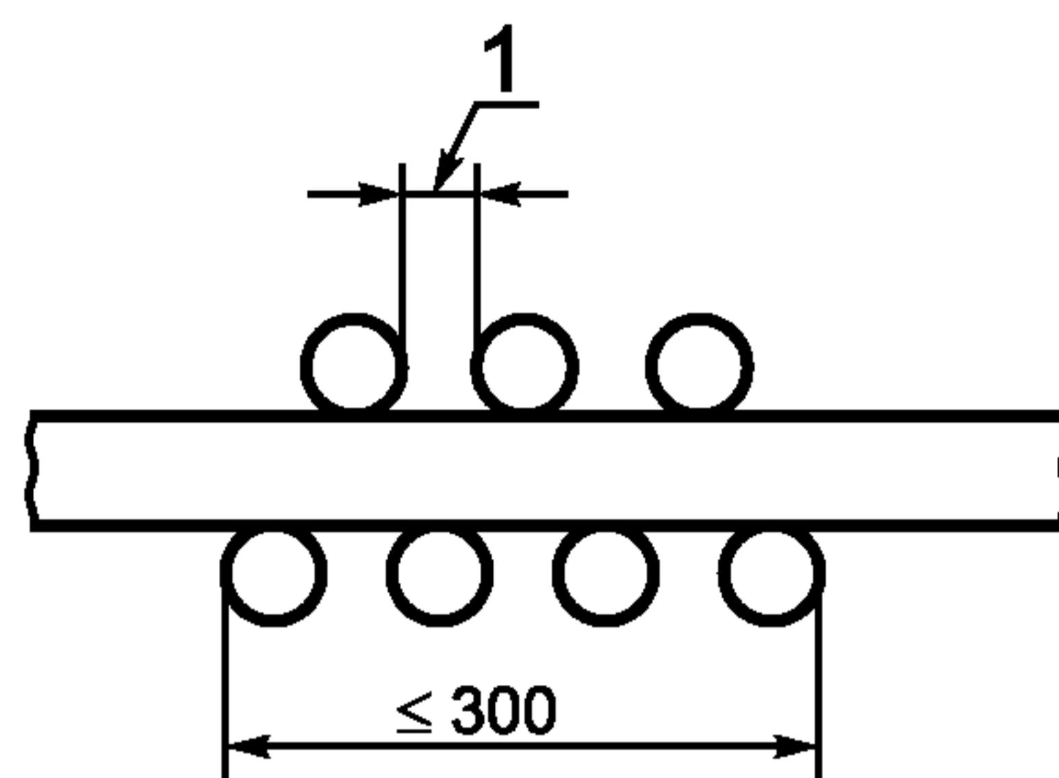
Рисунок 1 — Типичное расположение с зазором кабелей, закрепленных на обеих сторонах стандартной лестницы (категория А F/R)
