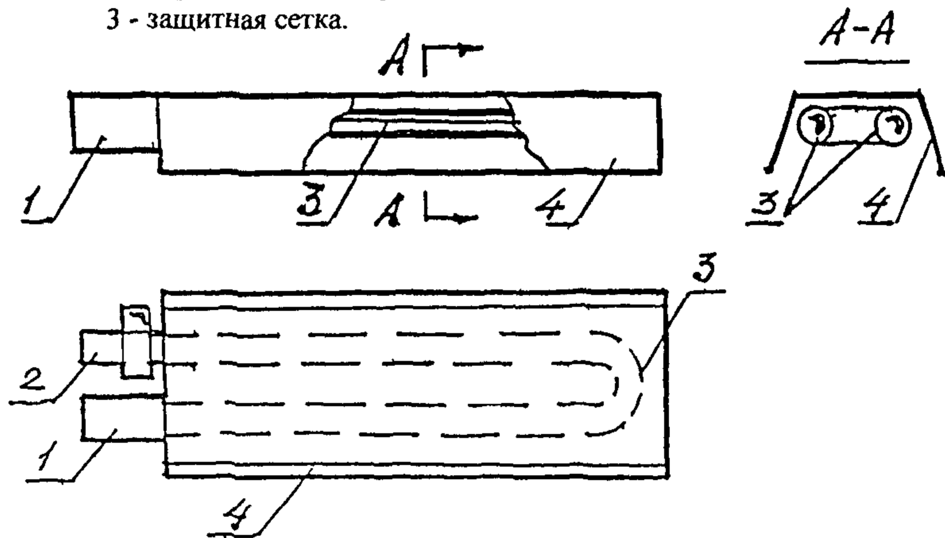
Рис. 1б. Схема "темного" газового инфракрасного излучателя
