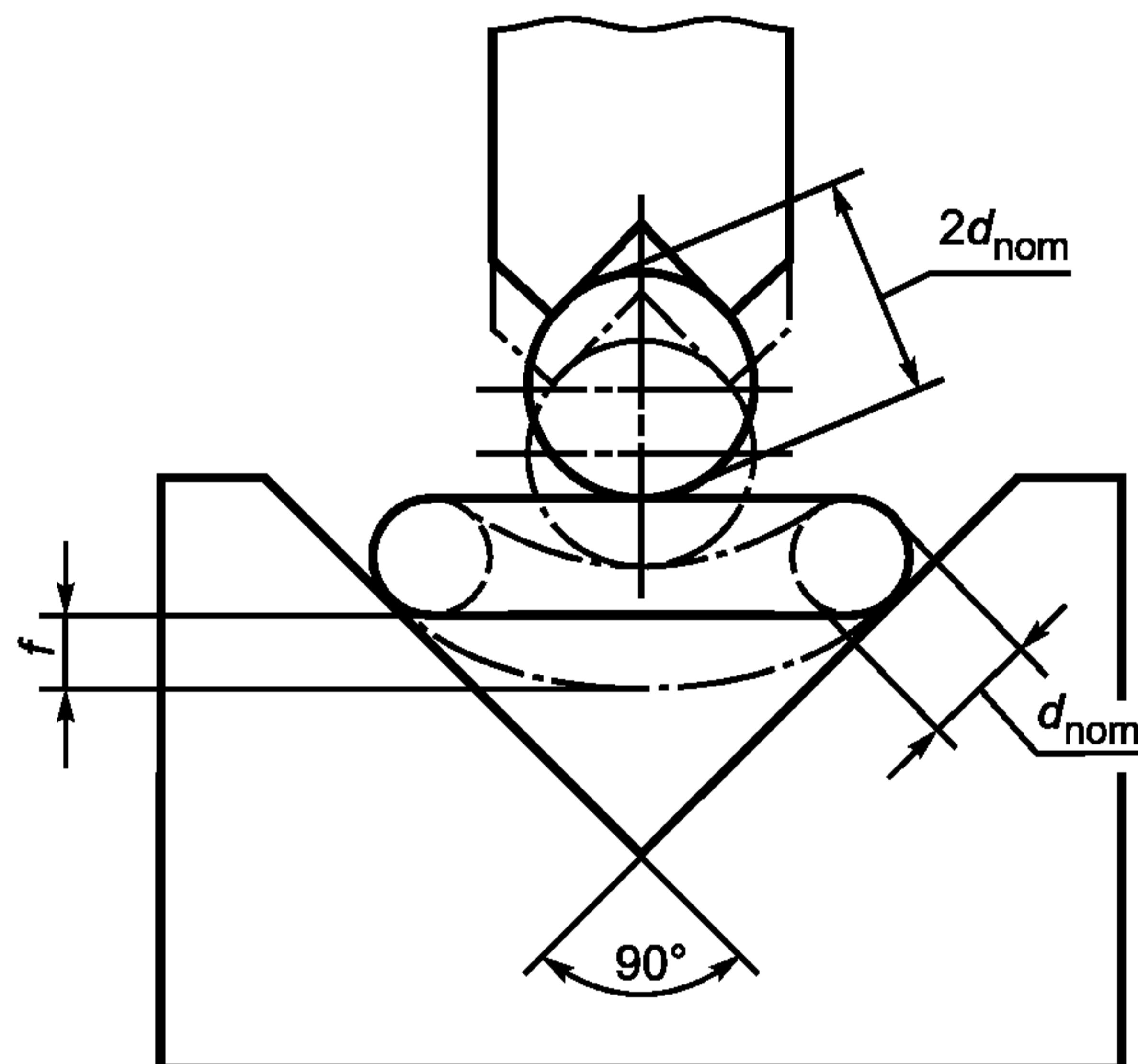
Рисунок 1 — Прогиб f
