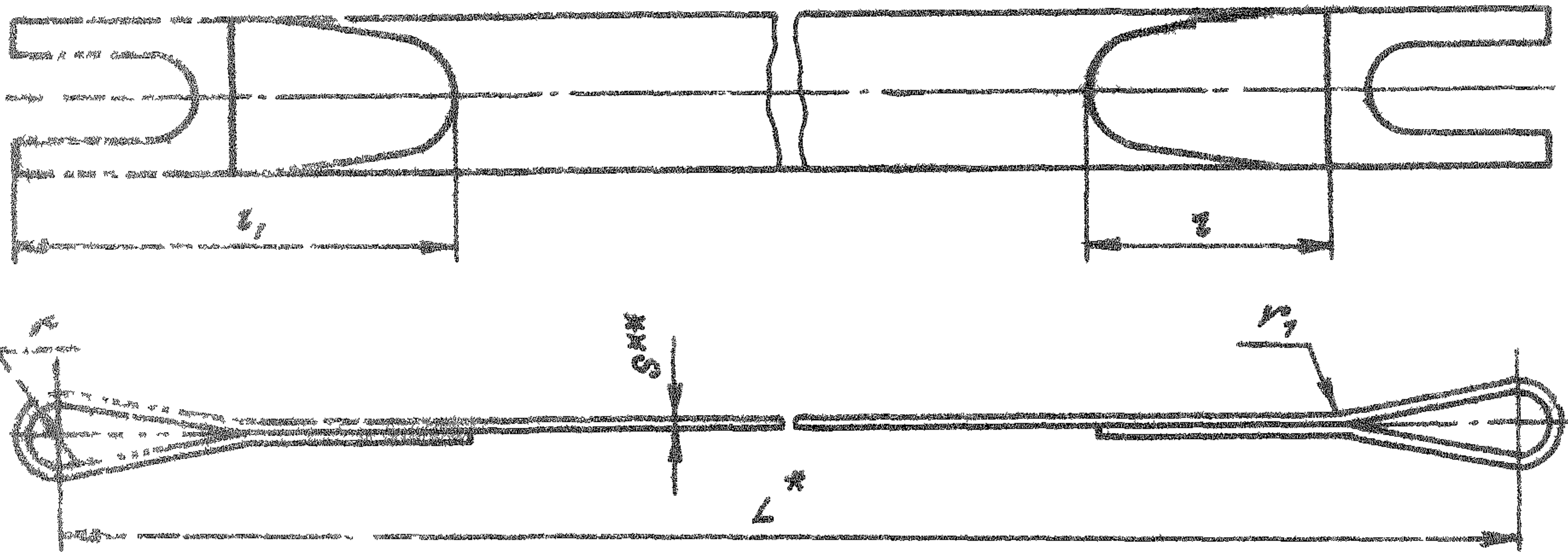
Развертка
