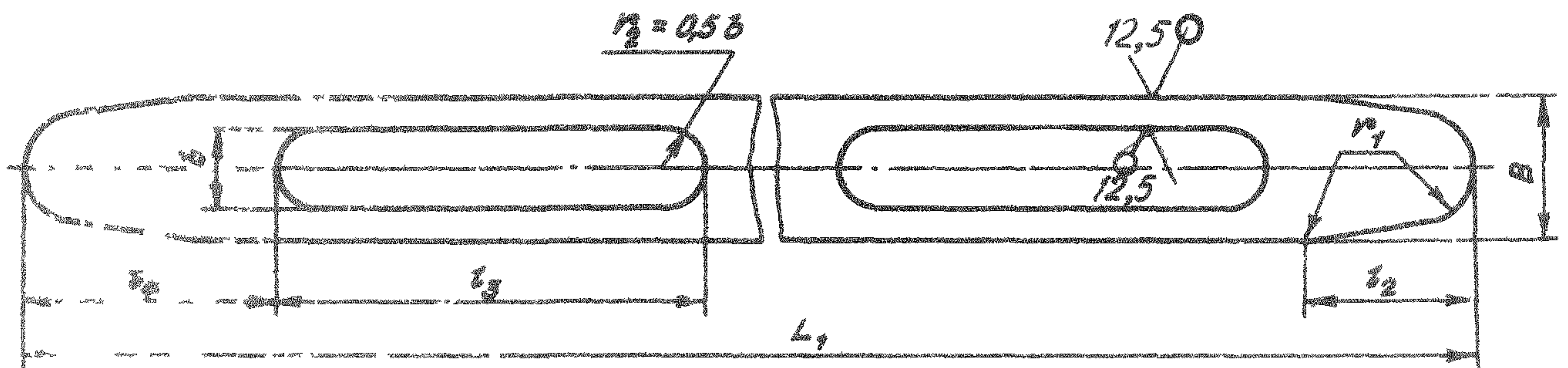
Направление проката
