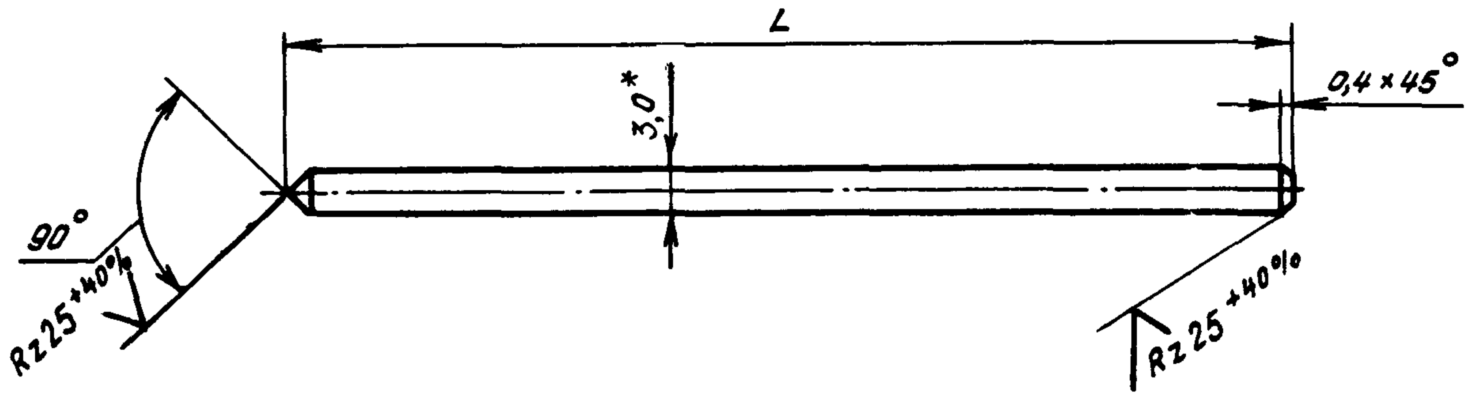
Размеры, мм
