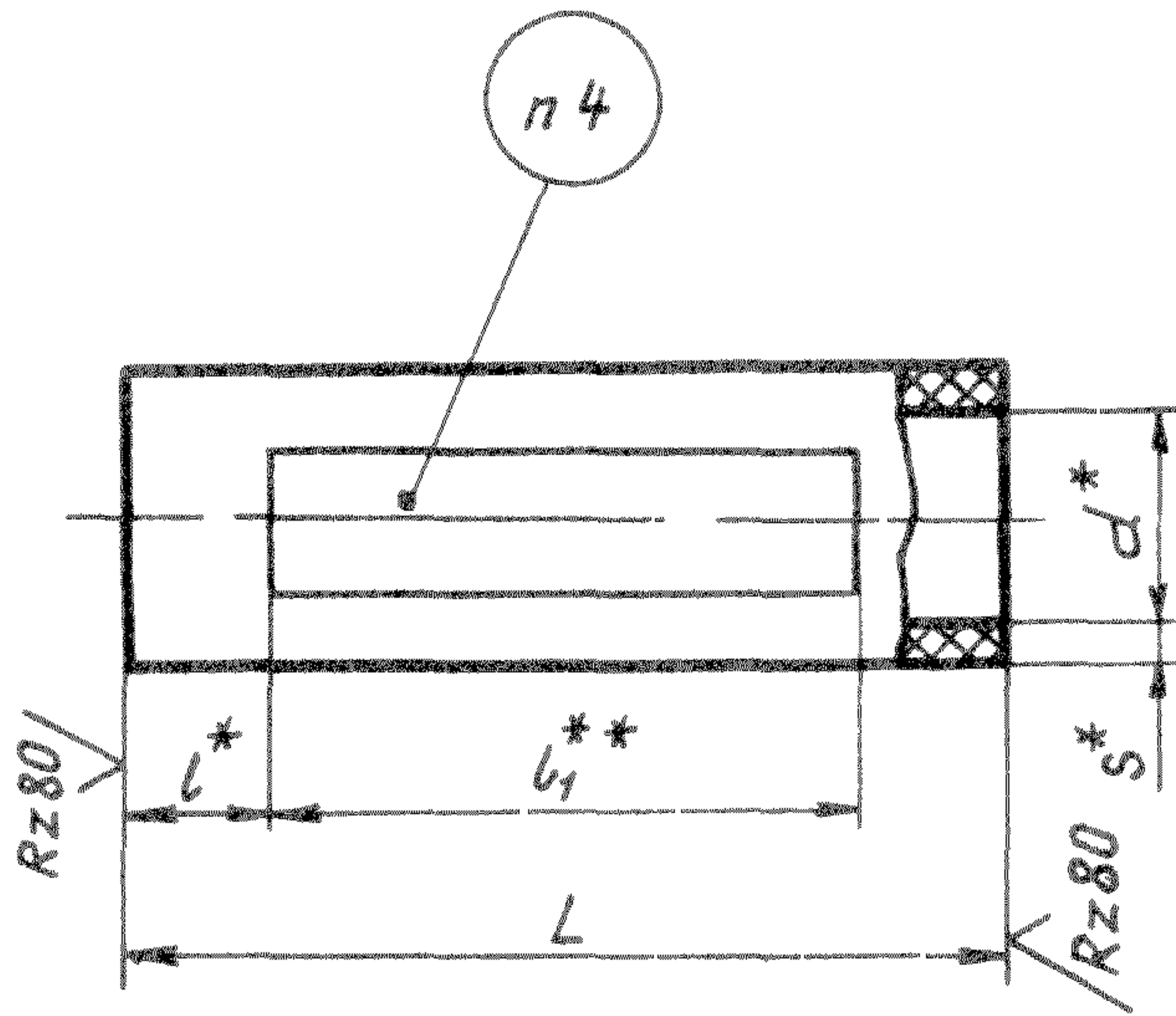
Размеры, мм
