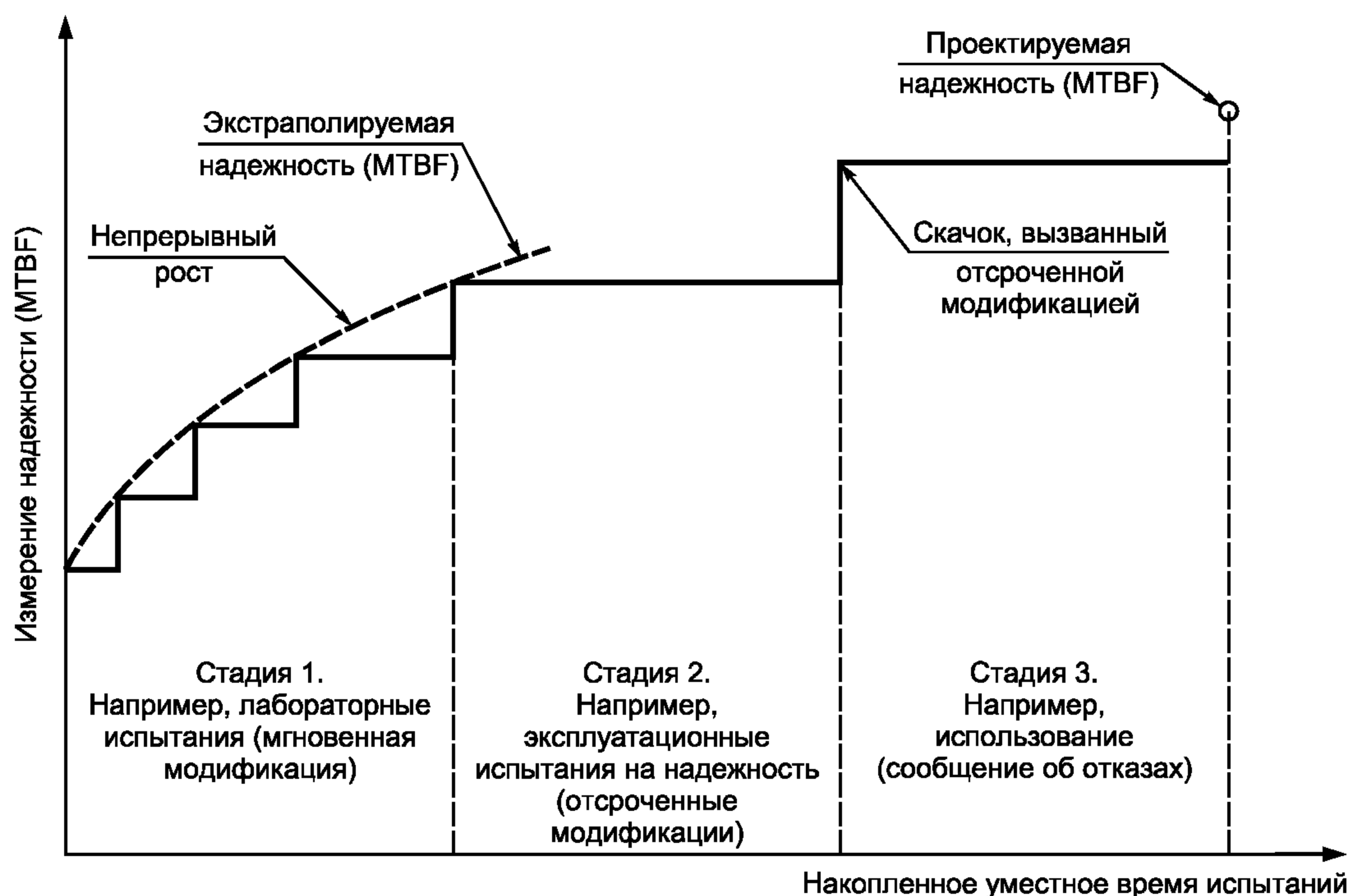
Рисунок 10 — Примеры кривых повышения надежности и скачков
