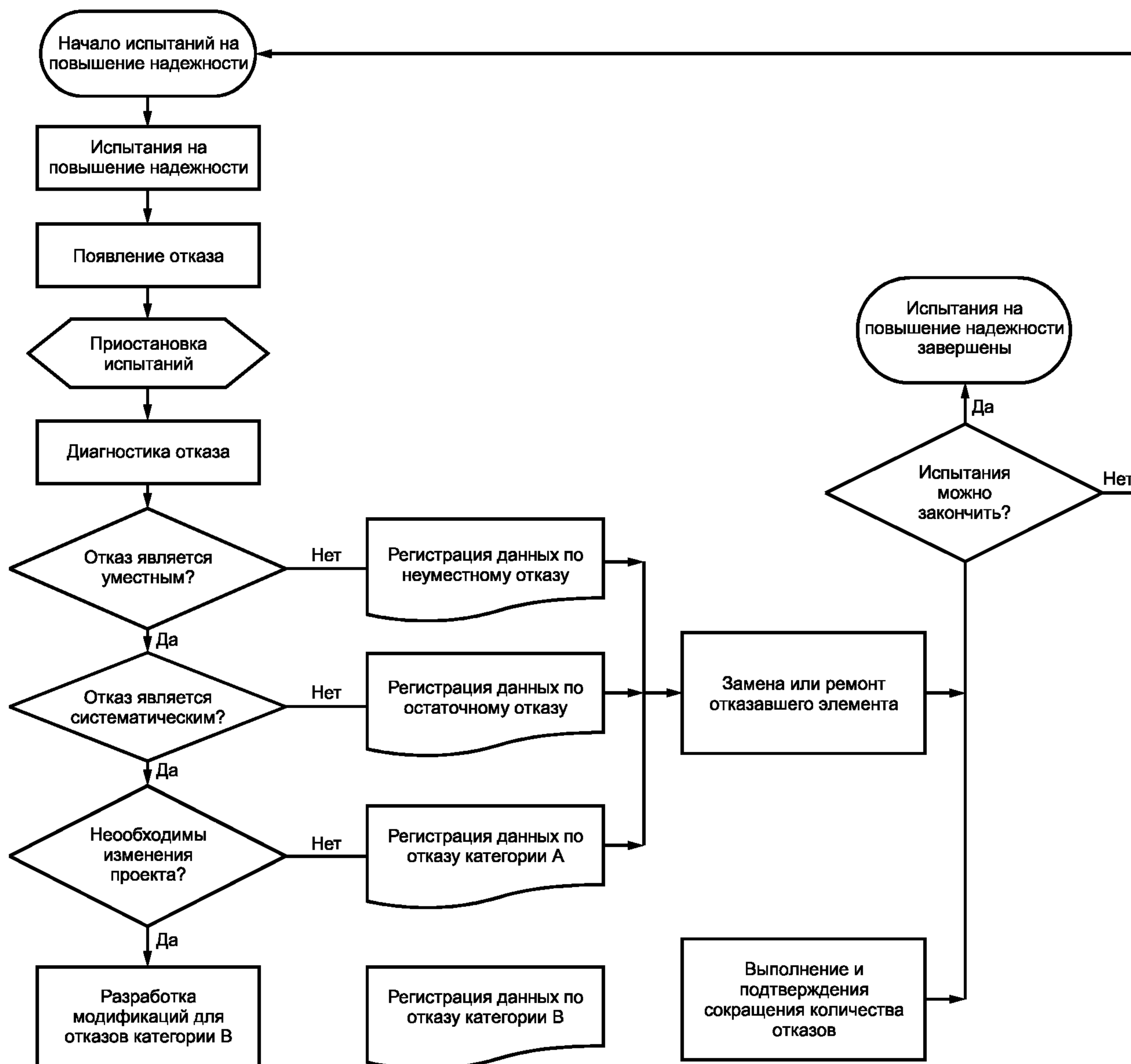
Рисунок 8 — Процесс испытаний на повышение надежности
