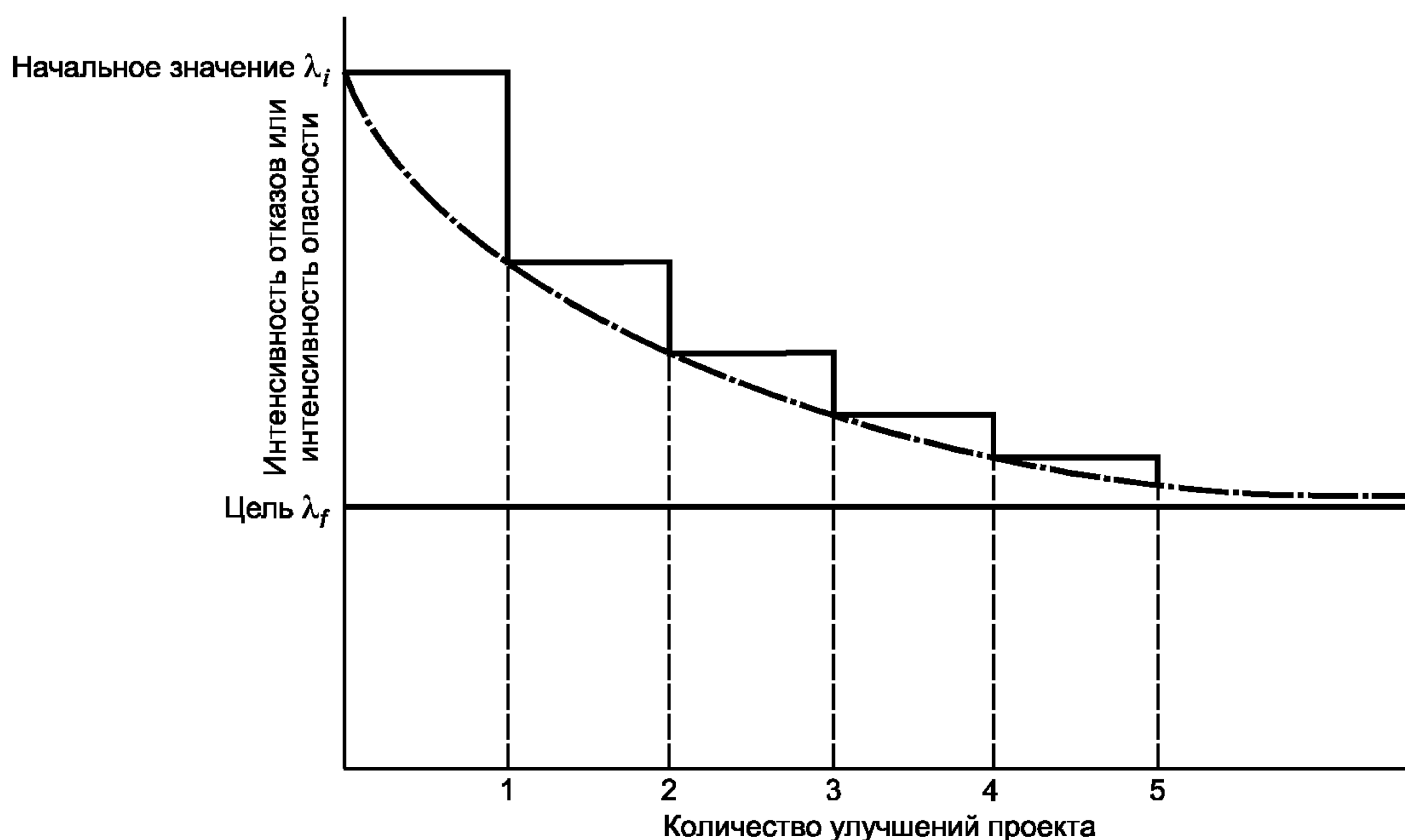
Рисунок 2 — Запланированное улучшение (снижение) эквивалентной интенсивности отказов
