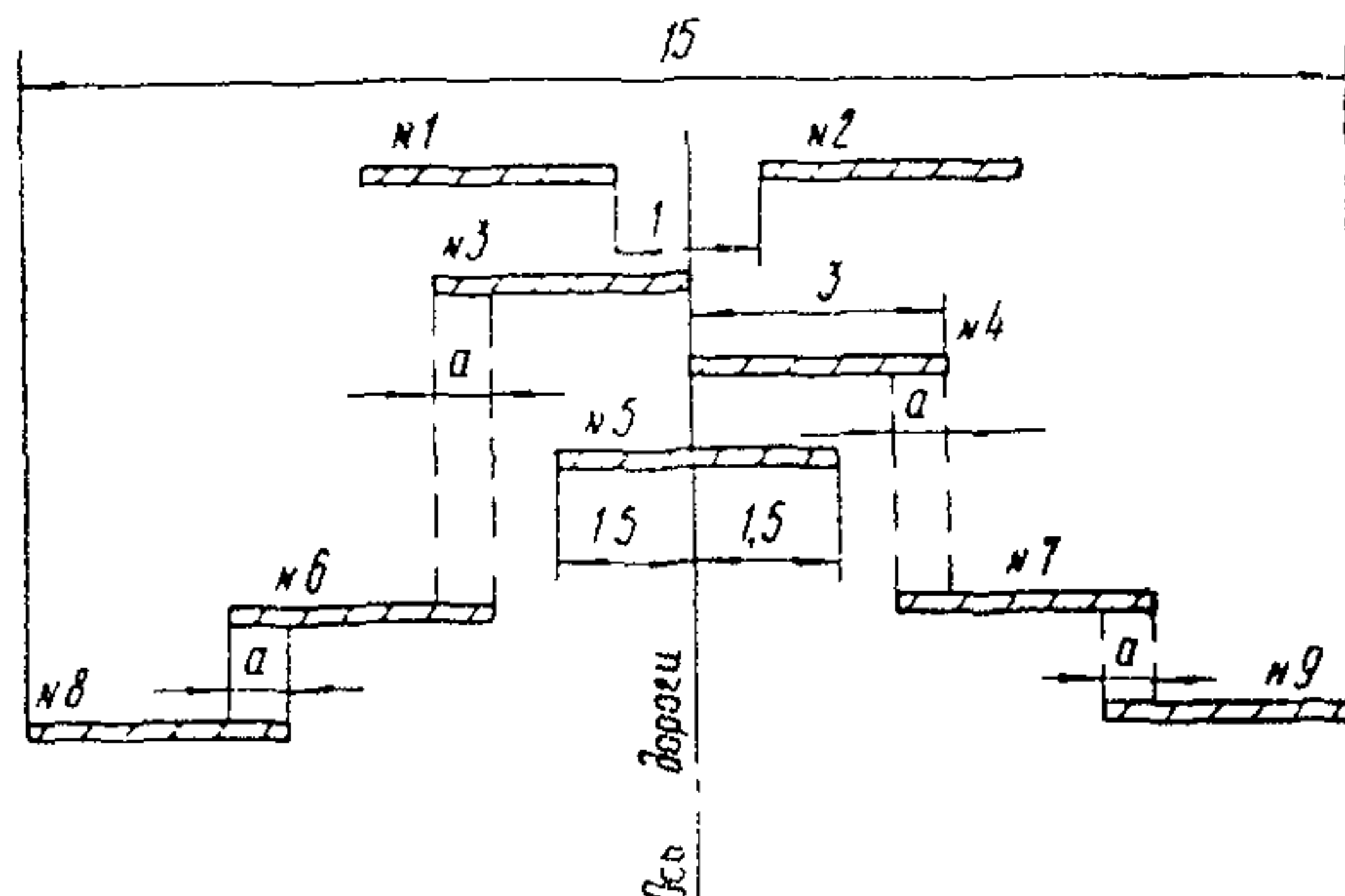
Рис 2 Схема последовательности проходов бульдозера при послойном разравнивании грунта в насыпи
