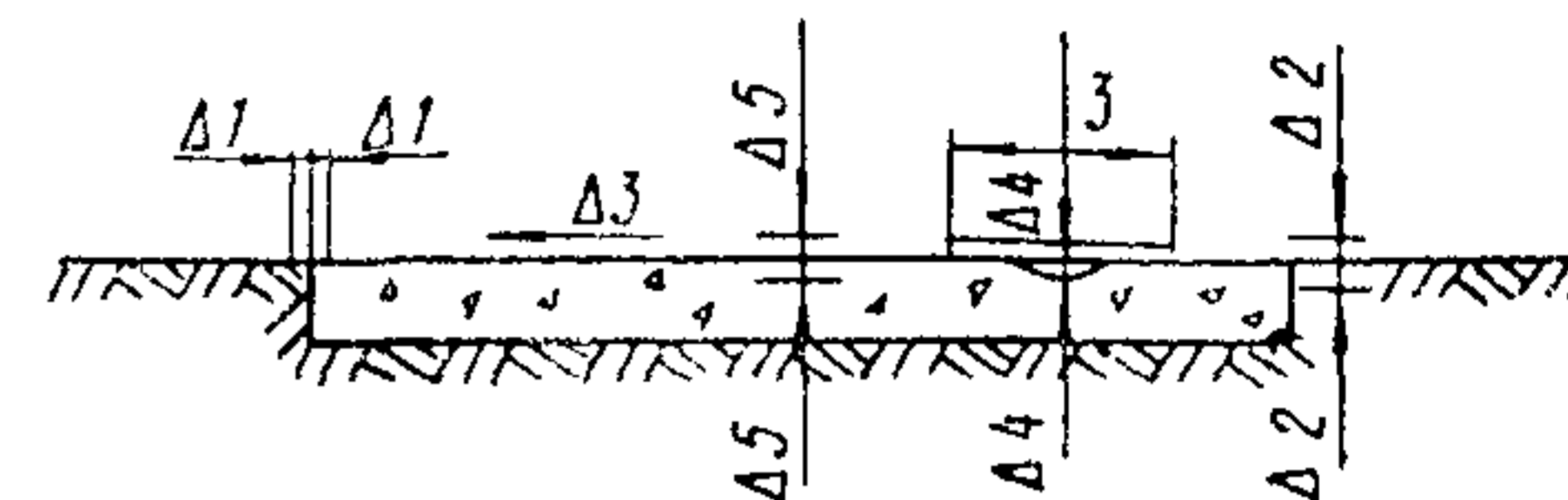
Схема конструкции основания с указанием предельных отклонений
