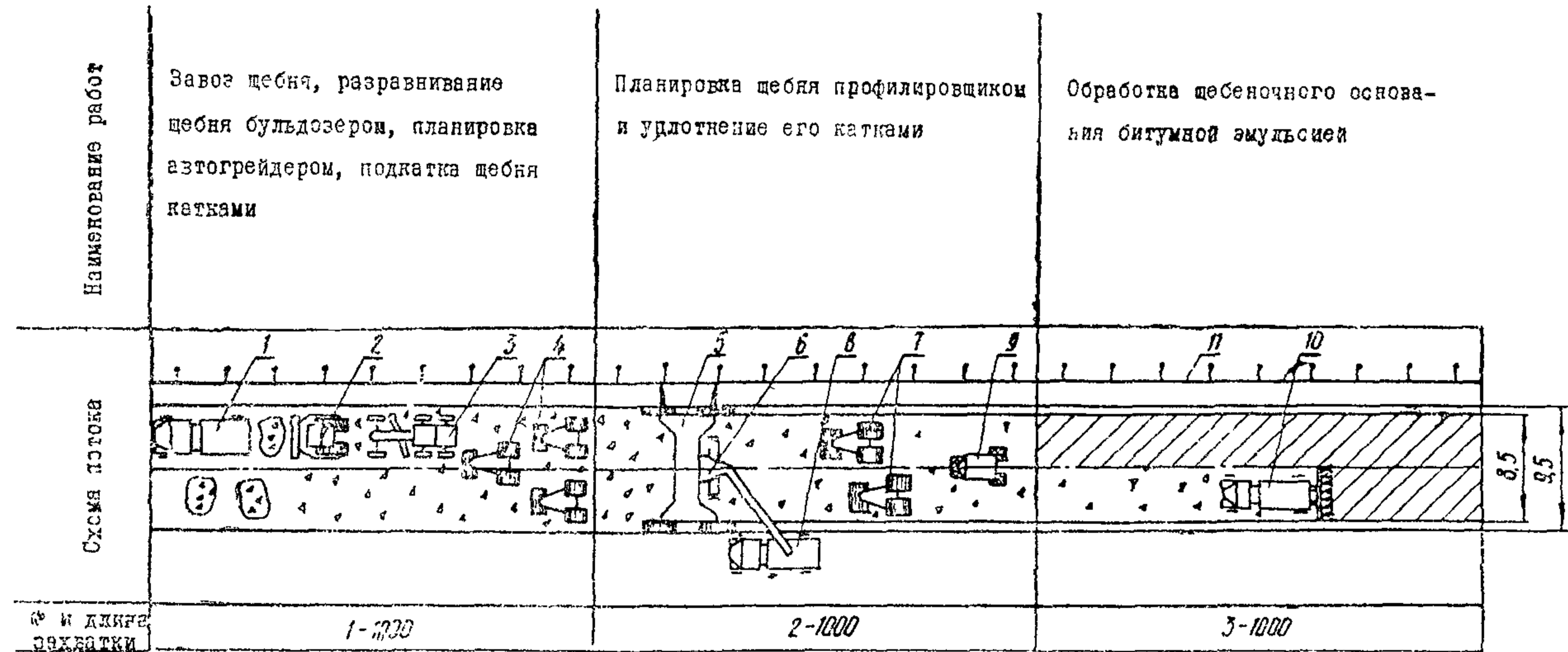
Рис. 2. Технологическая схема погока по устройству щебеночного основания:
