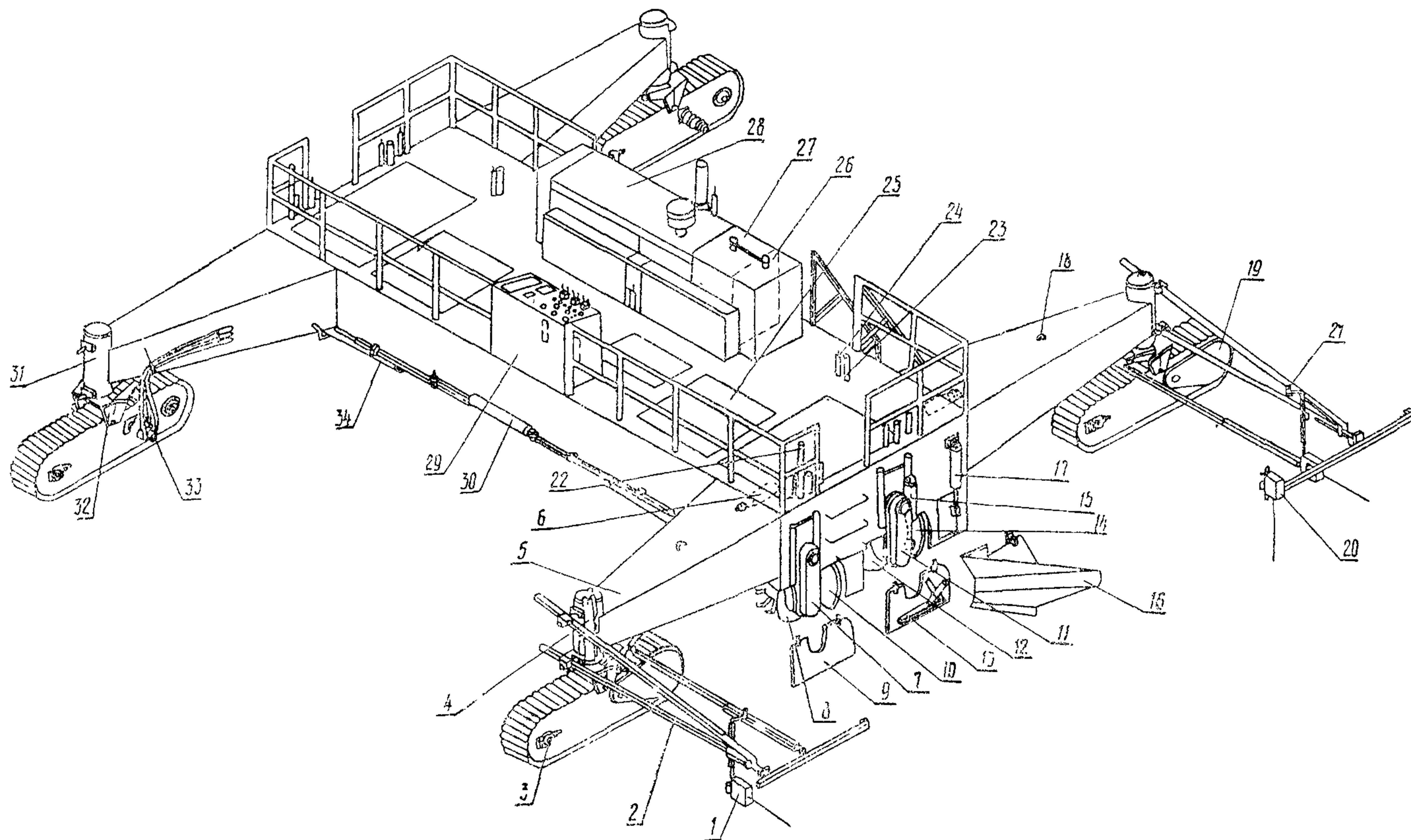
Рис. 1. Общий вид профилировщика ДС-97:
