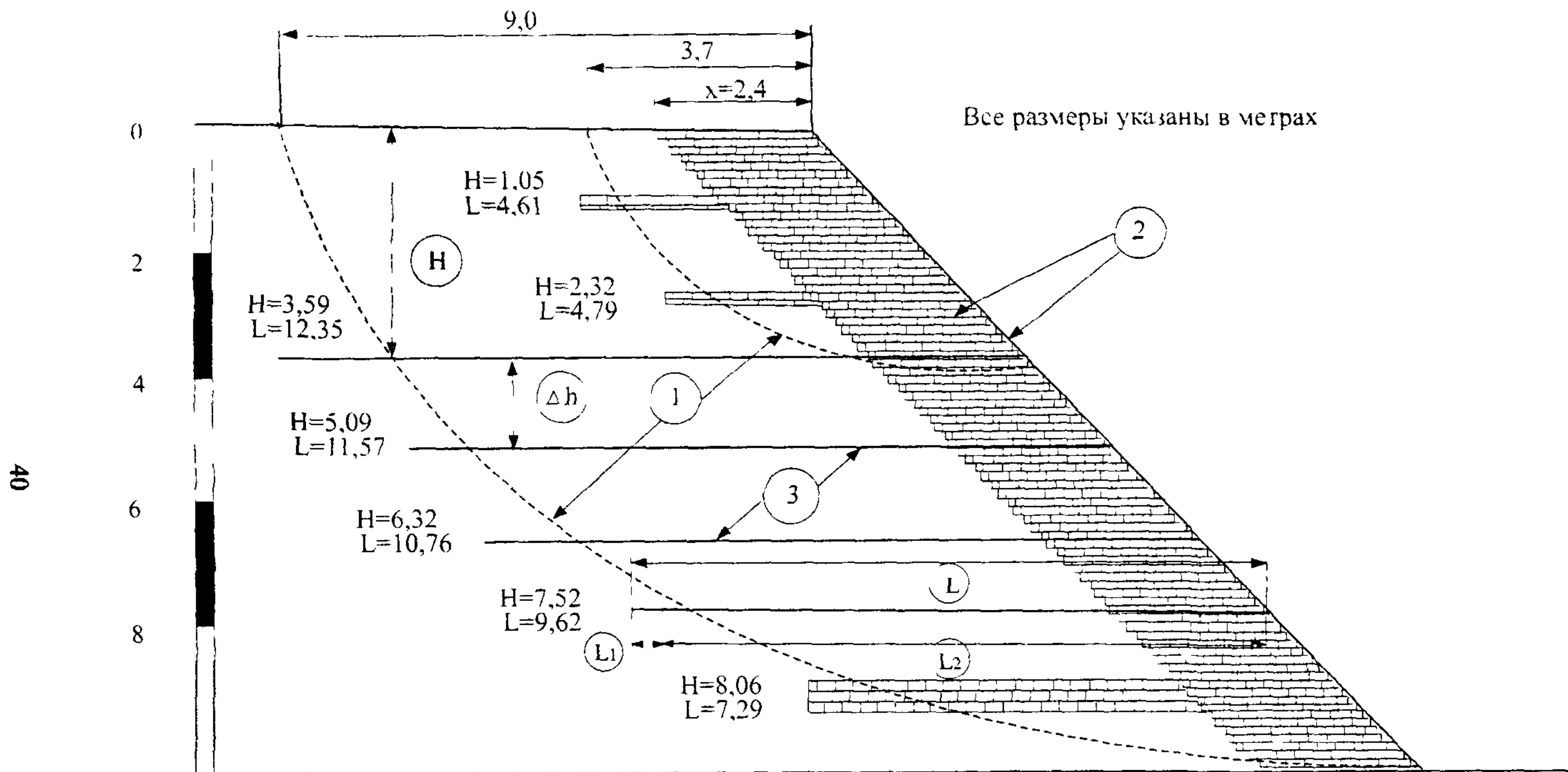
Рис. 11. Схема армирования насыпи с углом скольжения откоса 45^\circ 1 - расчетные поверхности скольжения; 2 - георешетки "Прудон - 494" 3 - геотекстильный материал"
