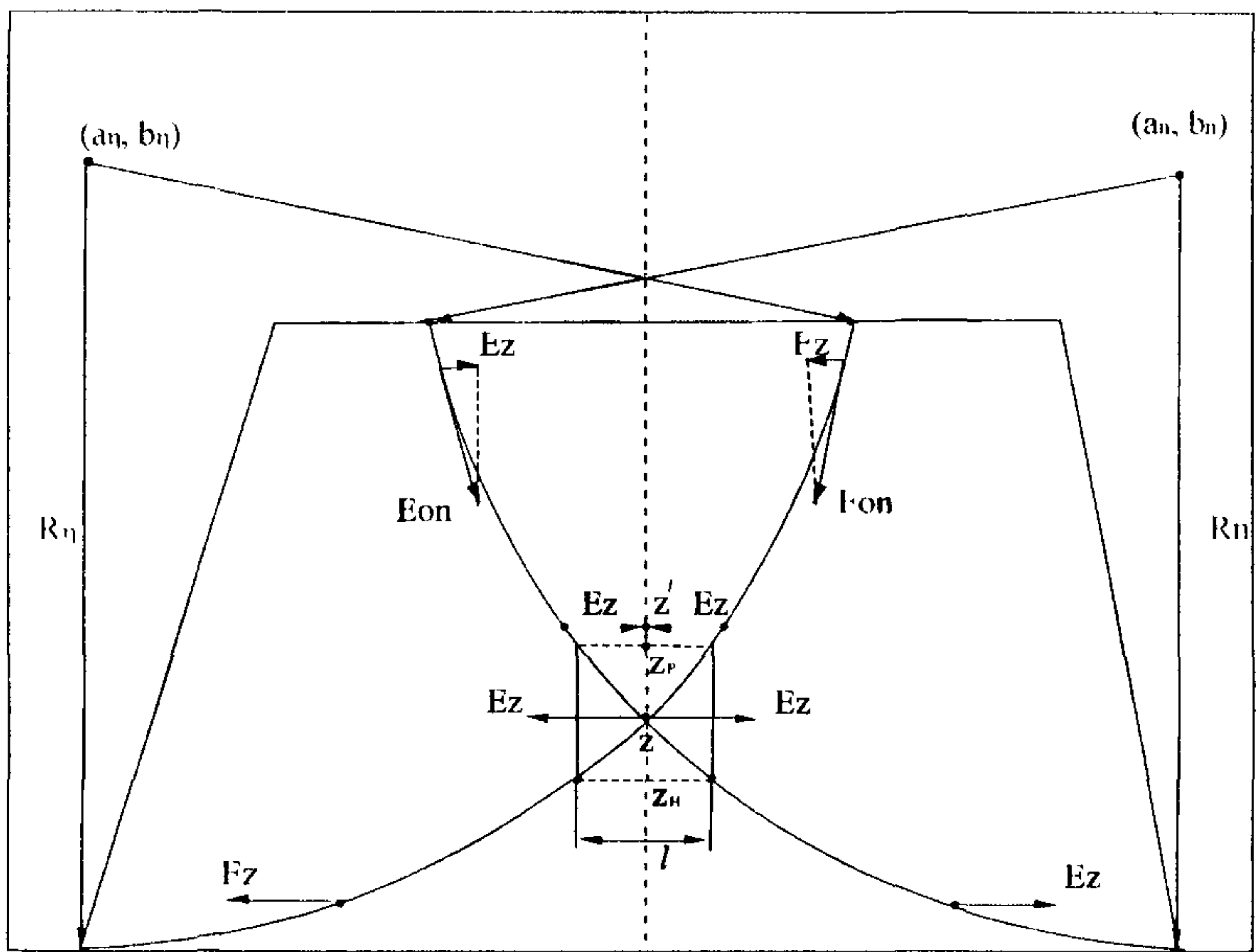
Рис.6. Учет взаимодействия потенциальных поверхностей обрушения неустойчивых частей левого и правого откосов насыпи.
