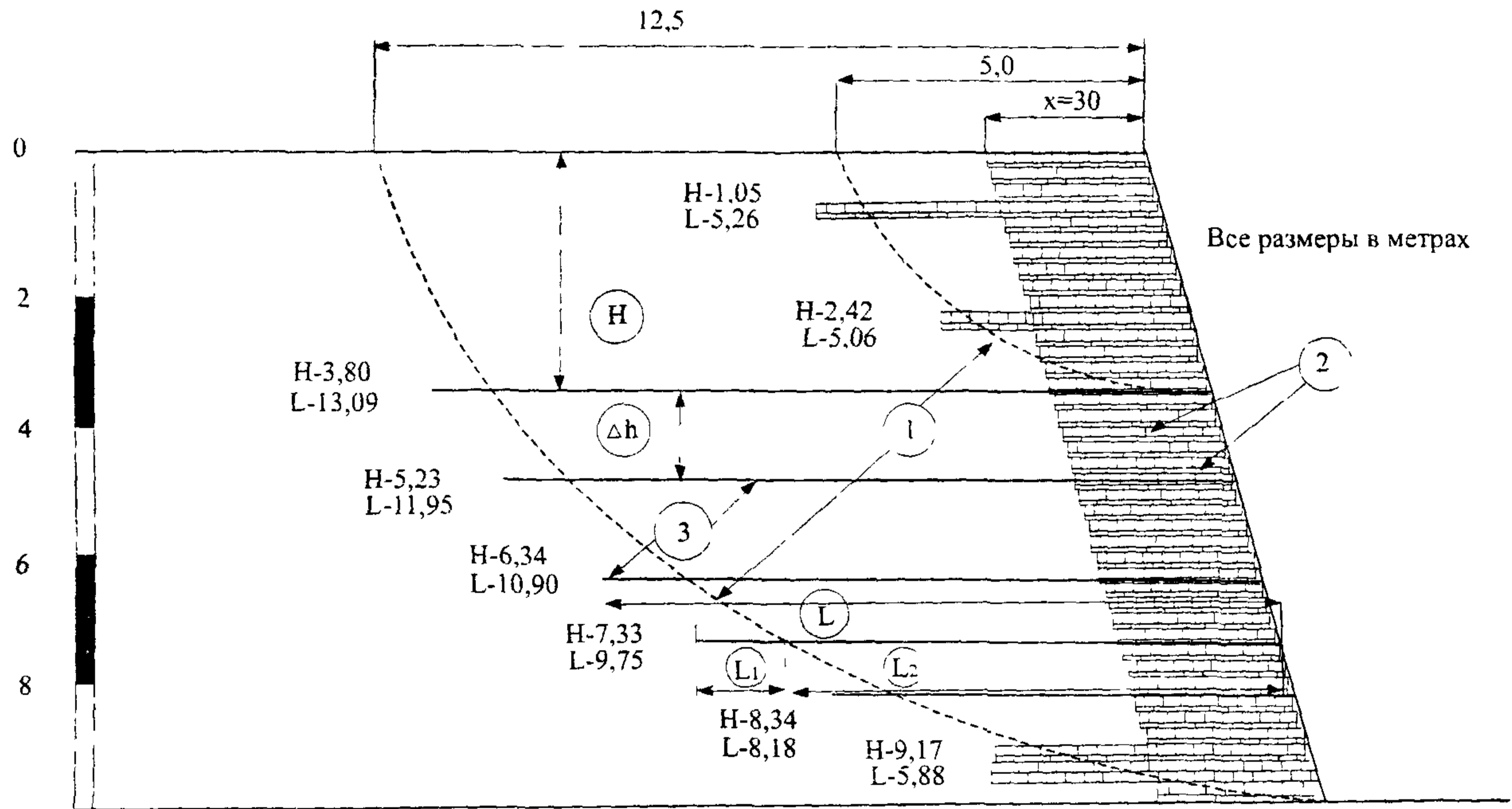
Рис.9. Схема армирования насыпи с углом заложения откоса 75^\circ 1 - расчетные поверхности скольжения; 2 - георешетки "Прудон - 494" 3 - геотекстильный материал
