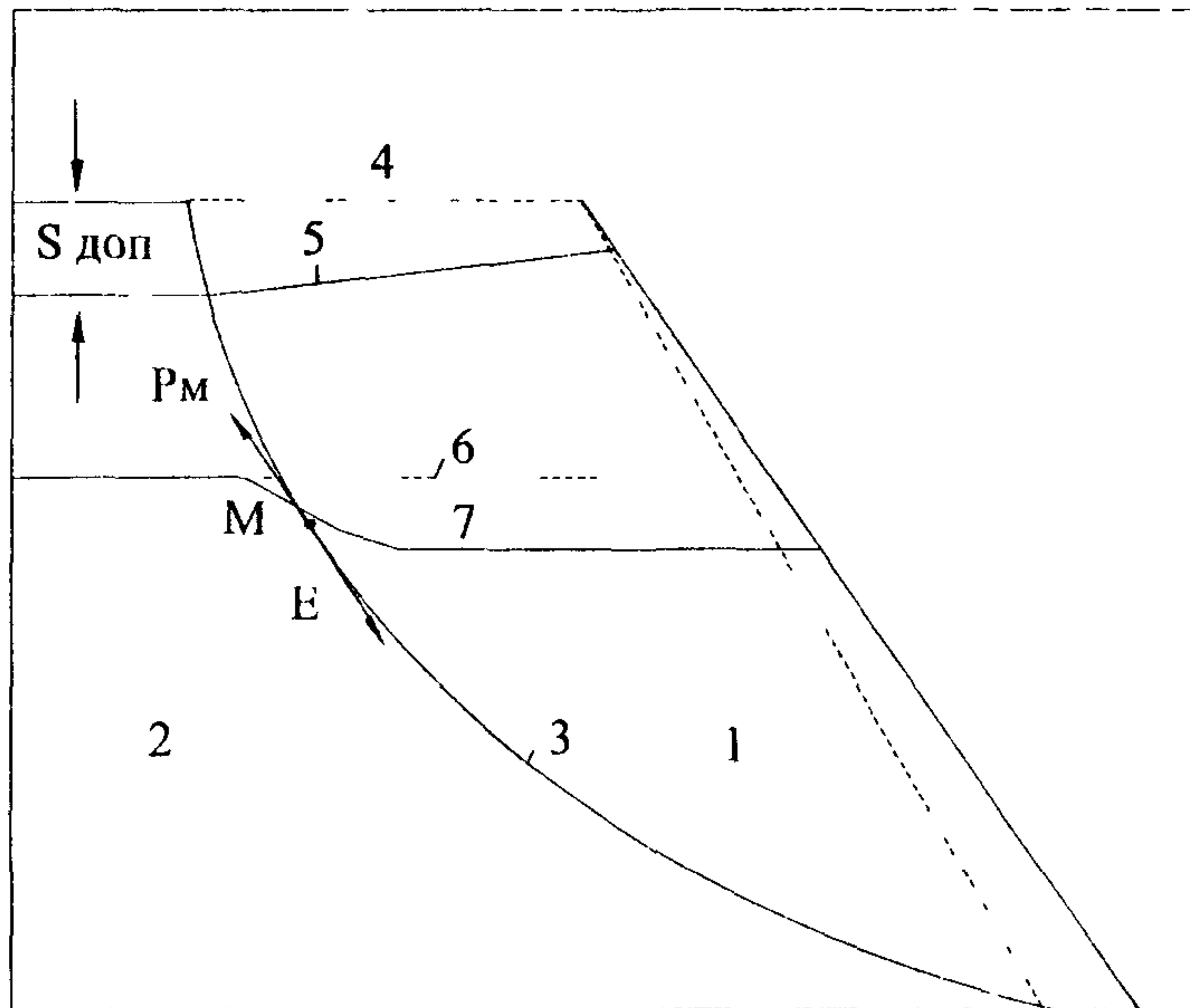
Рис. 2. Схема деформирования армирующей прослойки.
