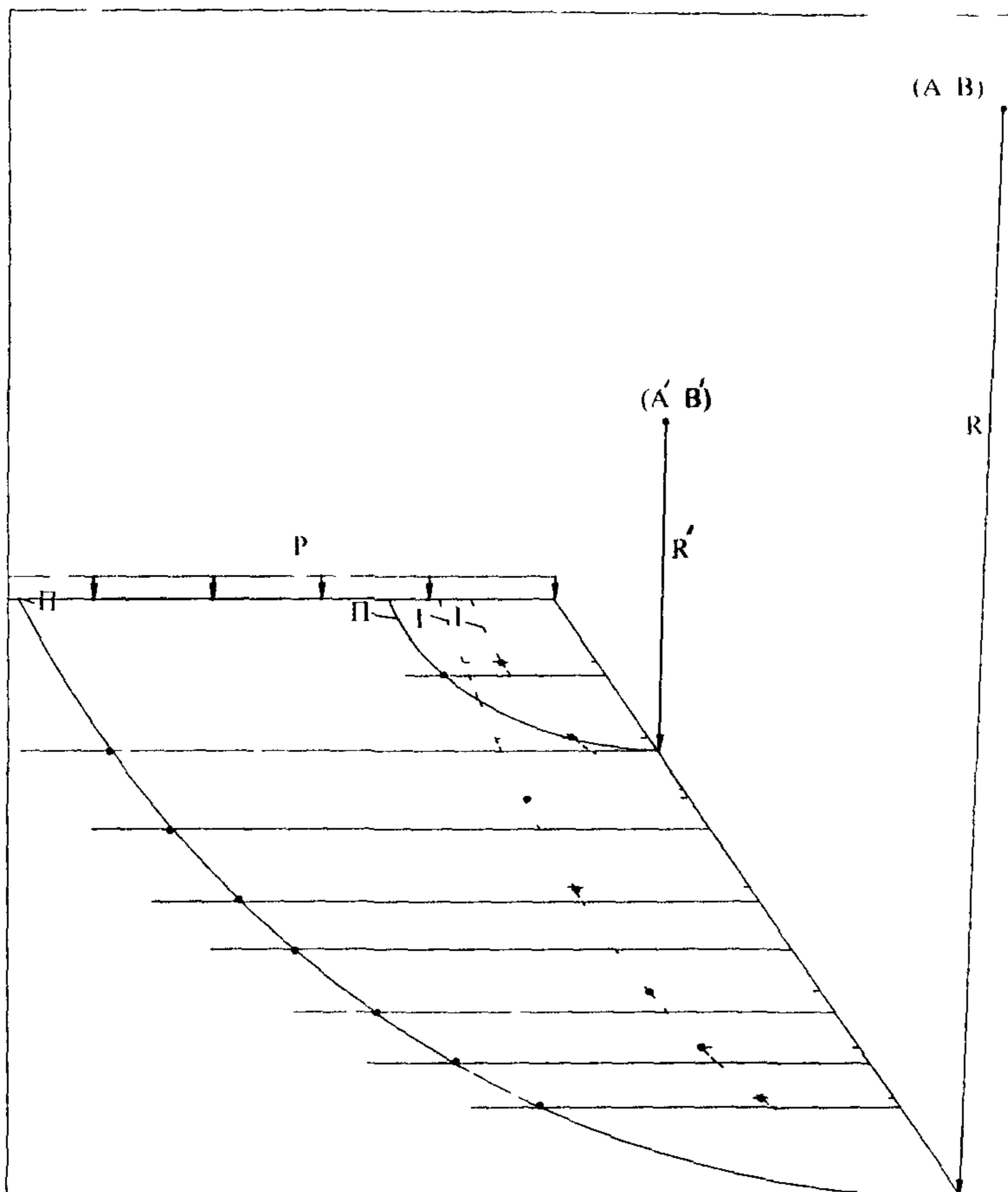
Рис 3 Схемы армирования откоса относительно I критических (штриховые линии, K_{уст} = 0,53 ) и II предельных (сплошные линии, K_{уст} = 1 ) поверхностей обрушения его неустойчивых частей
