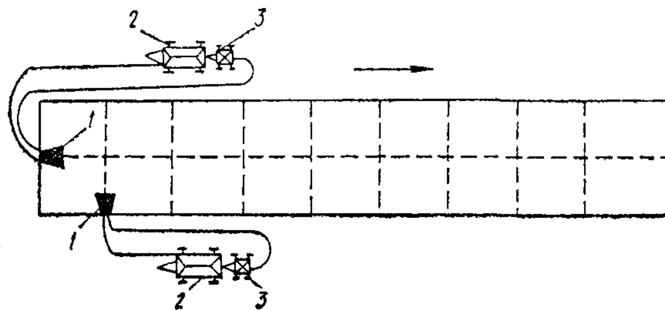
1 — нарезчик Д-432А; 2 — передвижная электростанция; 3 — емкость для воды. Стрелкой указано направление фронта работ.
