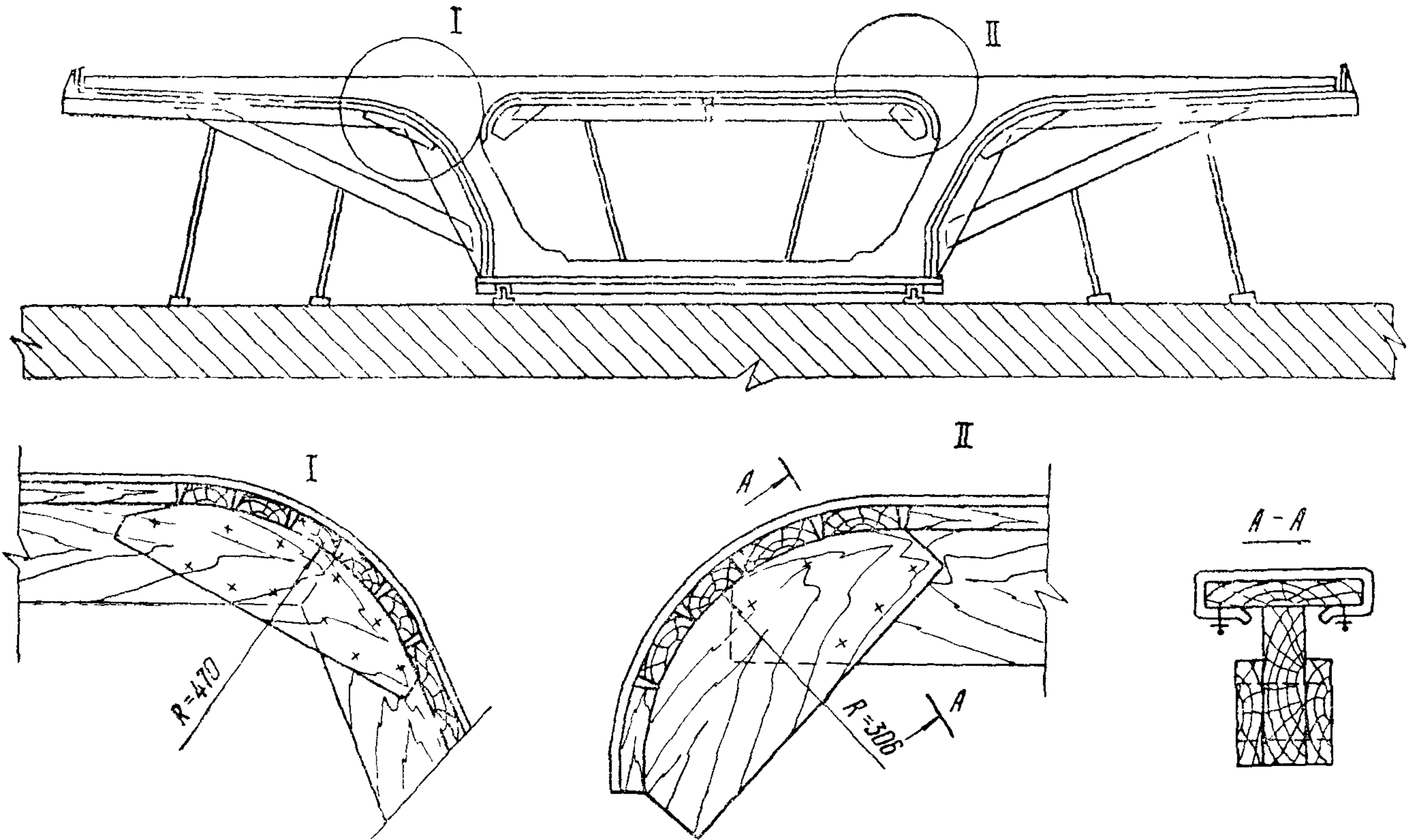
Рис 3 Опалубка стыка блоков
