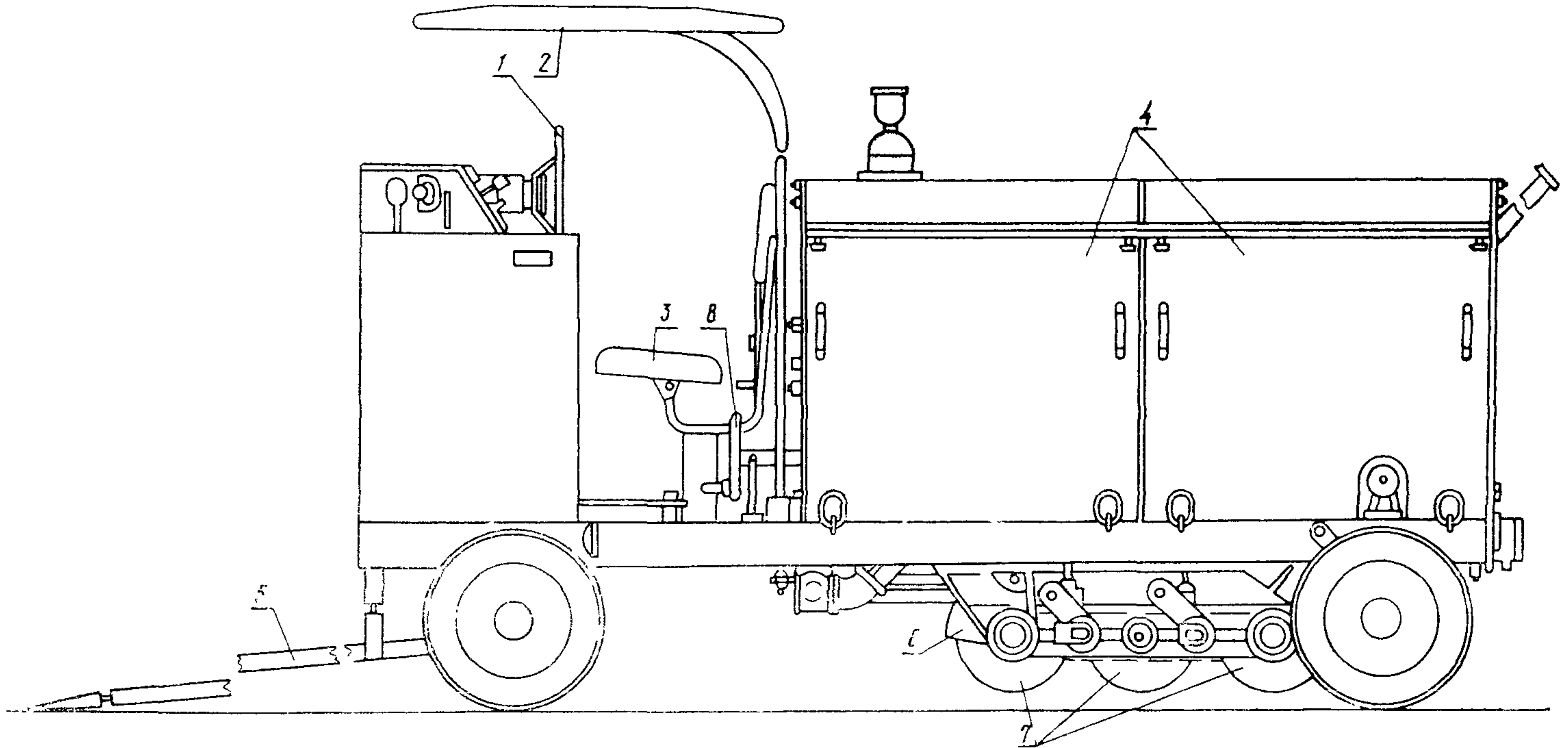
Общий вид нарезчика швов ДС-115:
