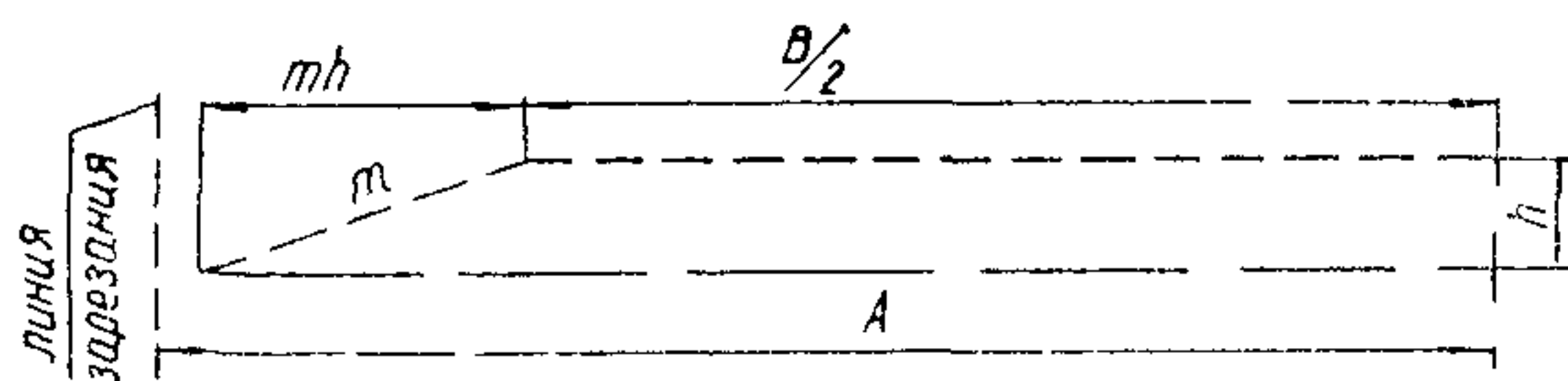
Рис 2. Схема зарезания первого прохода грейдер-элеватора
