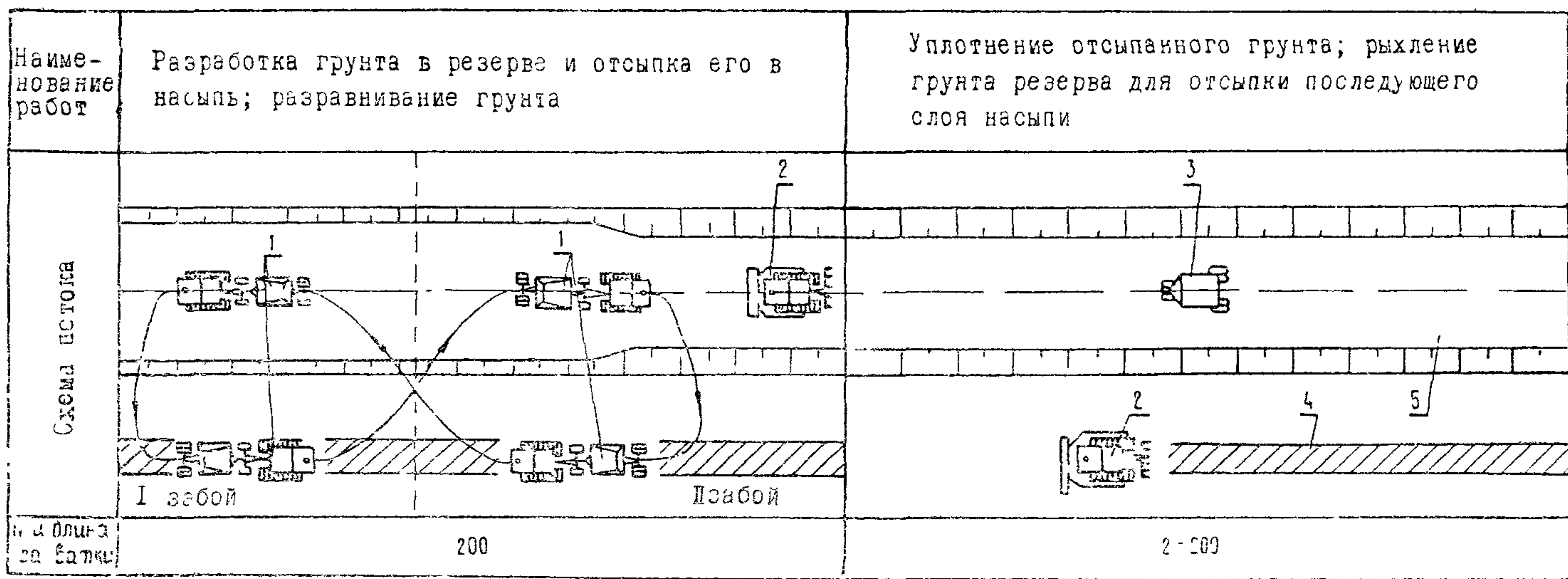
Рис. 1. Технологическая схема возведения земляного полотна:
