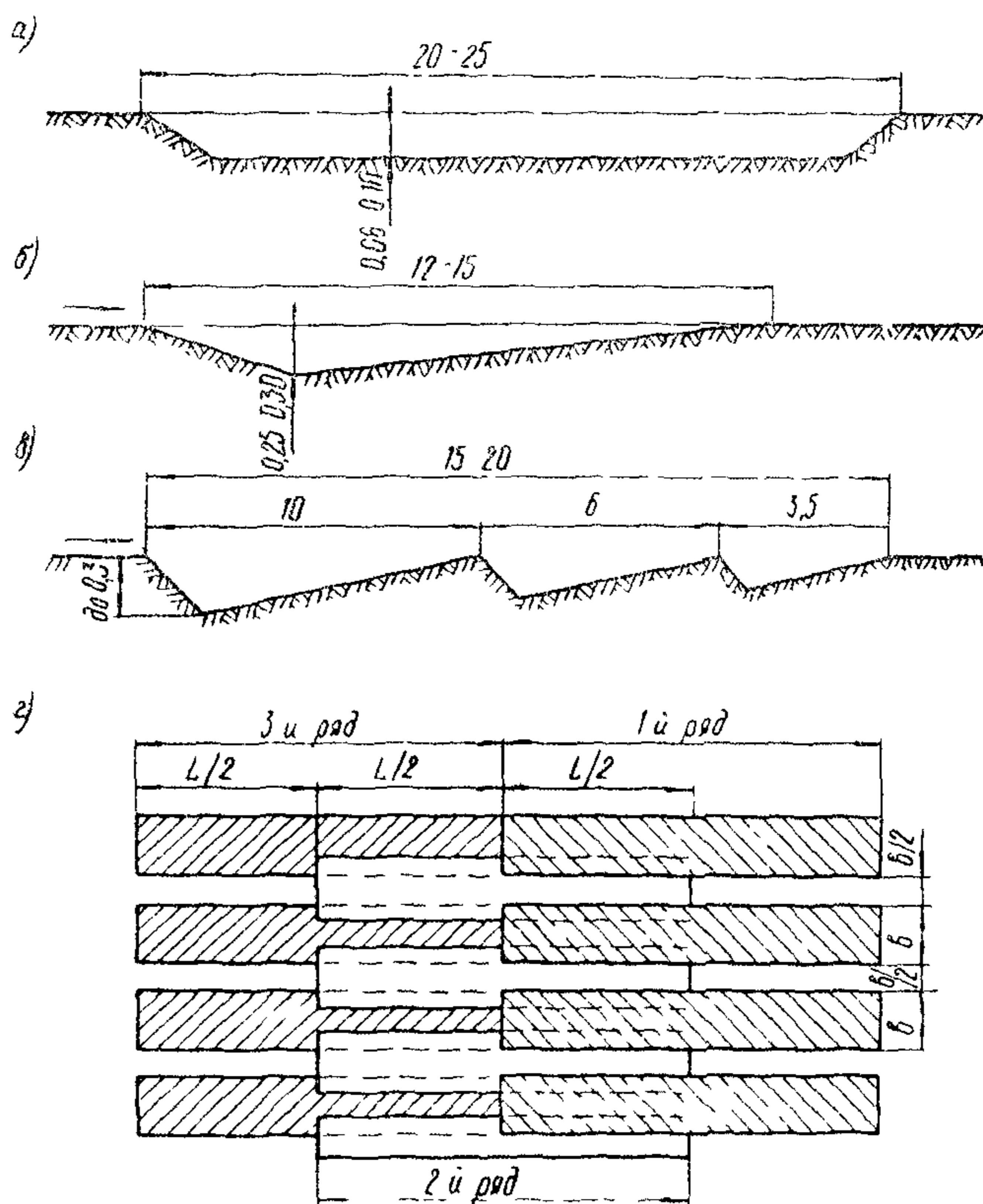
Рис. 2. Схемы зарезания грунта скрепером. а—обычная; б—клиновья, в—гребенчатая; г—ребристо-шахматная (стрелкой показано направление движения машины), L —длина набора грунта; в —ширина резания грунта
