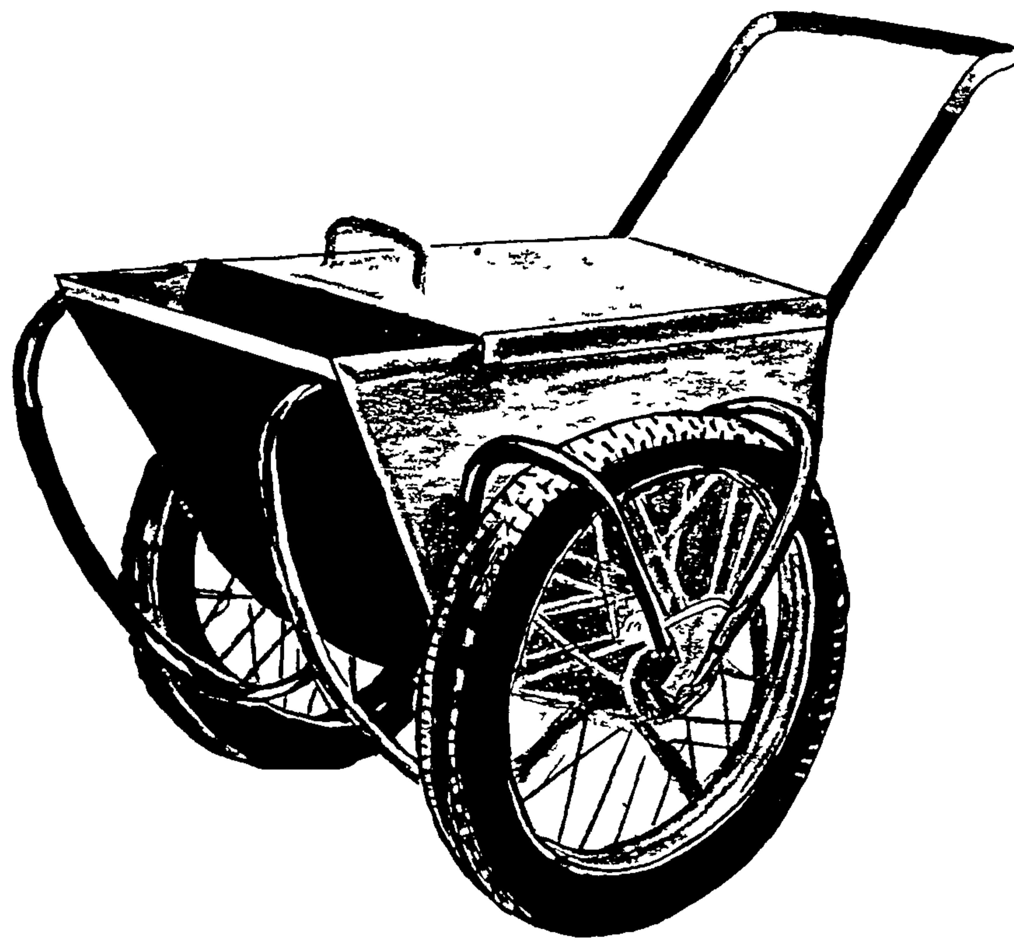
Рисунок 7 – Тележка на пневмоходу для перевозки мраморных плит
