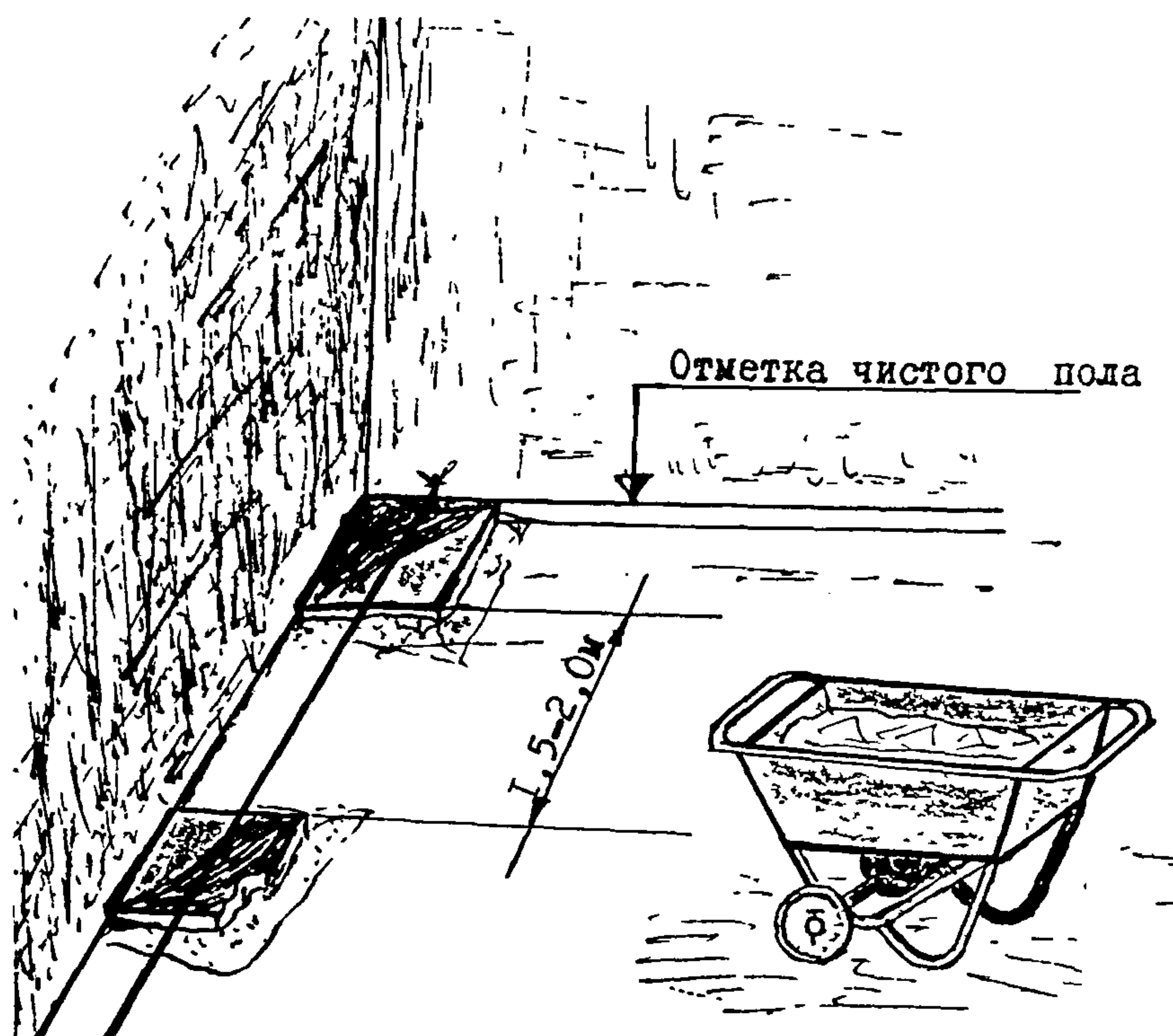
Рисунок 10 – Установка маяков
