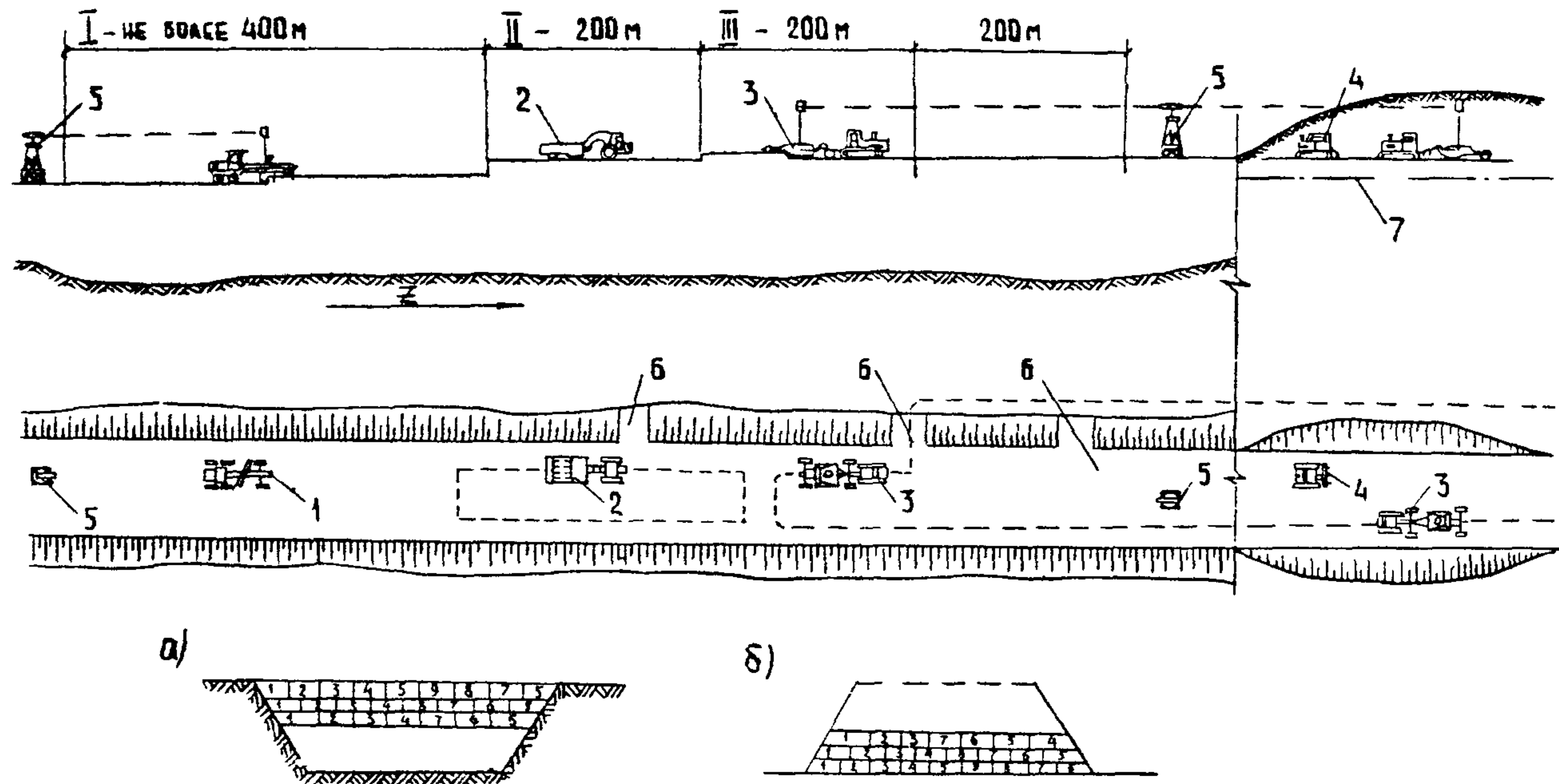
Рис.6. Схема организации строительной площадки:
