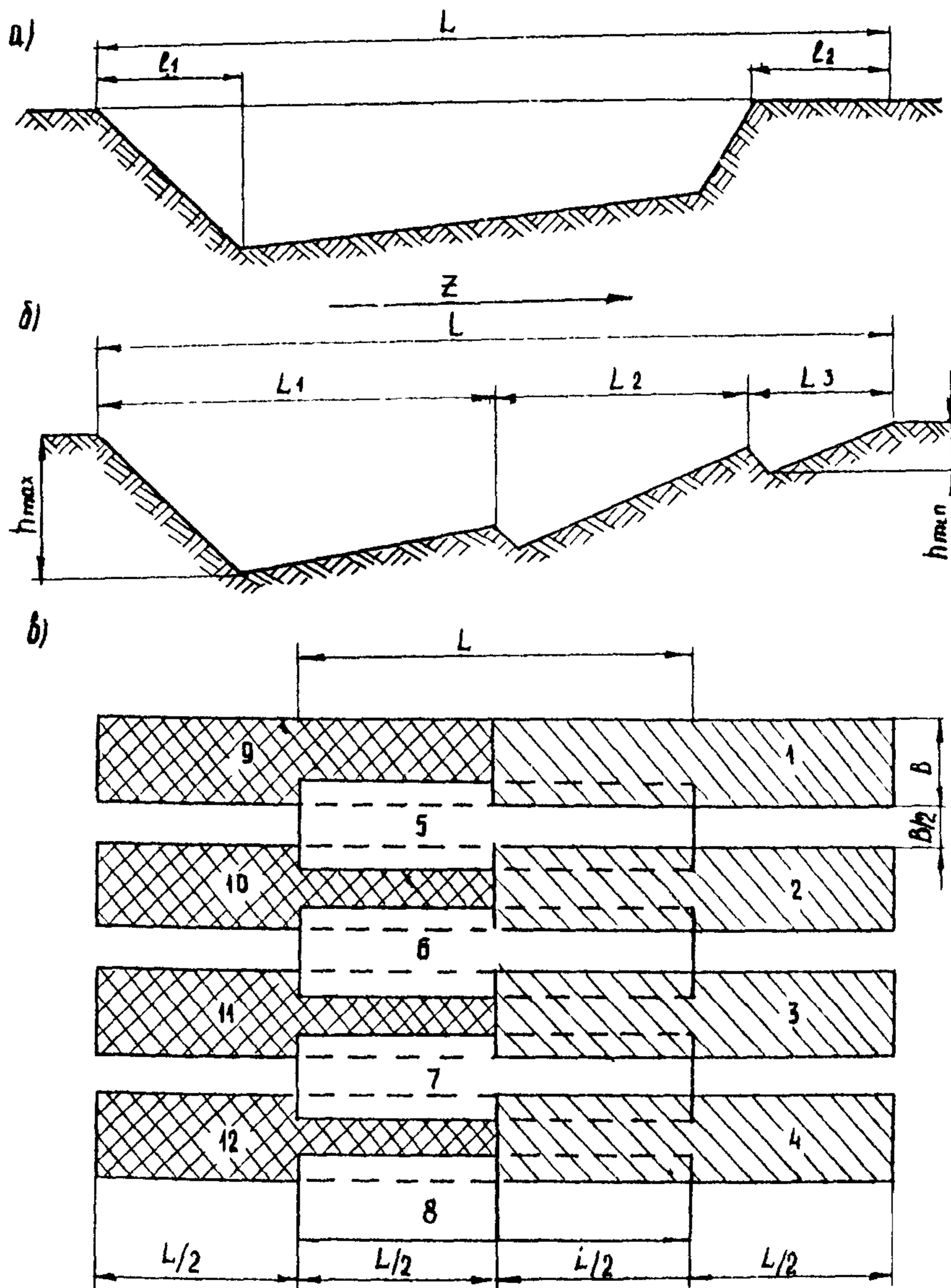
Рис. 8. Способы резания грунта скреперами: а - обычный; б - гребенчатый; в - ребристо-шахматный; Z - направленные движения; L - длина набора грунта; l_1 - путь резания; l_2 - путь извлечения ковша скрепера; h - глубина резания; L_1, L_2, L_3 - длина пути набора при 1 - 3 зарезании грунта; 1 - 12 - проходы скреперов; B - ширина захвата
