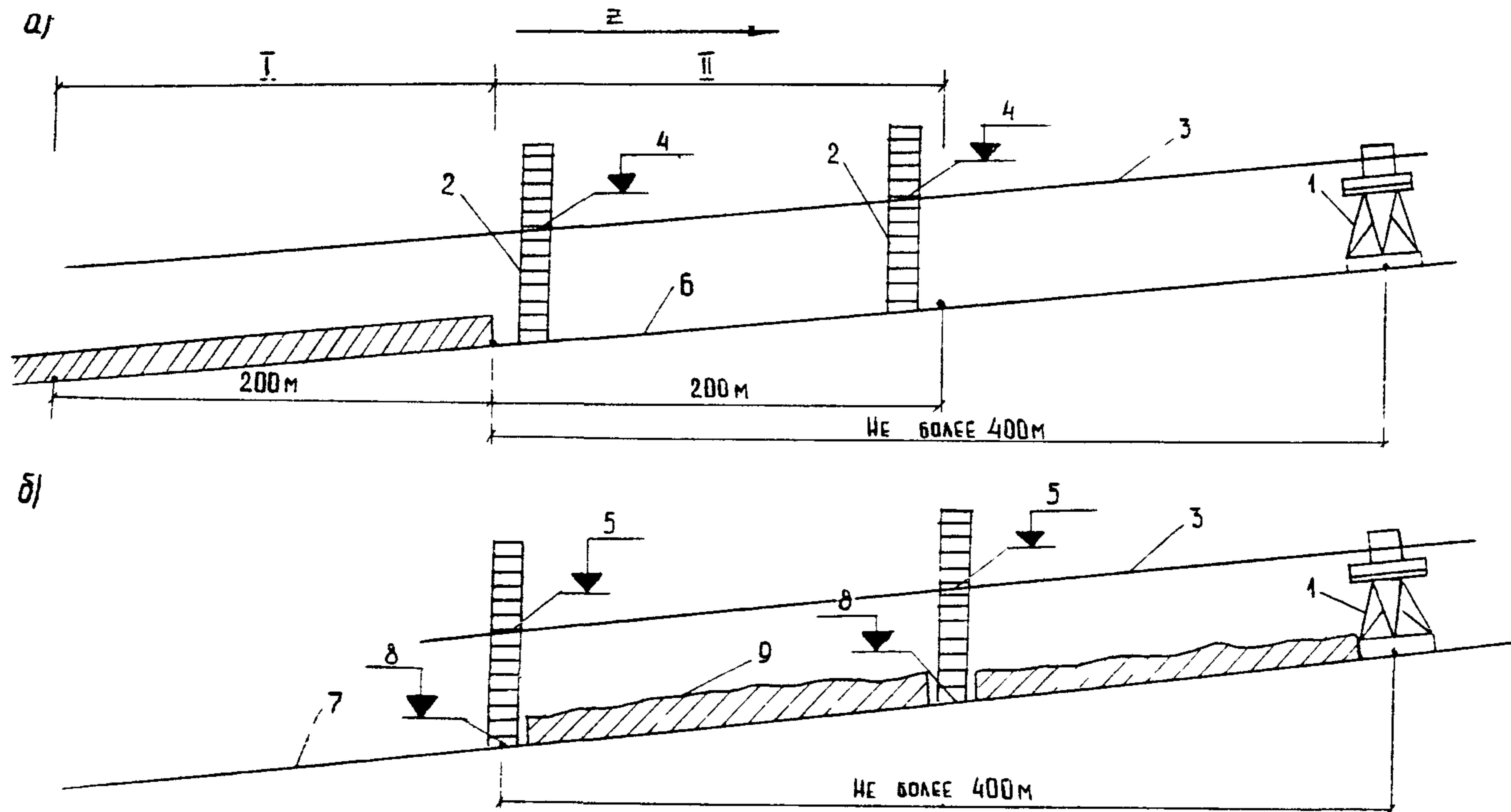
Рис. 7. Схема установки поста лазерного излучателя:
