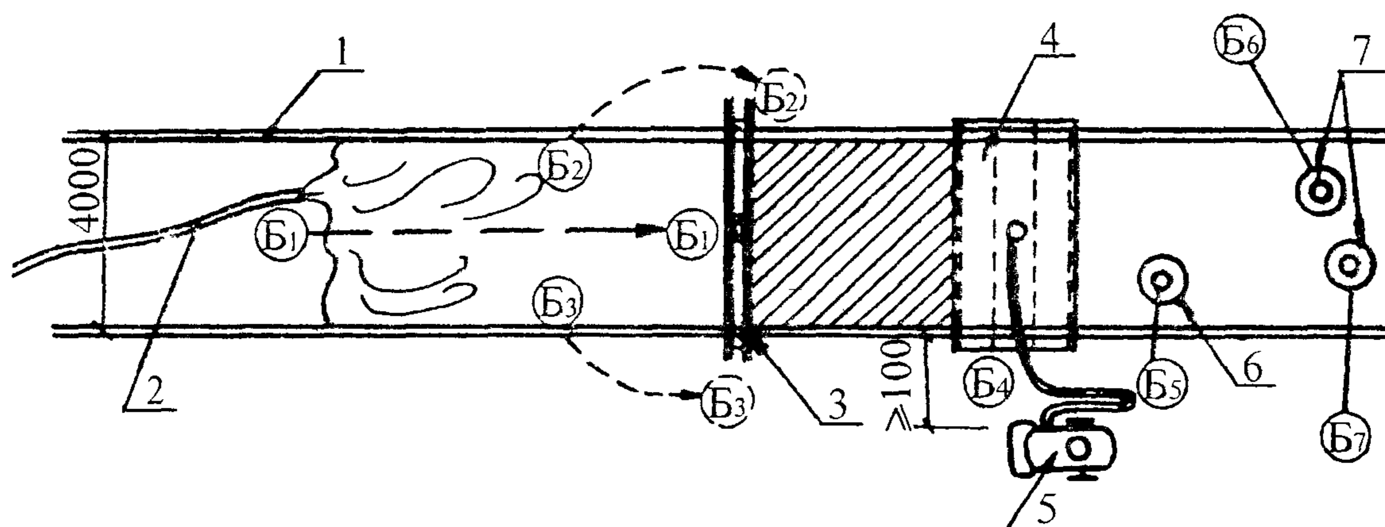
Рисунок 6 — Схема организации рабочего места
