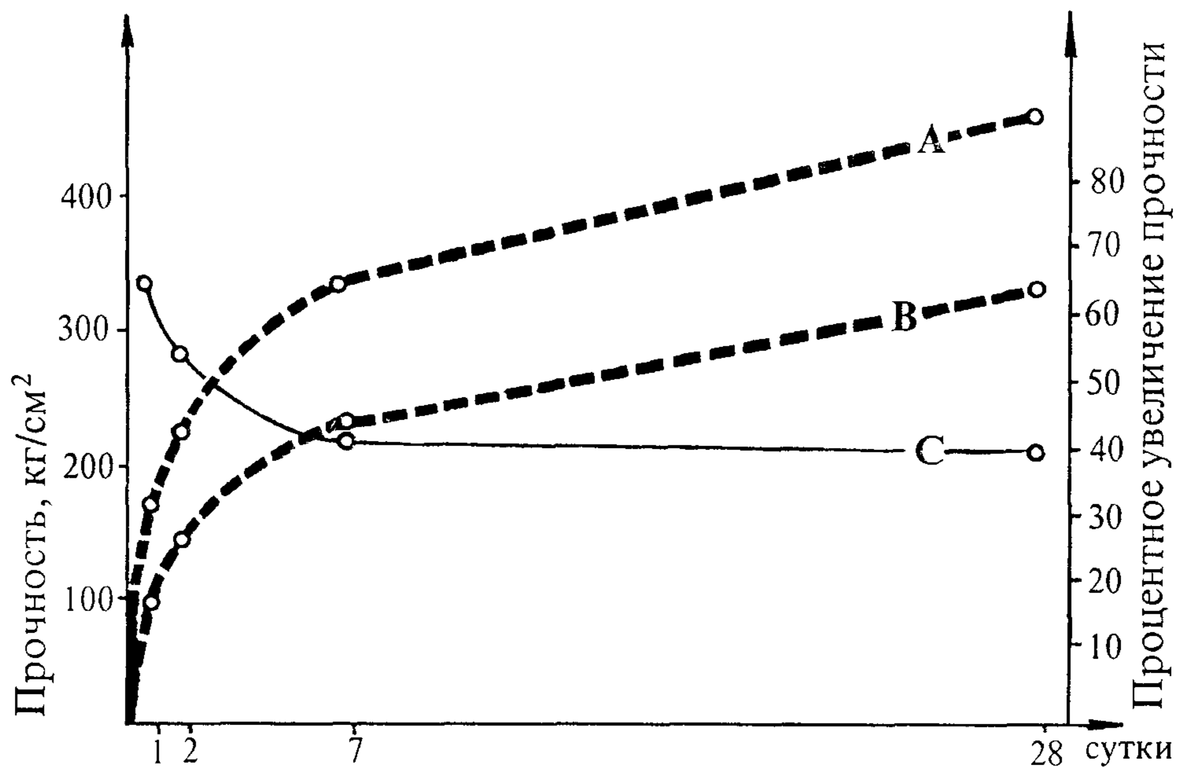
Рисунок 1 — График нарастания прочности бетона во времени: A — при вакуумной обработке; B — при естественном твердении; C — процентное увеличение прочности бетона после вакуумной обработки.
