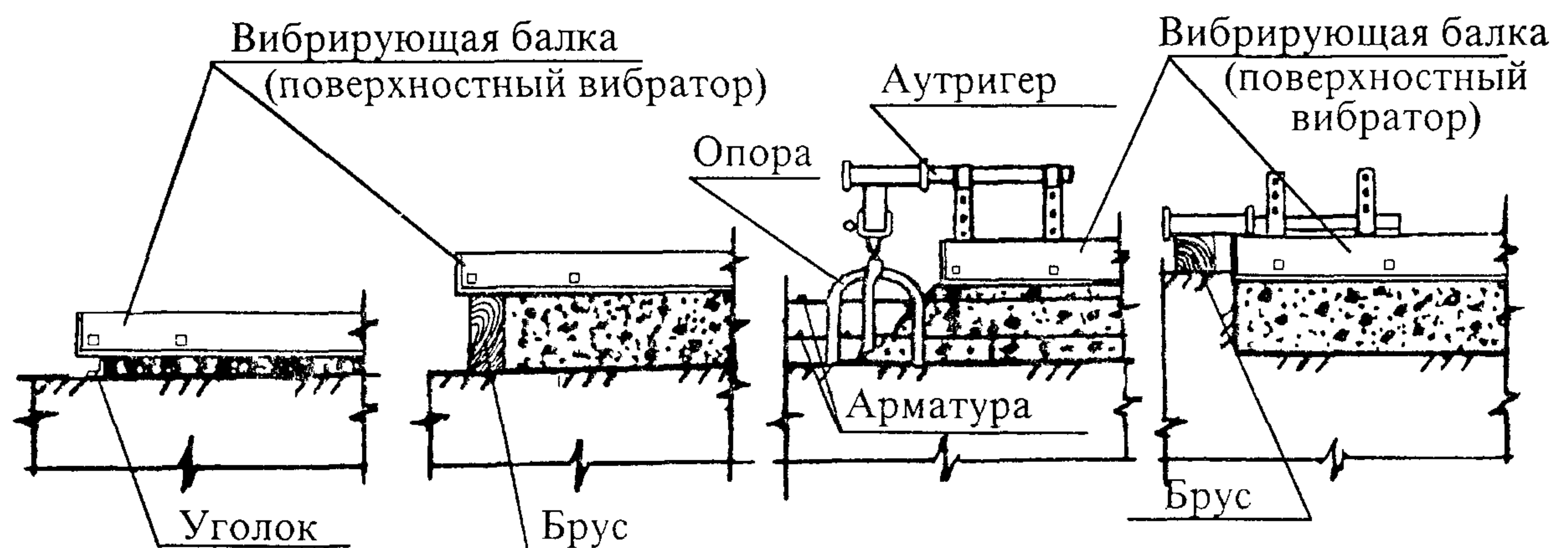
Рисунок 5 — Варианты установки опалубки и поддерживающих опор
