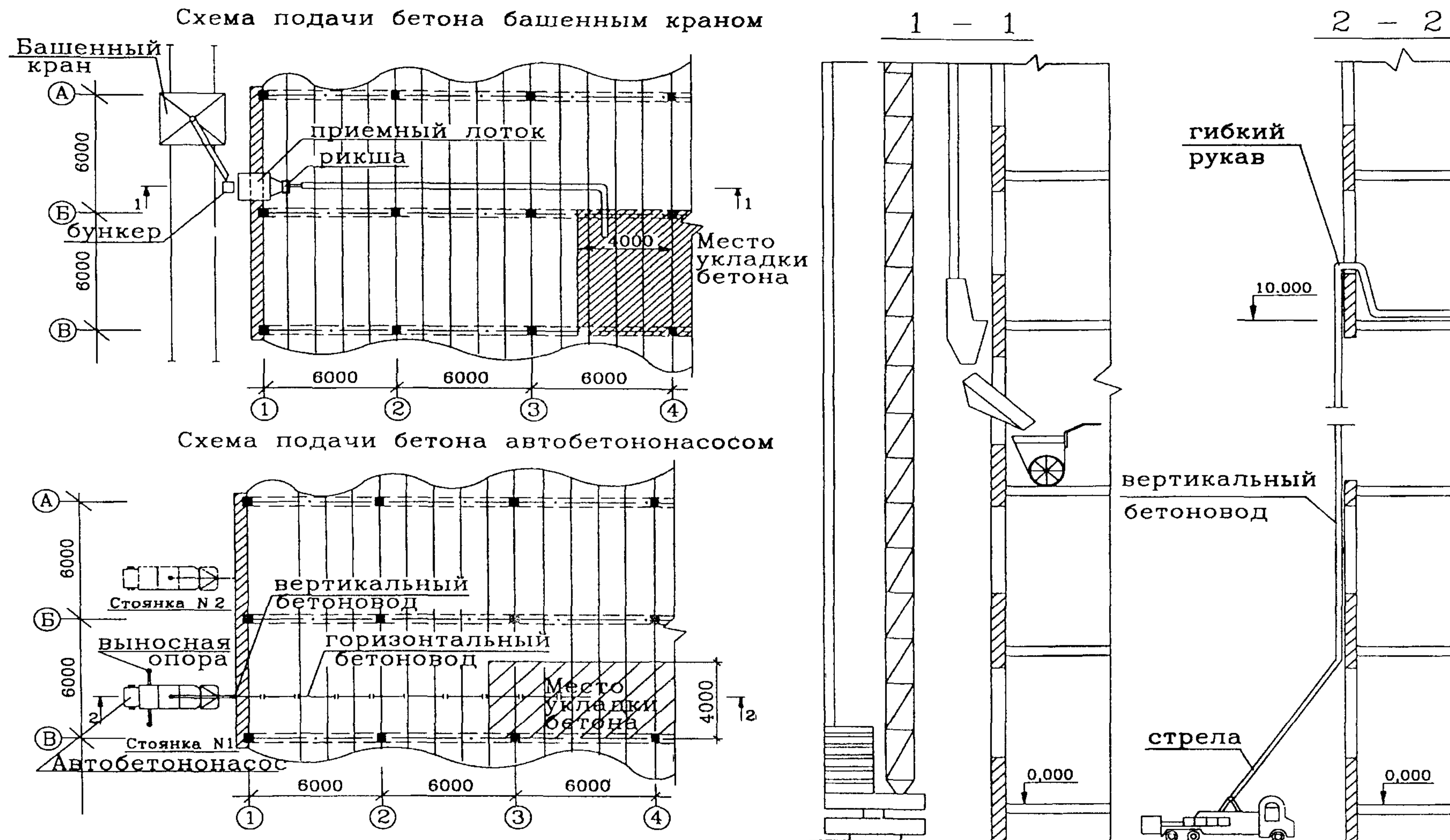
Рисунок 3 – Схема подачи бетона с помощью башенного крана и автобетононасоса
