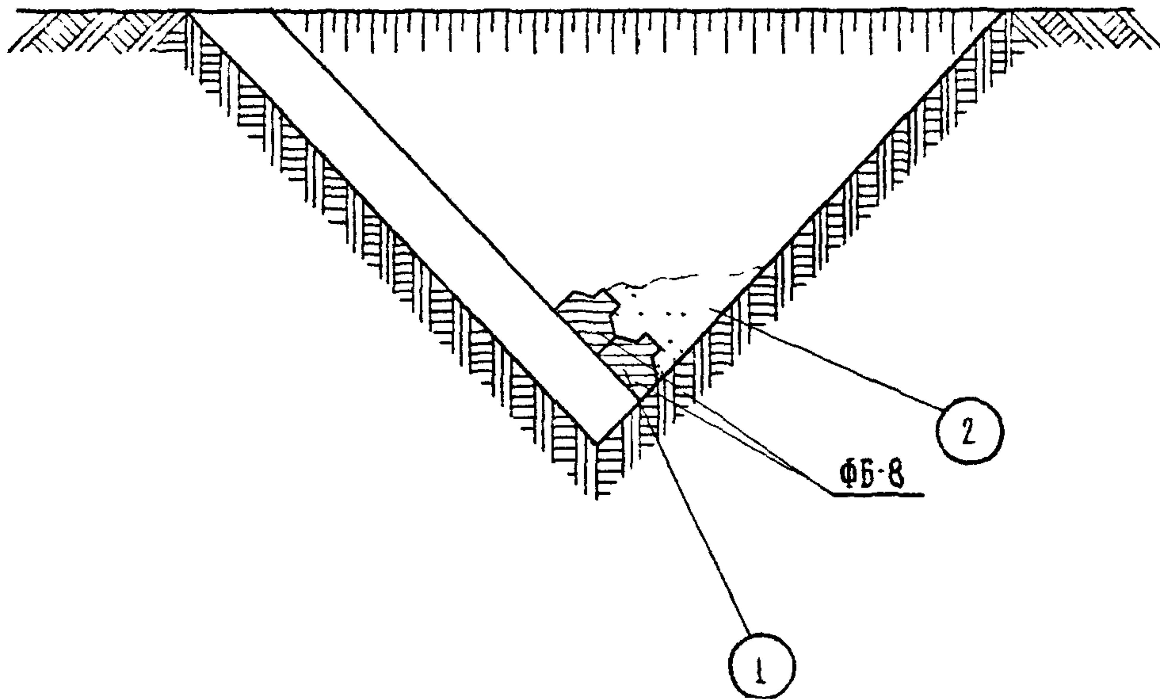
Рис.13. Последовательность монтажа анкерного фундамента. I этап
