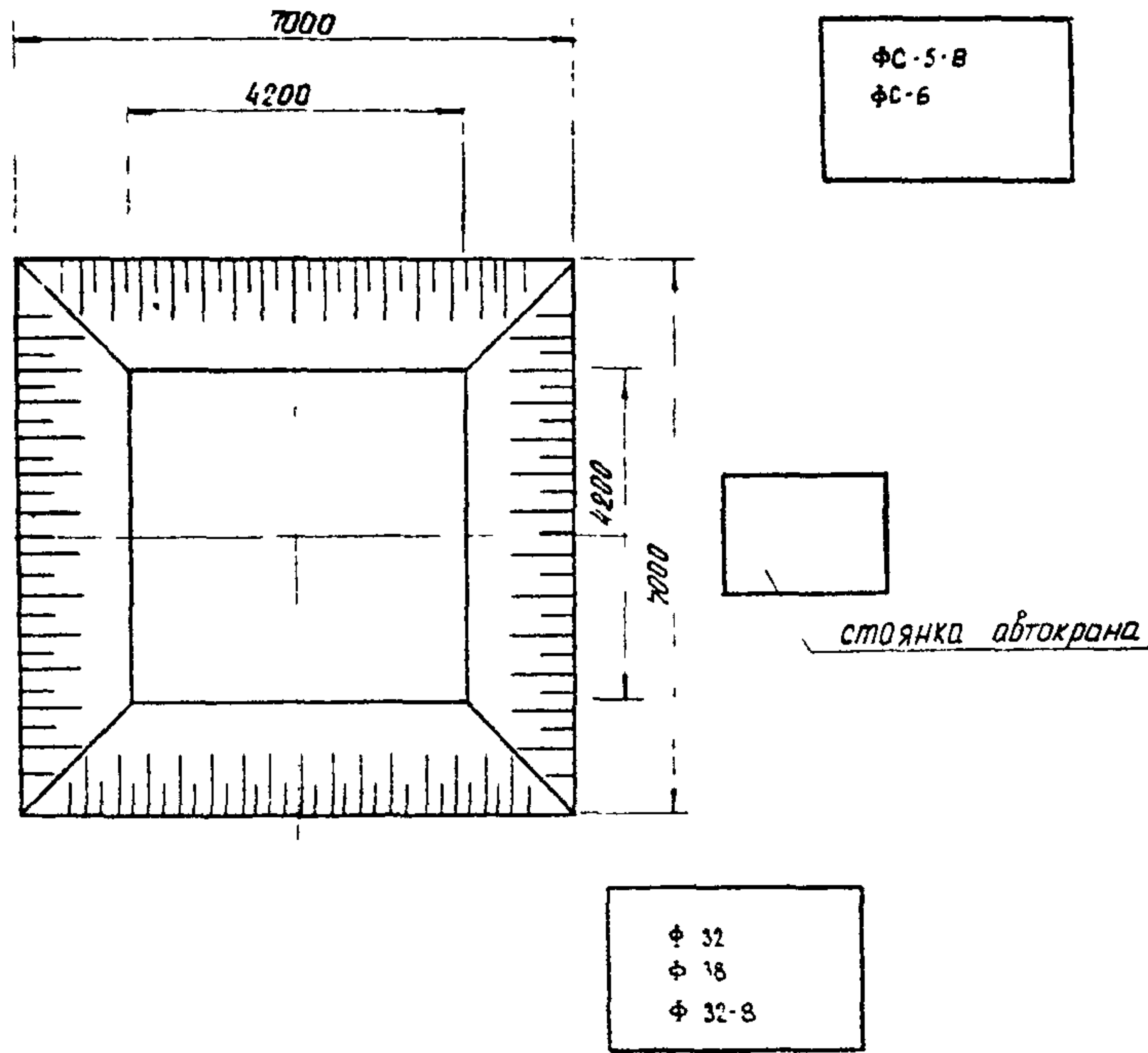
Рис.8. Размещение фундаментных блоков у котлована
