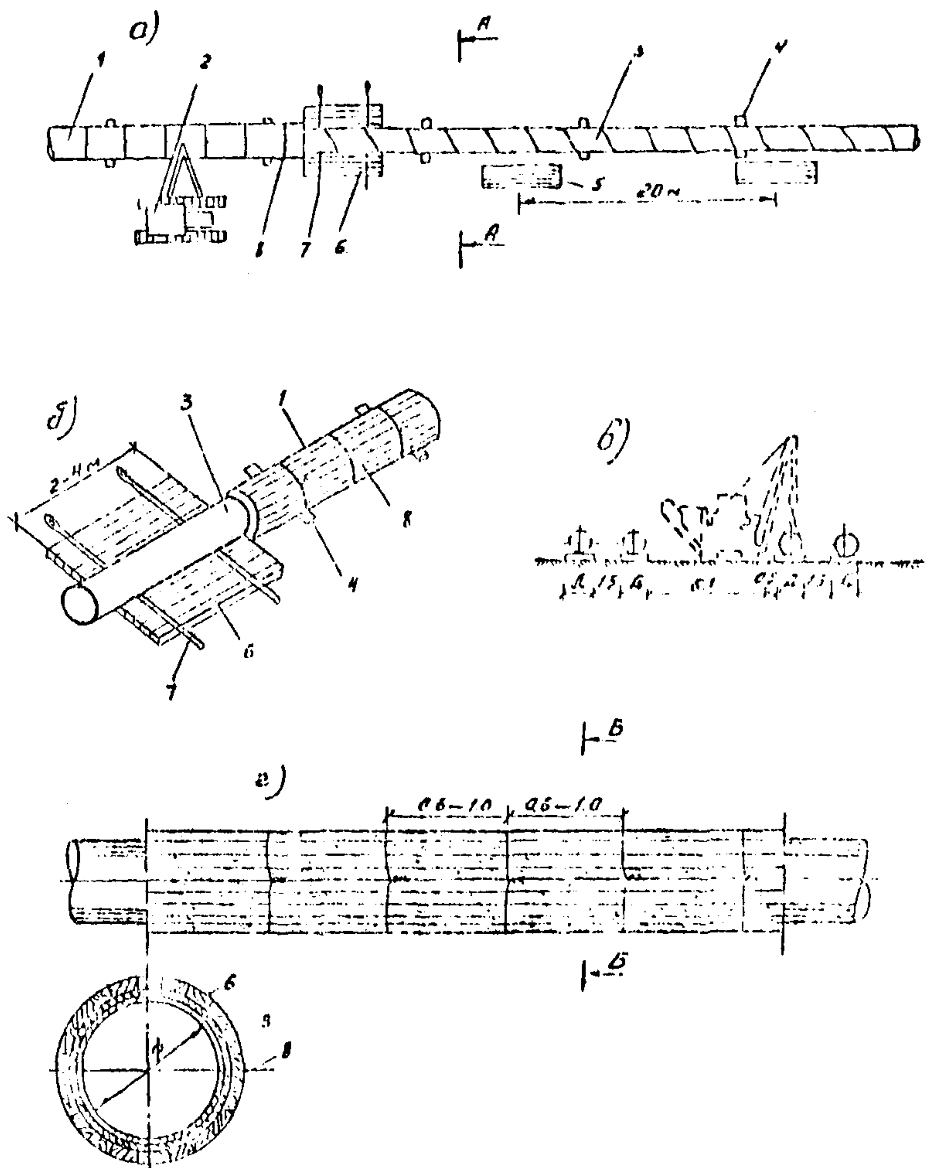
Рисунок. Схема футеровки трубопровода деревянными рейками. а- производство работ по футеровке одной плиты; б- футеровка трубопровода рейками с помощью двух поясов; в- футеровка нескольких плит; г- футерованный участок трубопровода. 1- футерованный участок трубопровода; 2- трубоукладчик Т 15-30; 3- заизолированный участок трубопровода; 4- лежки; 5- пакет футеровочной рейки; 6- футеровочная рейка; 7- переносные пояса; 8- проволочная скрутка.
