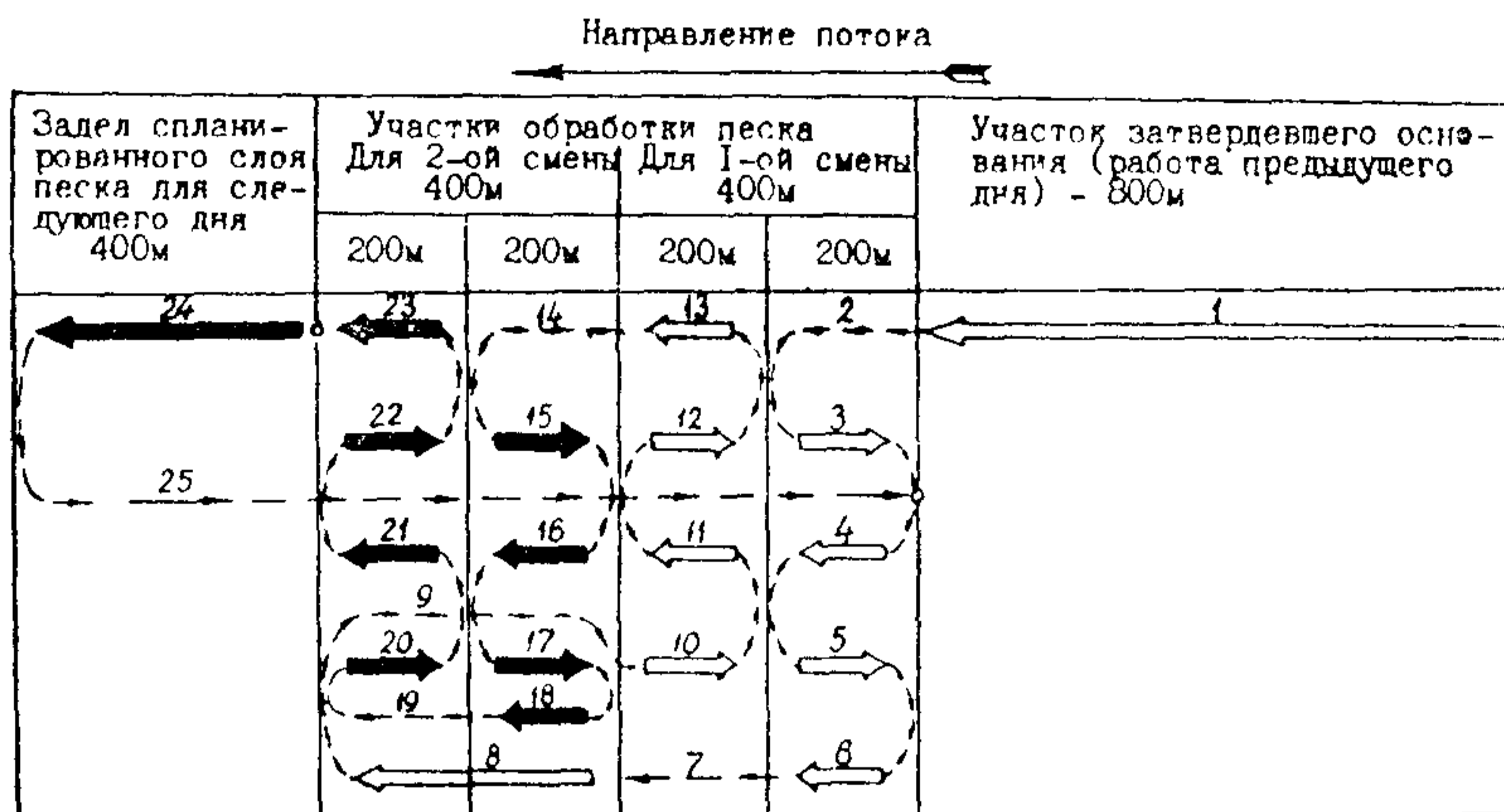
Рис. 5. Схема проходов профилировщика TS-425.
