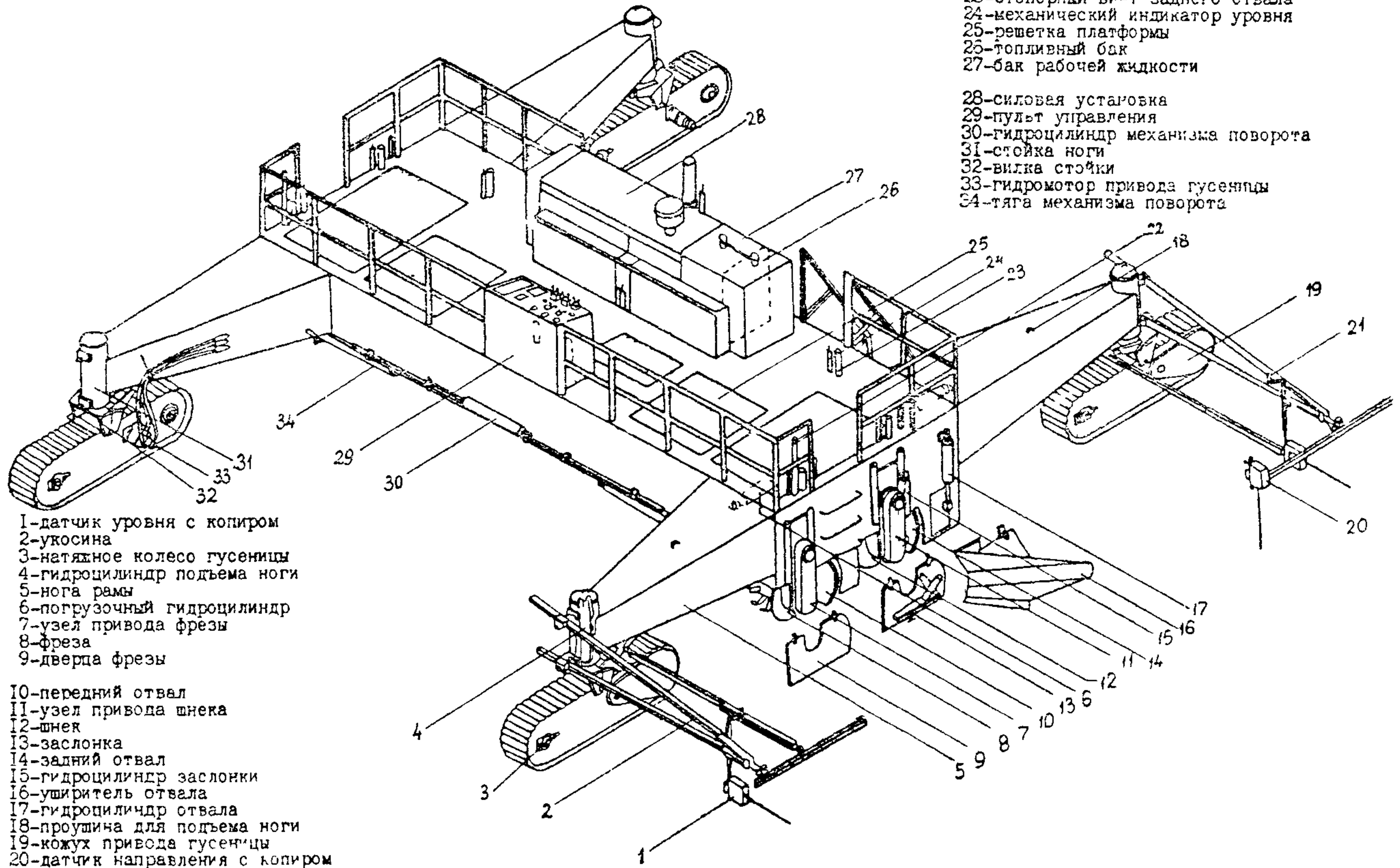
Рис. 1 Основные части профилировщика TS-425:
