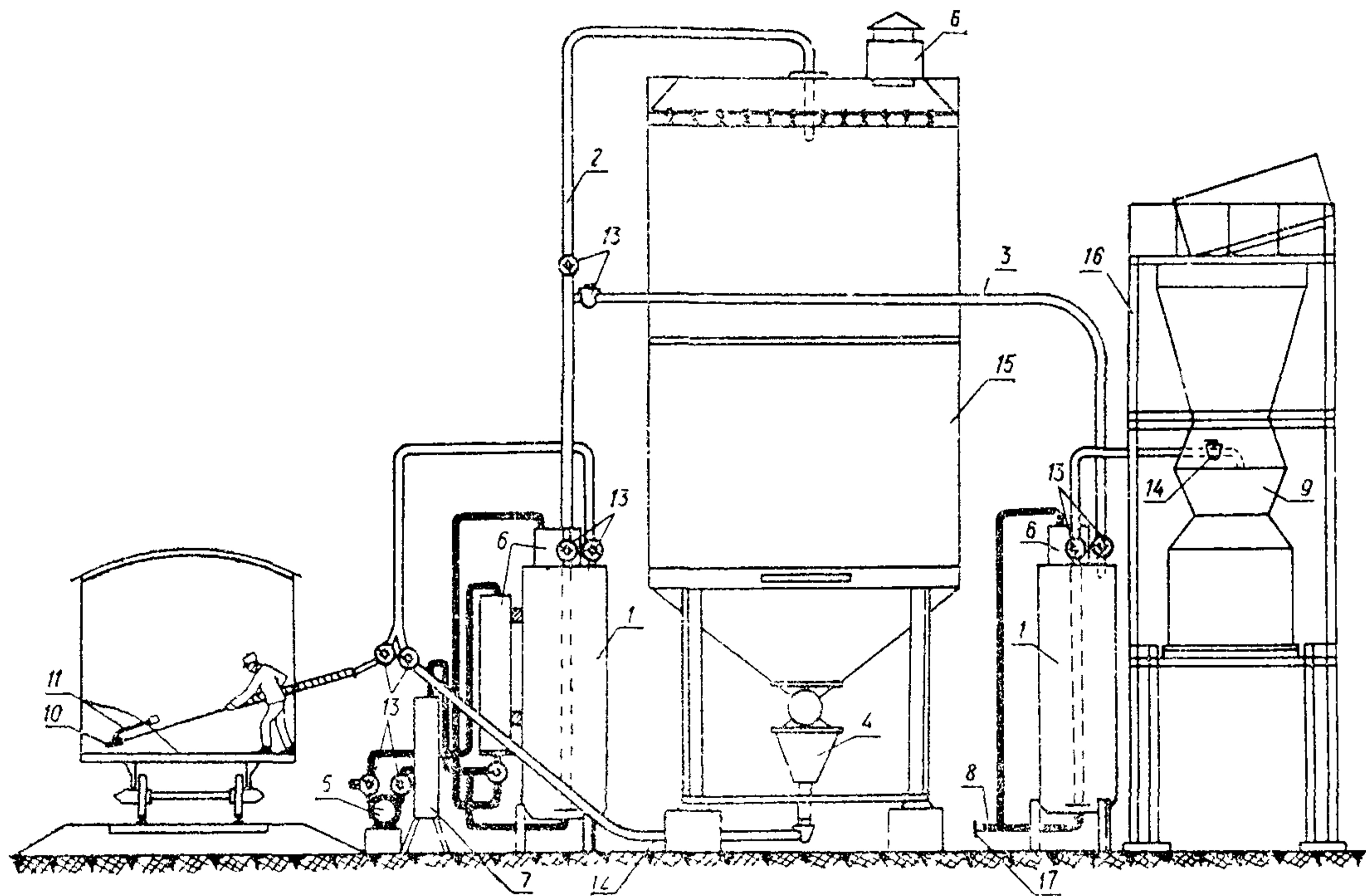
Рис 2 Технологическая схема работы монжусов на АБЗ.
