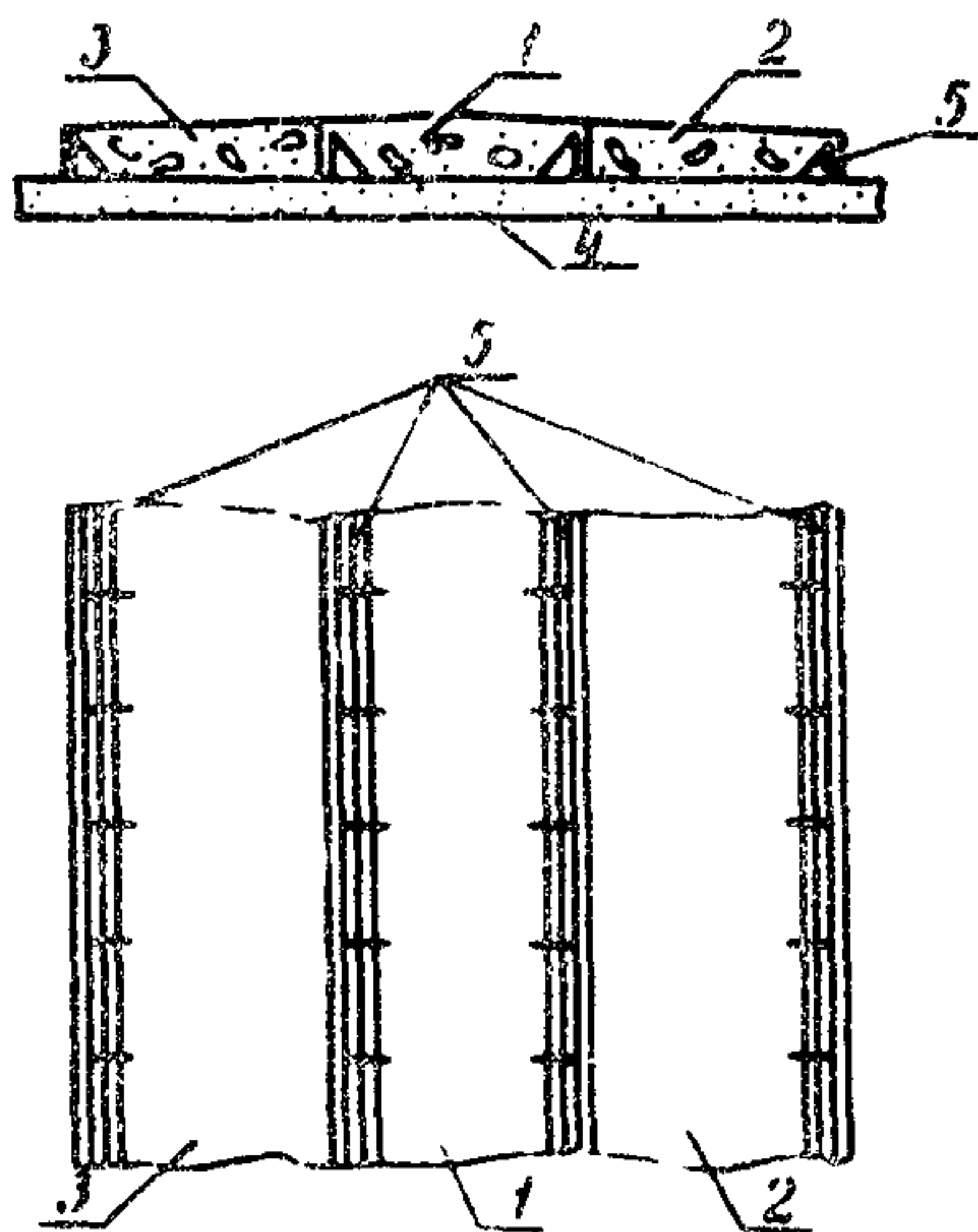
Рис.2. Схема многополосного покрытия, бетонизируемого в скользящих формах:
