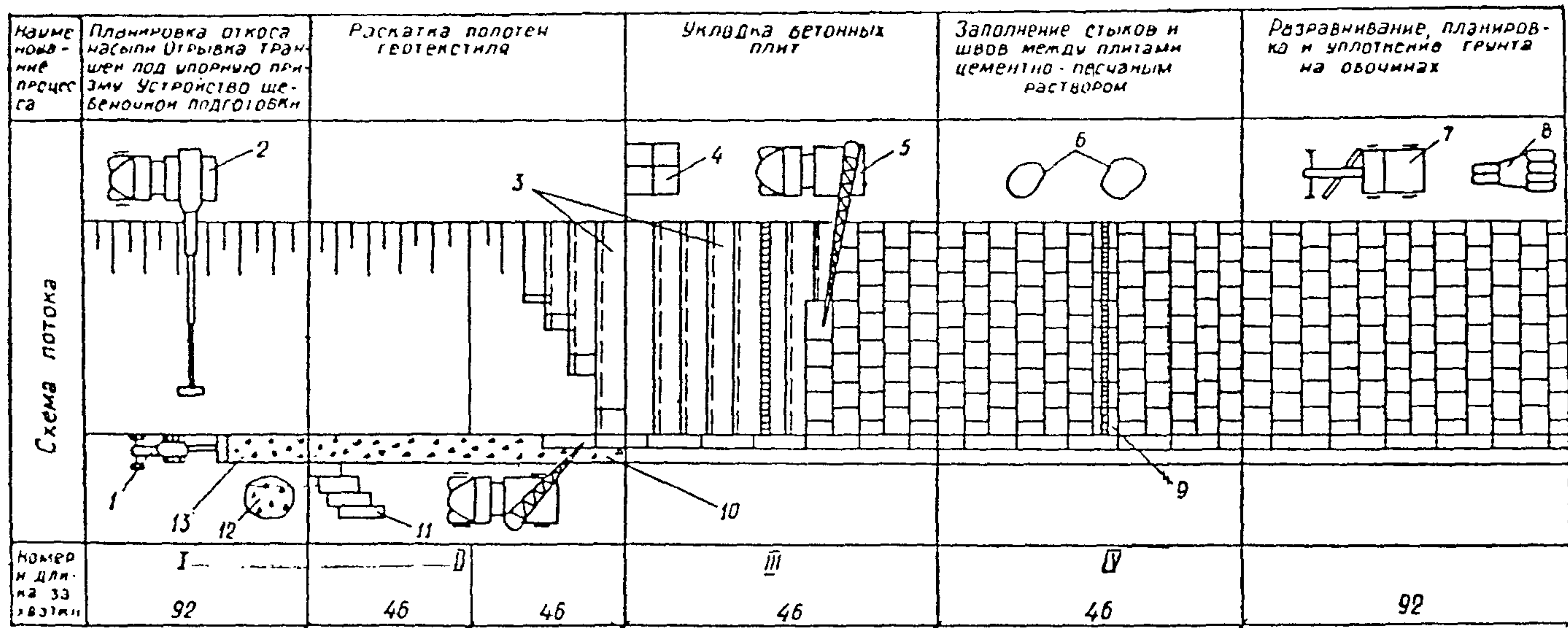
Рис. 1. Технологическая схема выполнения работ по укреплению откоса насыпи бетонными плитами: 1—экскаватор ЭО-2623; 2—экскаватор-планировщик ЭО-3332А; 3—полотна геотекстиля; 4—штабеля плит; 5—автокран КТС-3Г; 6—емкости для цементно-песчаного раствора; 7—автогрейдер ДЗ-48А; 8—каток на пневмошинах ДУ-16Г; 9—переносный трап; 10—щебеночная подготовка; 11—разложенные блоки упорной призмы; 12—щебень для устройства щебеночной подготовки; 13—траншея под упорную призму
