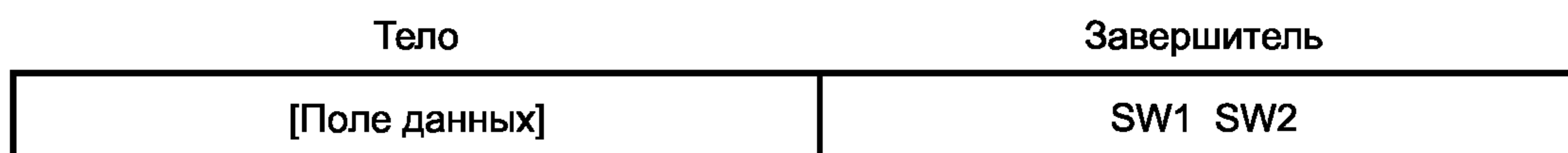
Рисунок 6 — Структура ответного APDU
