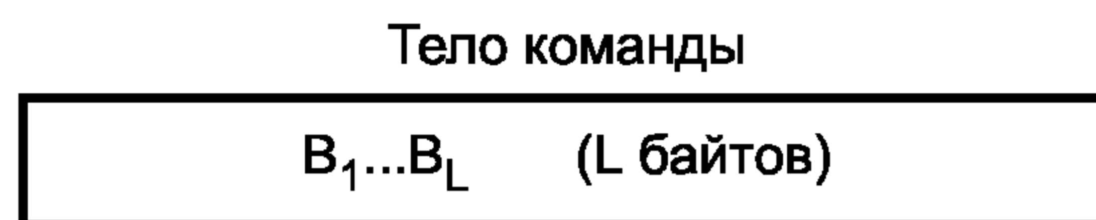
Рисунок 5 — Непустое тело
