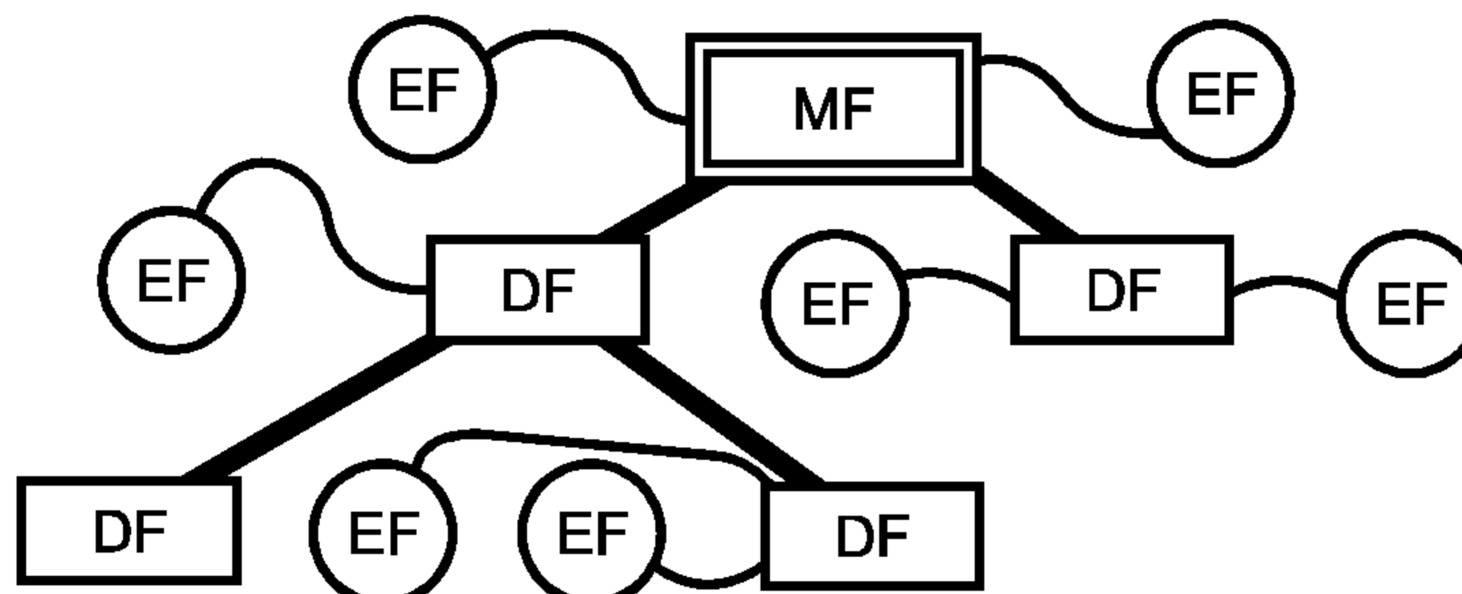
Рисунок 1 — Пример логической организации файлов
