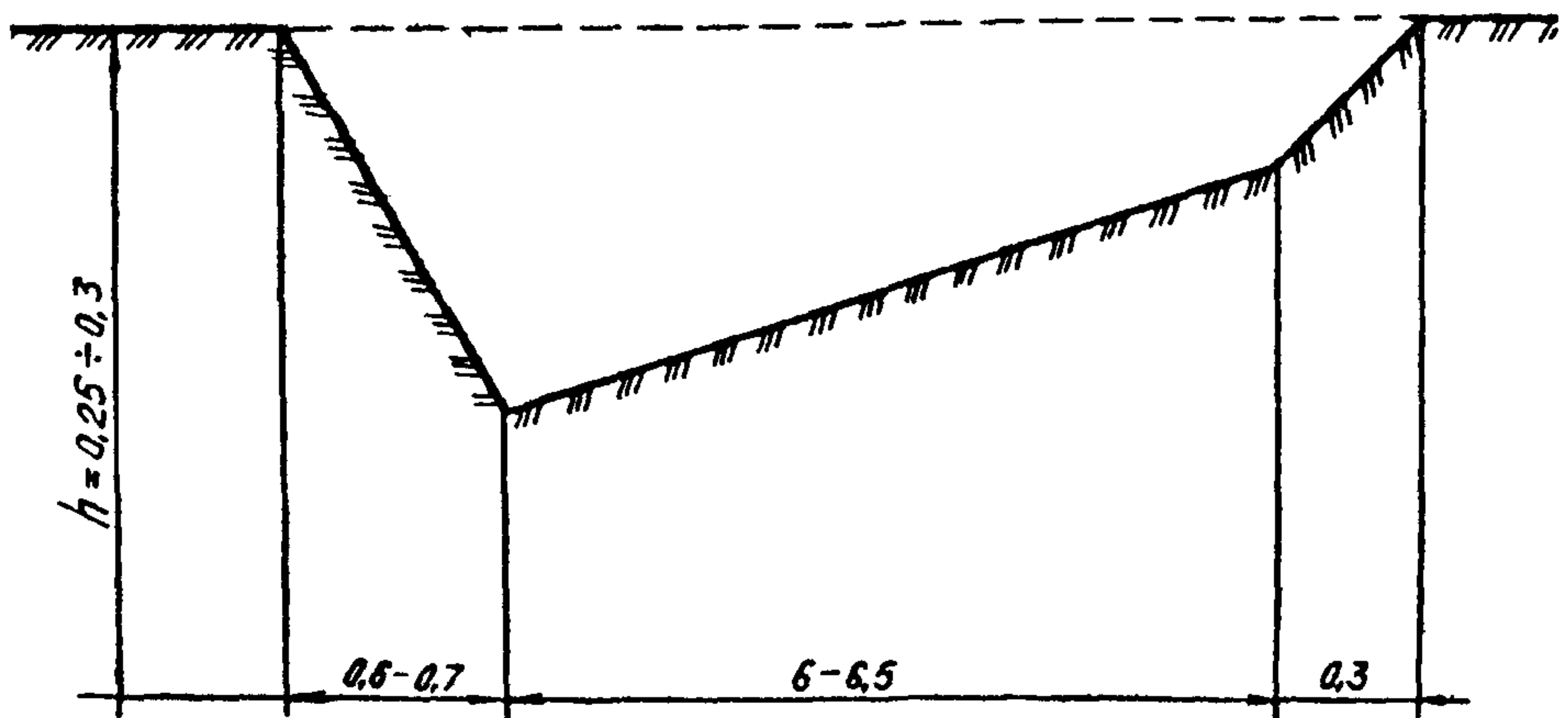
Рис. 4. Клиновая схема зарезания грунта
