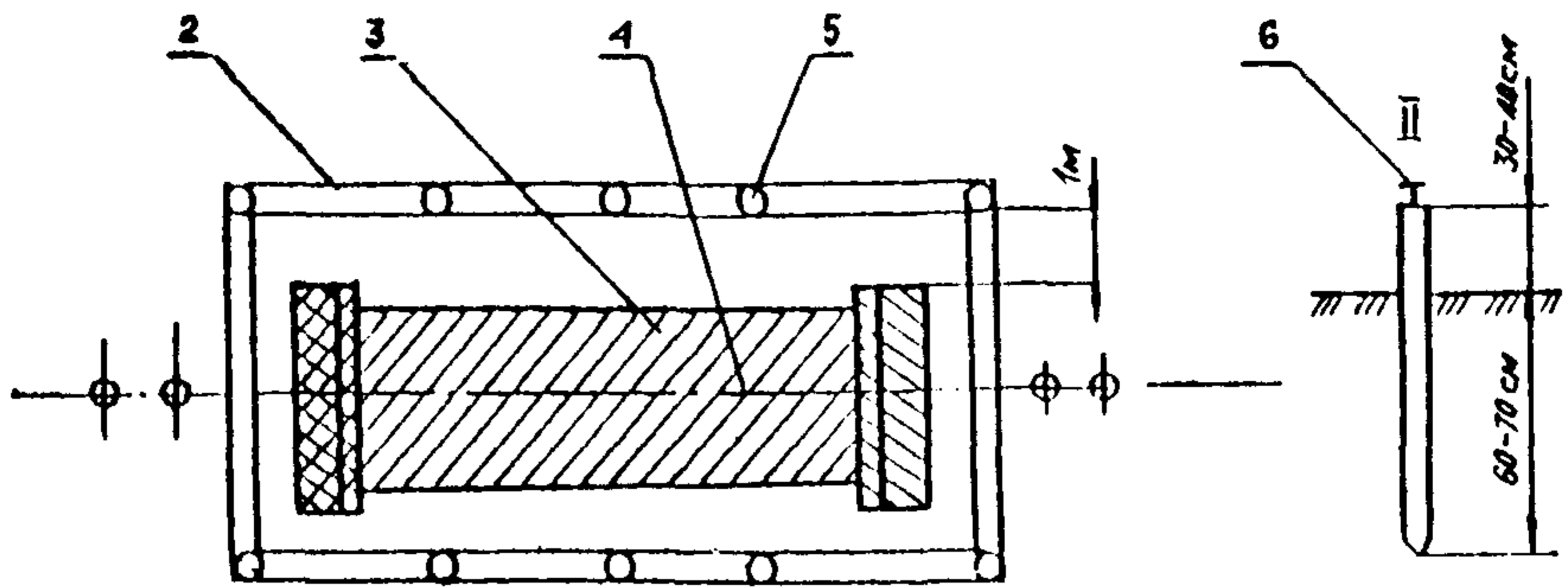
Рис. 2. Схема разбивки котлована трубы:
