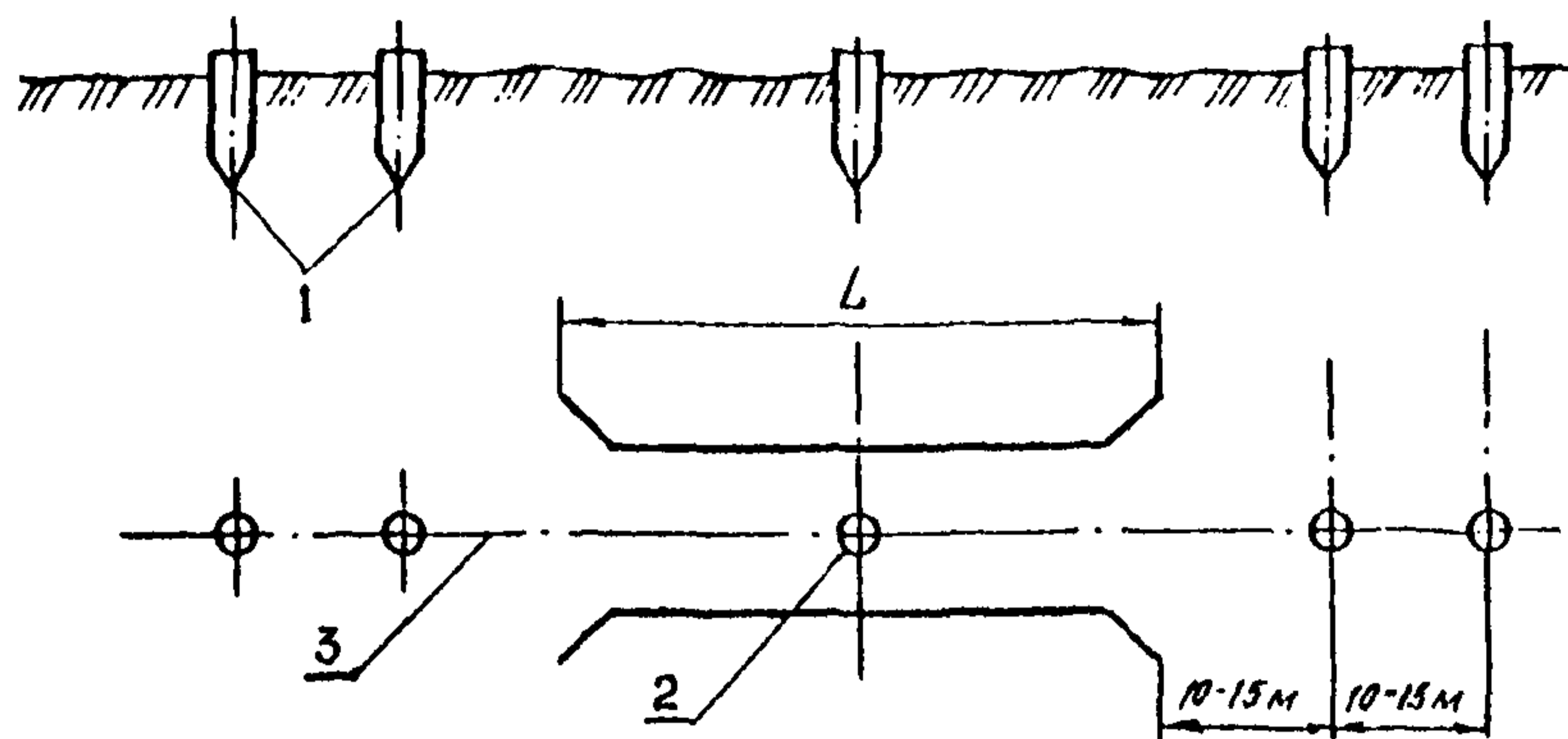
Рис. 1. Схема закрепления местоположения трубы на трассе: 1 – выносные столбы; 2 – точка и сторожек с надписью «ось», «пикет», «плюс»; 3 – продольная ось трубы; L – длина трубы
