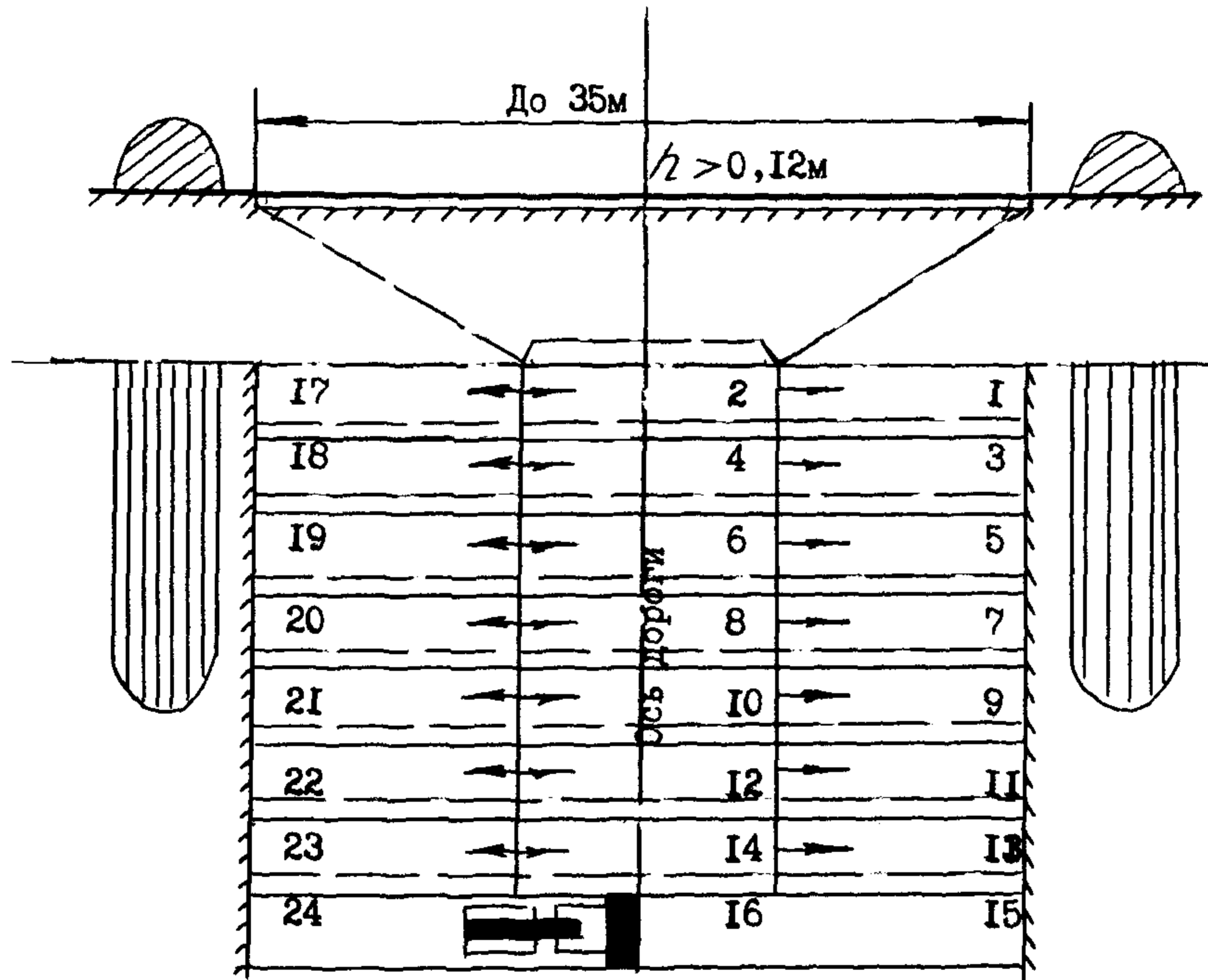
Поперечно-участковая схема срезки растительного слоя грунта.
