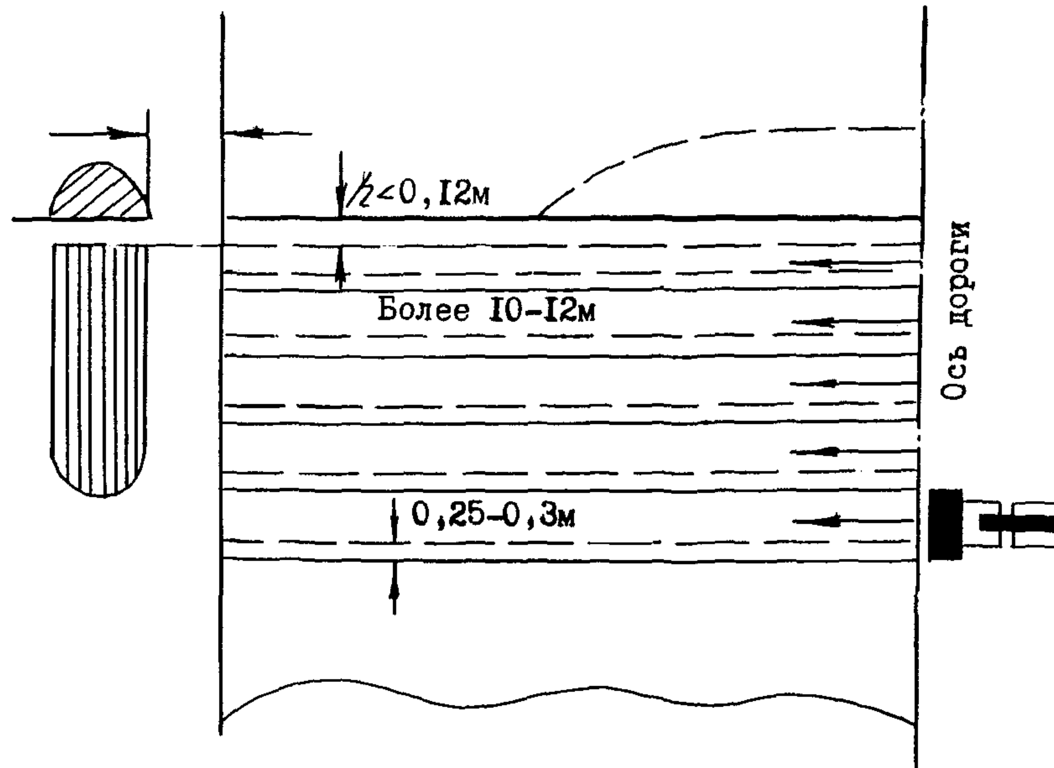
Поперечная схема срезки растительного слоя грунта.
