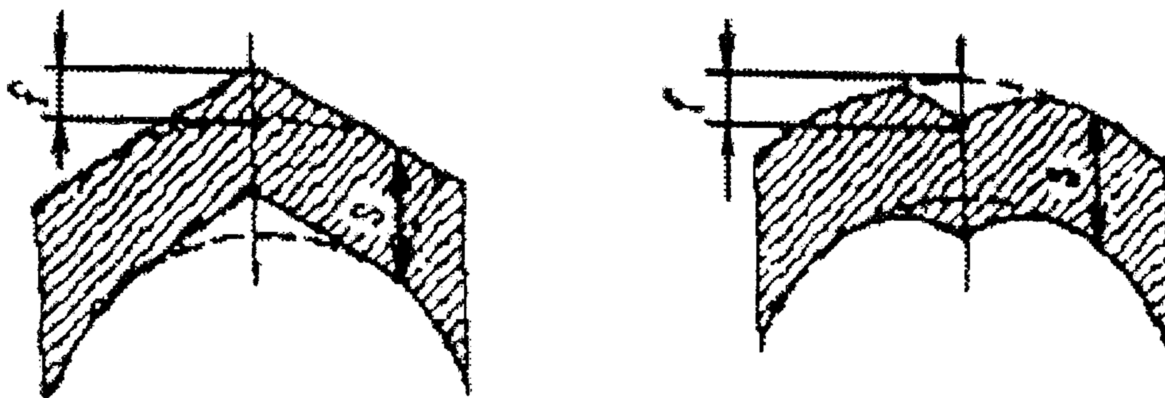
Рис. 1. Увод (угловатость) кромок в сварных швах
