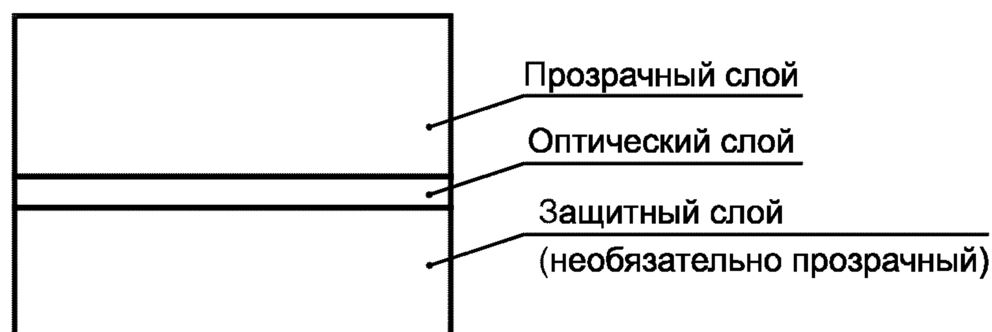
Рисунок 1 — Поперечное сечение карты в оптической зоне
