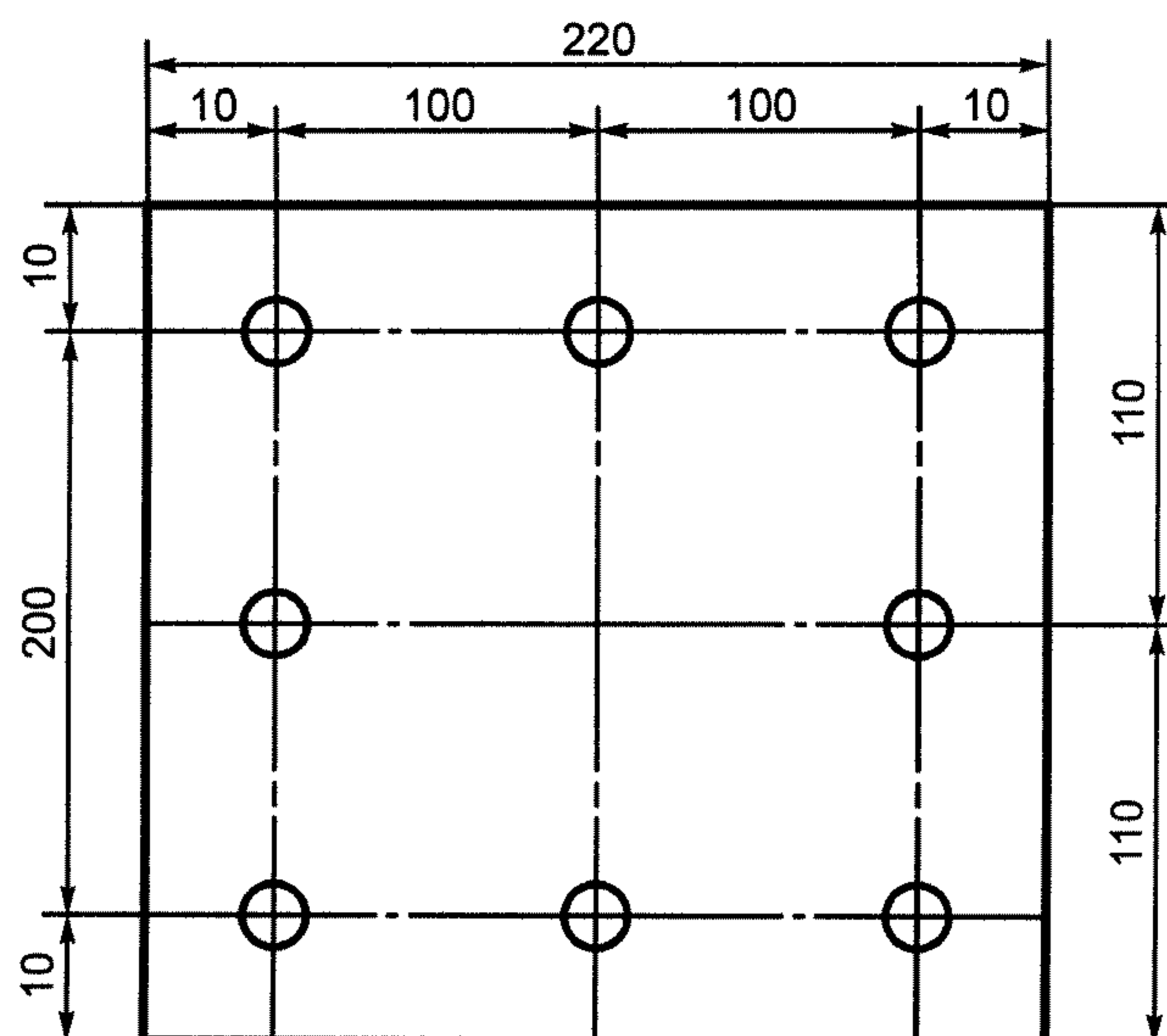
Рисунок 1 — Шаблон для нанесения меток на пробу
