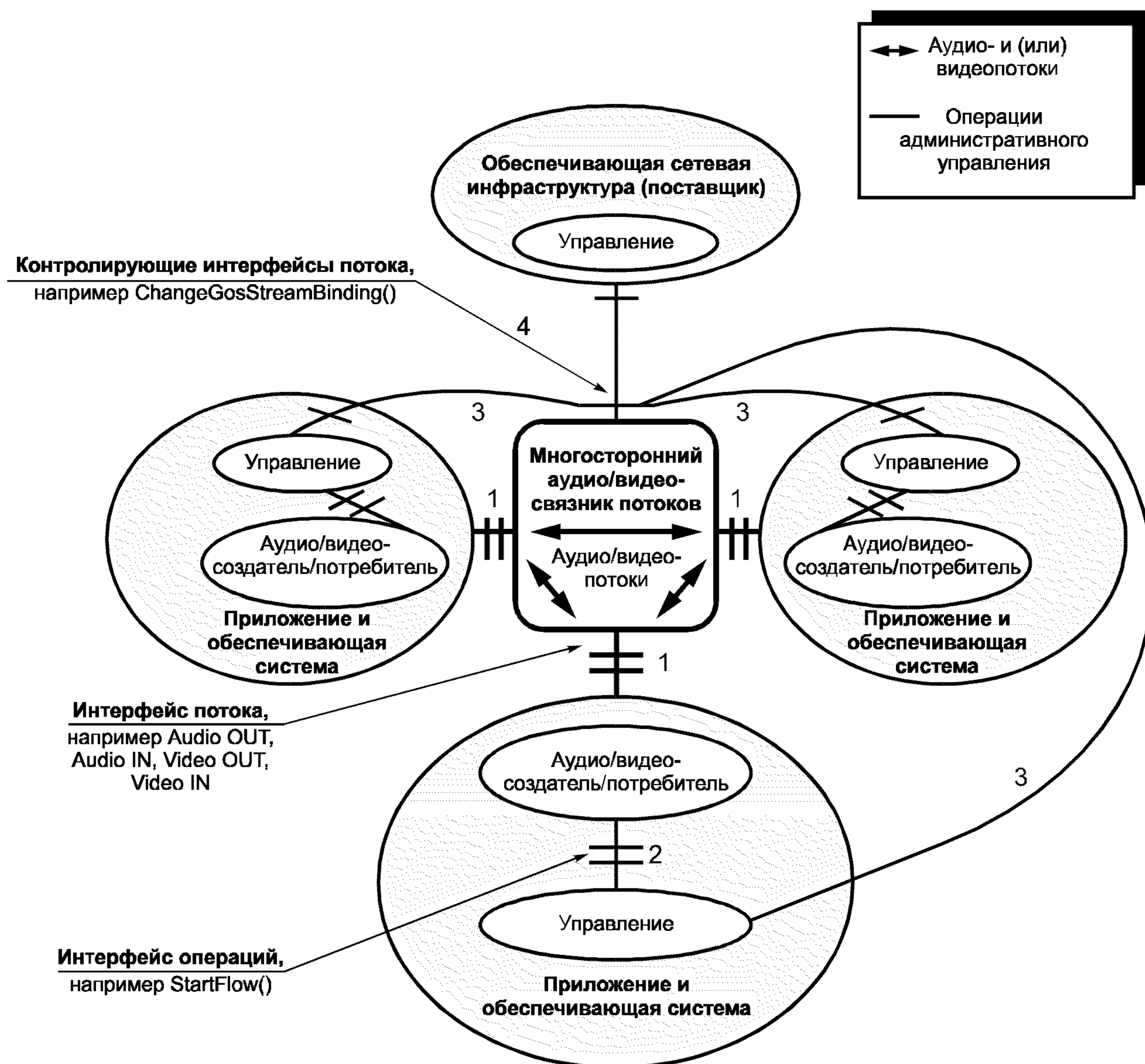
Рисунок 30 — Многостороннее связывание аудио/видеопотоков
