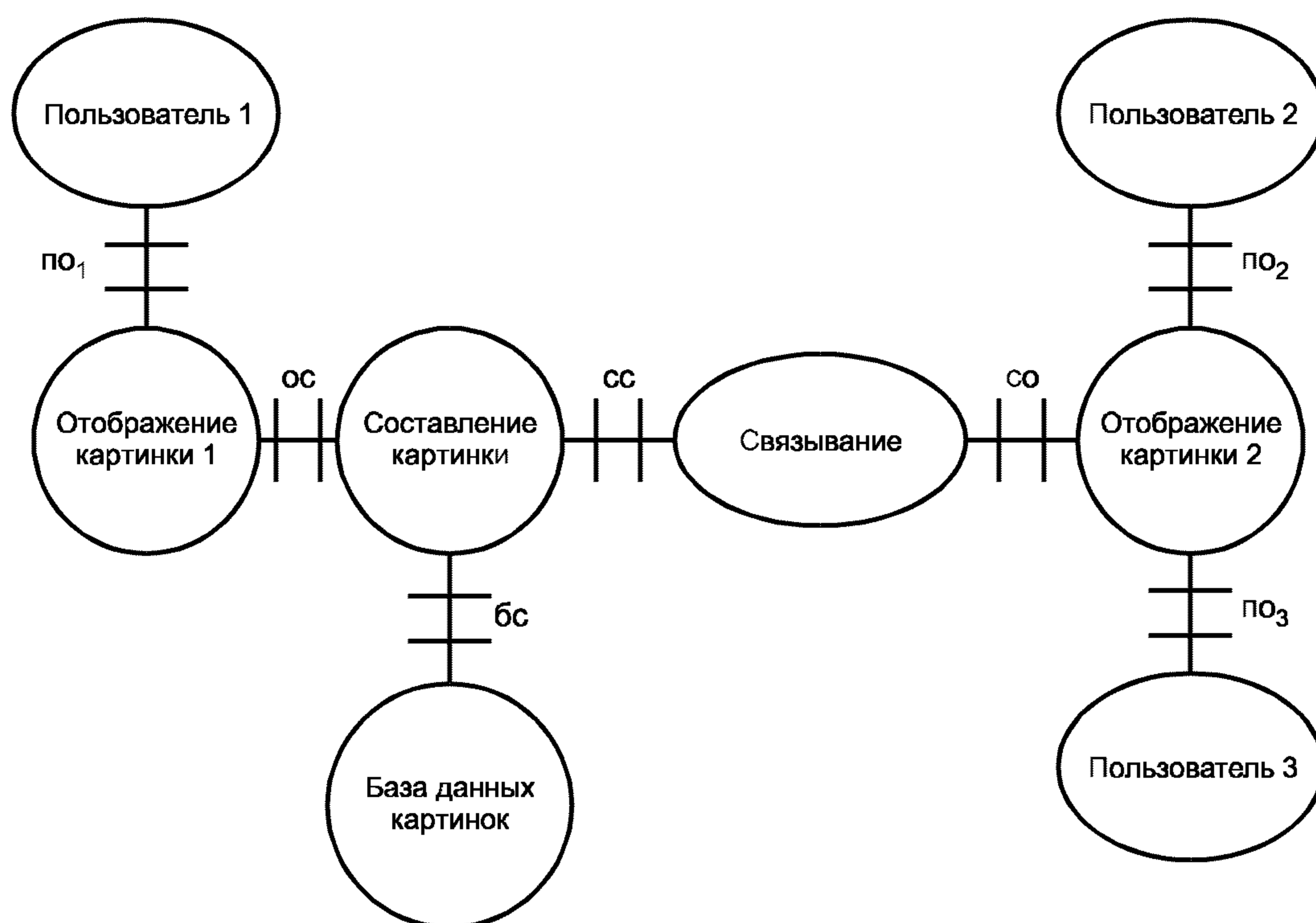
Рисунок 18 — Вычислительная точка зрения
