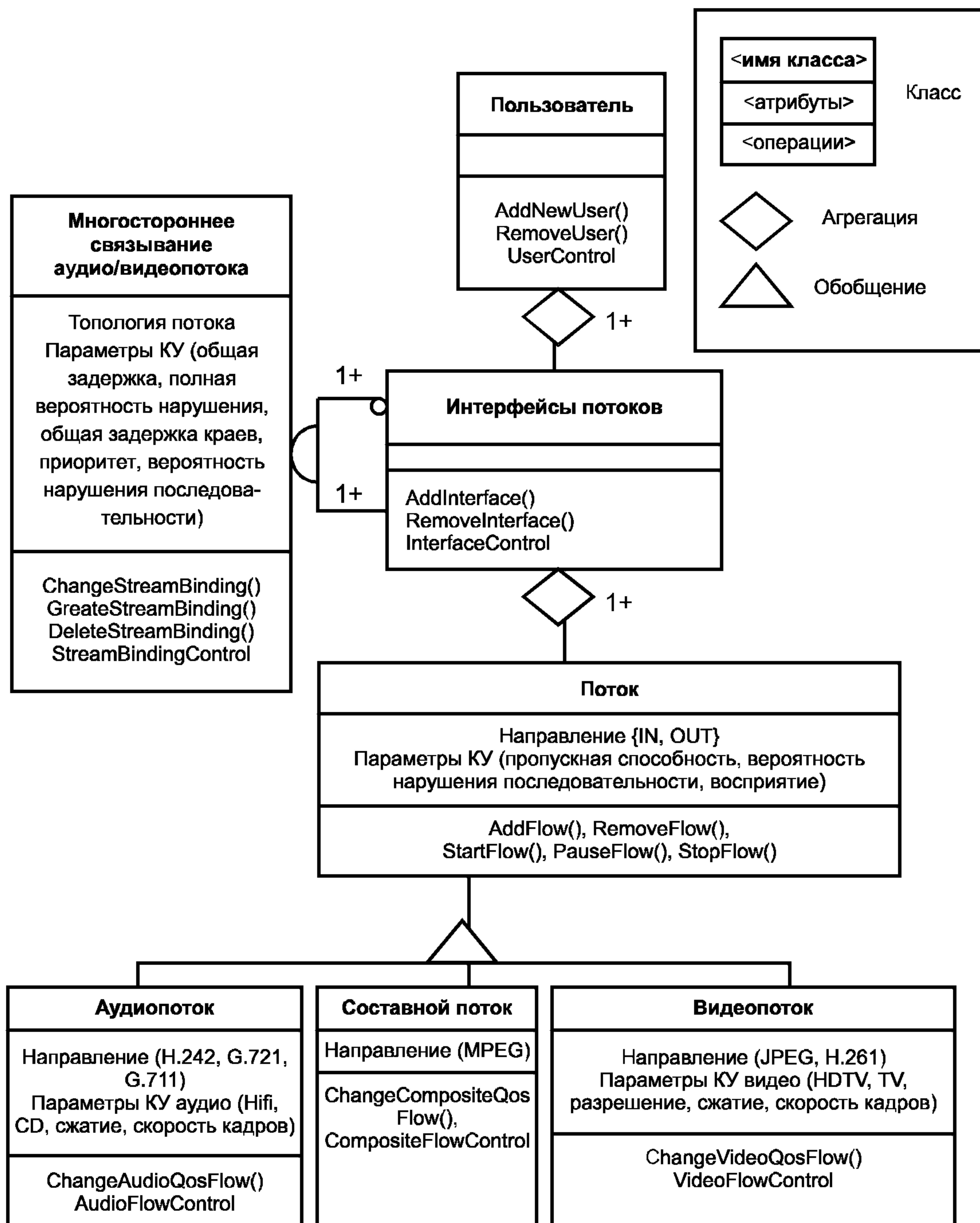
Рисунок 32 — Инвариантная схема связывающего контракта
