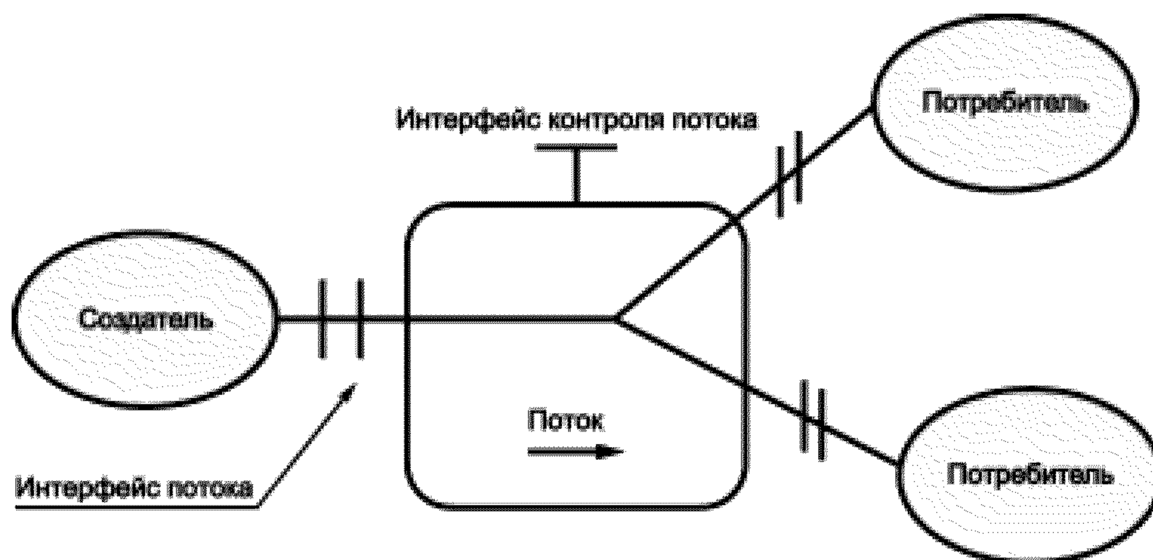
Рисунок 26 — Представление явного связывания (для потока)
