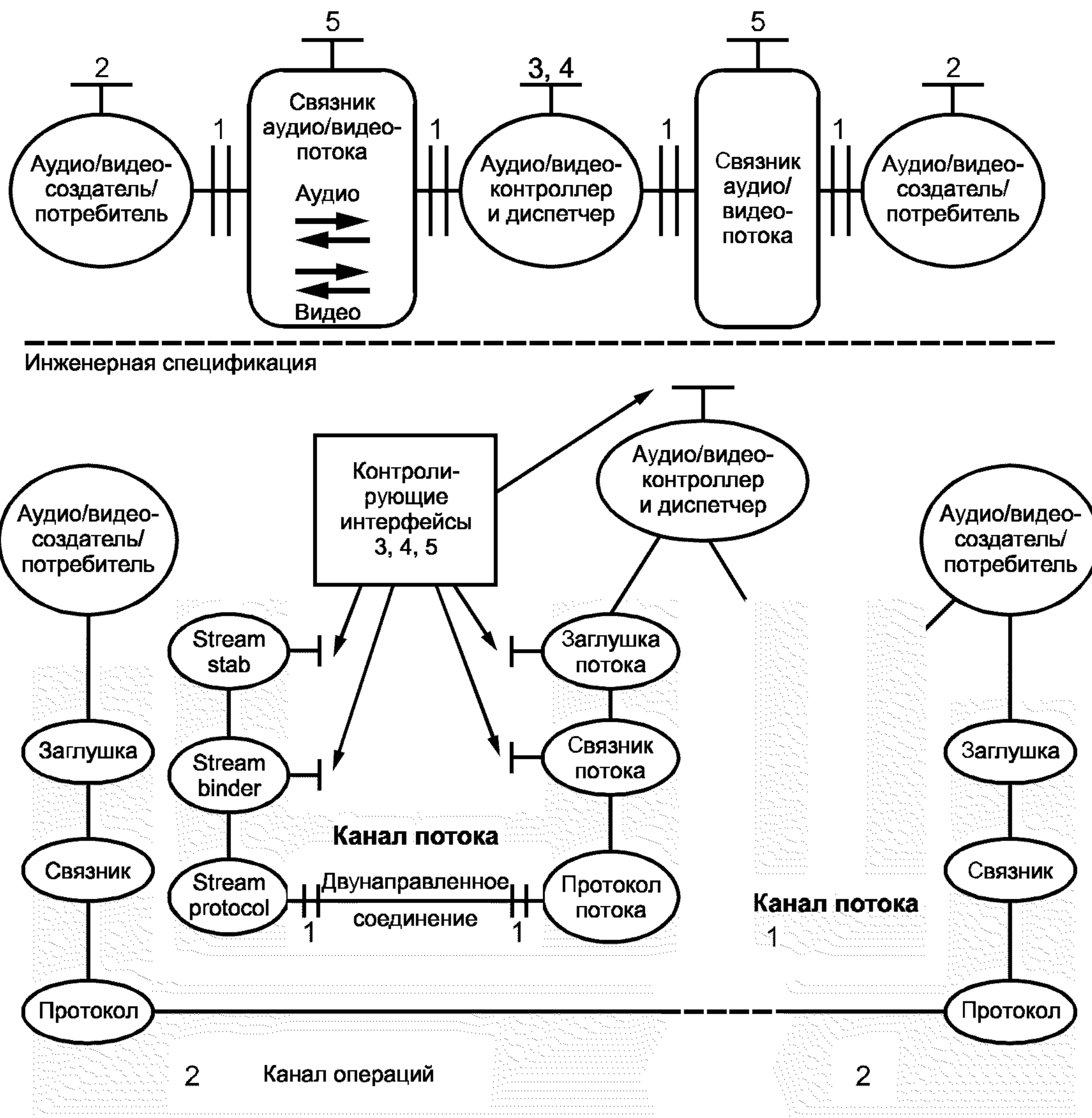
Рисунок 35 — Отображение вычислительной спецификации в инженерную
