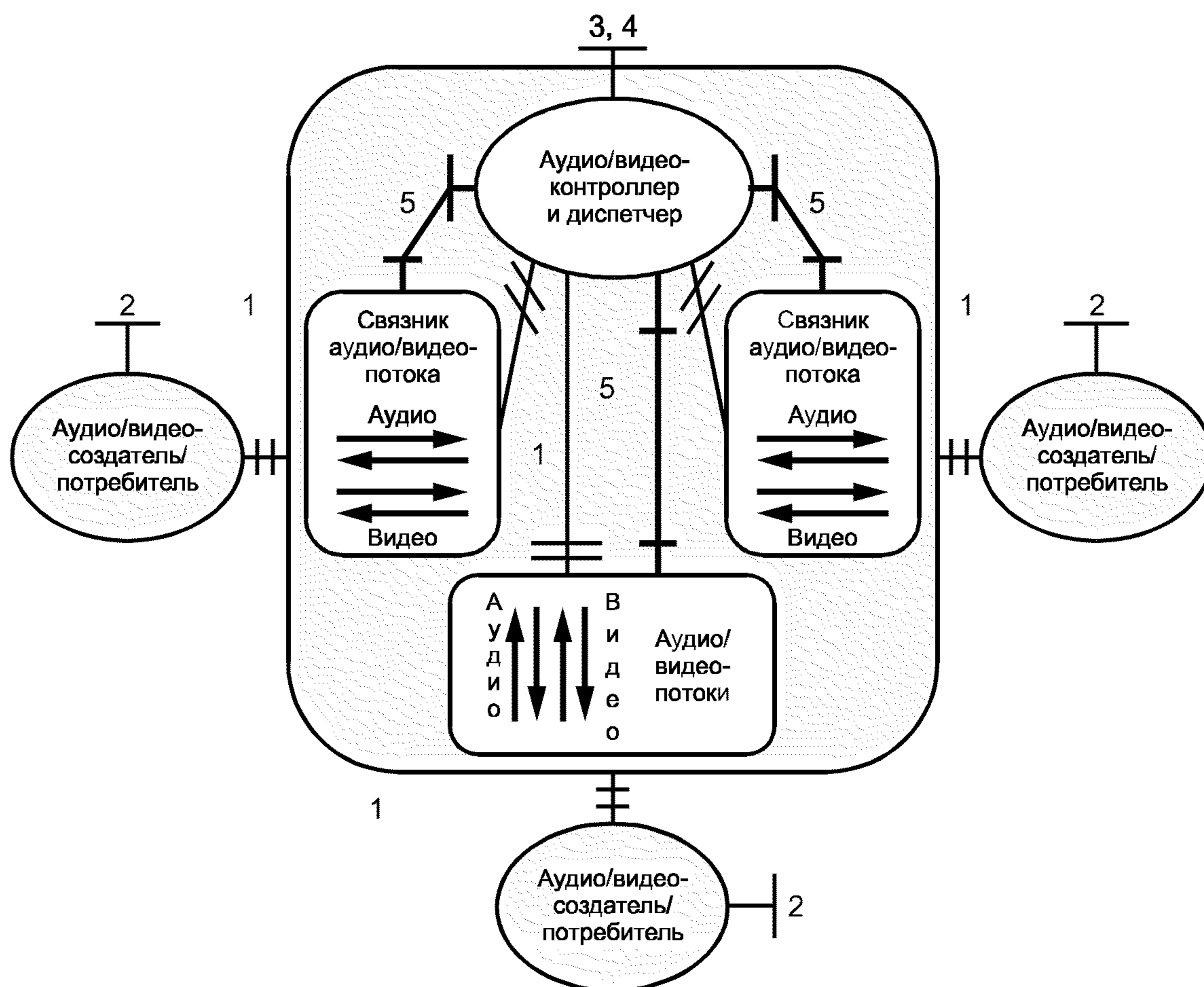
Рисунок 34 — Объекты, участвующие в многостороннем аудио/видеообмене
