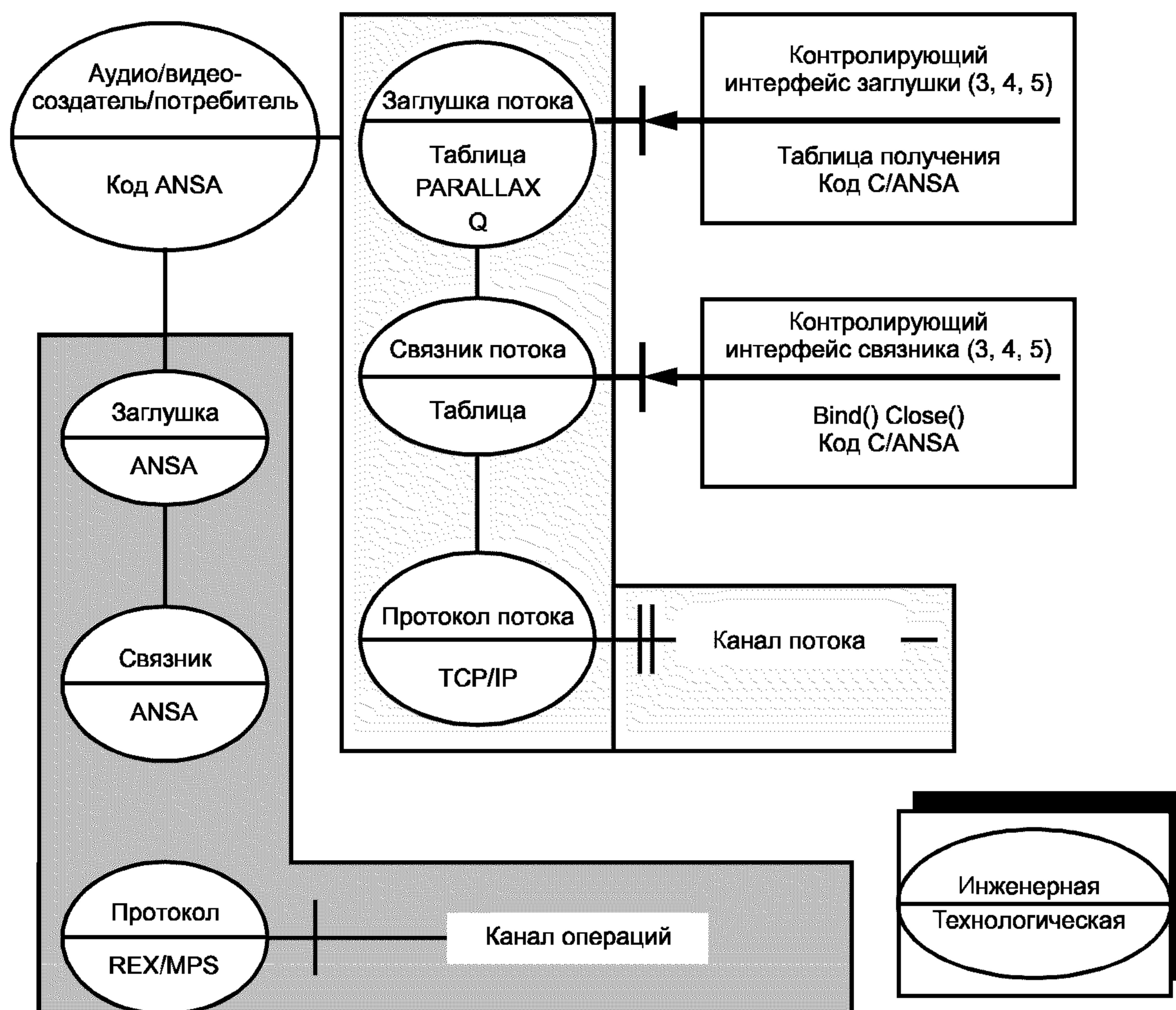
Рисунок 36 — Отображение инженерной спецификации в технологическую
