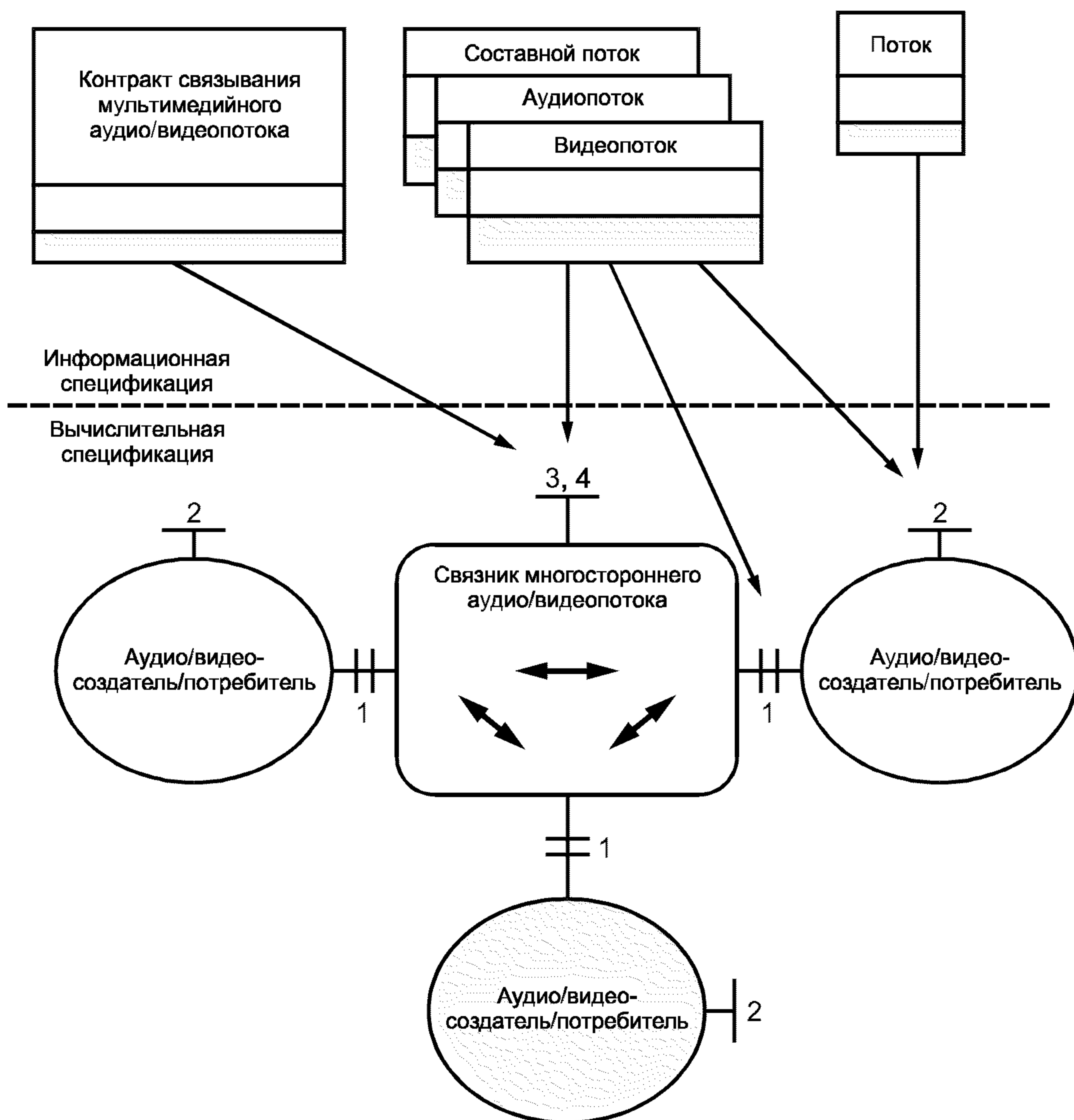
Рисунок 33 — Отображение информационной спецификации в вычислительную
