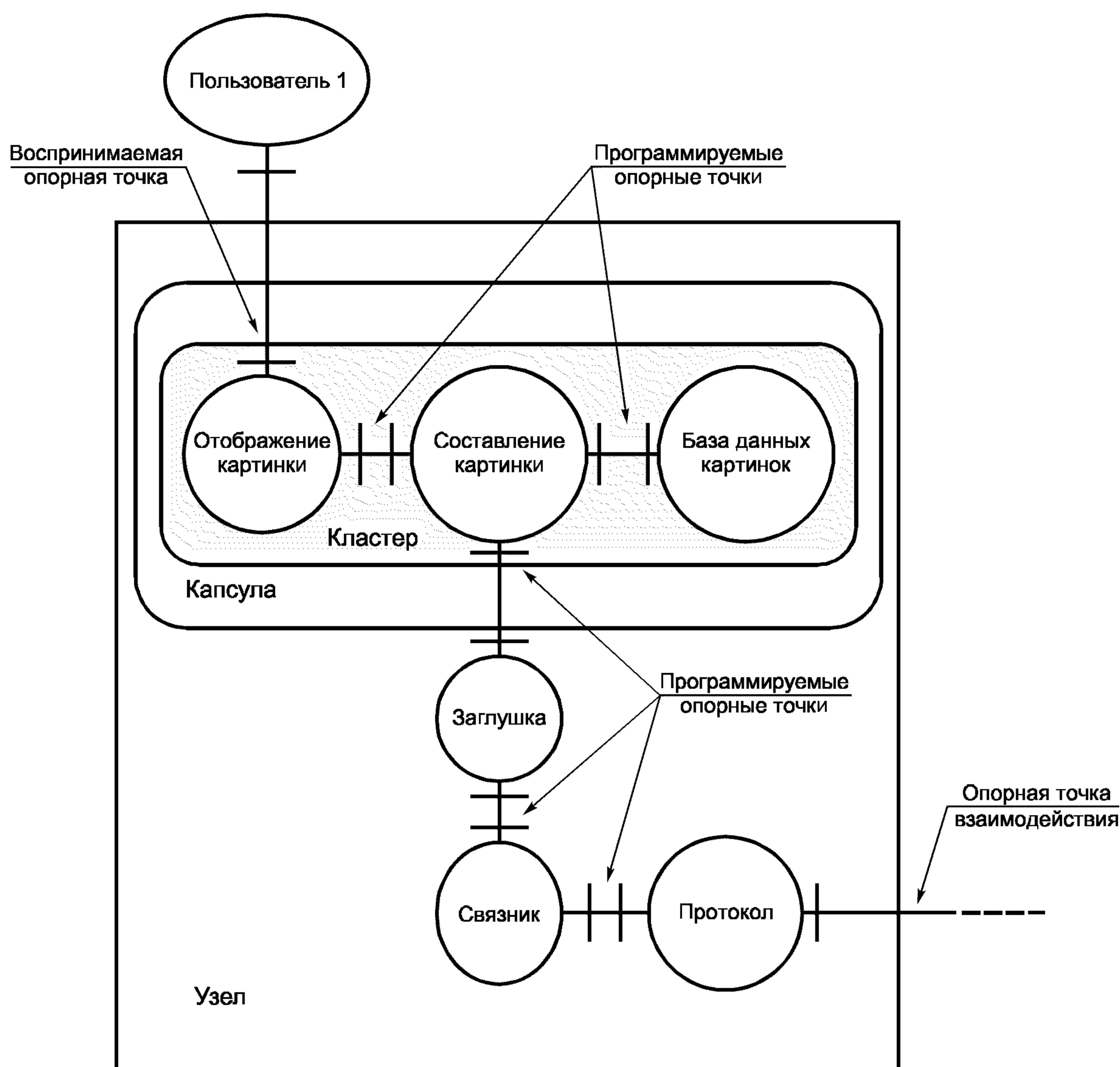
Рисунок 19 — Инженерная точка зрения (часть)
