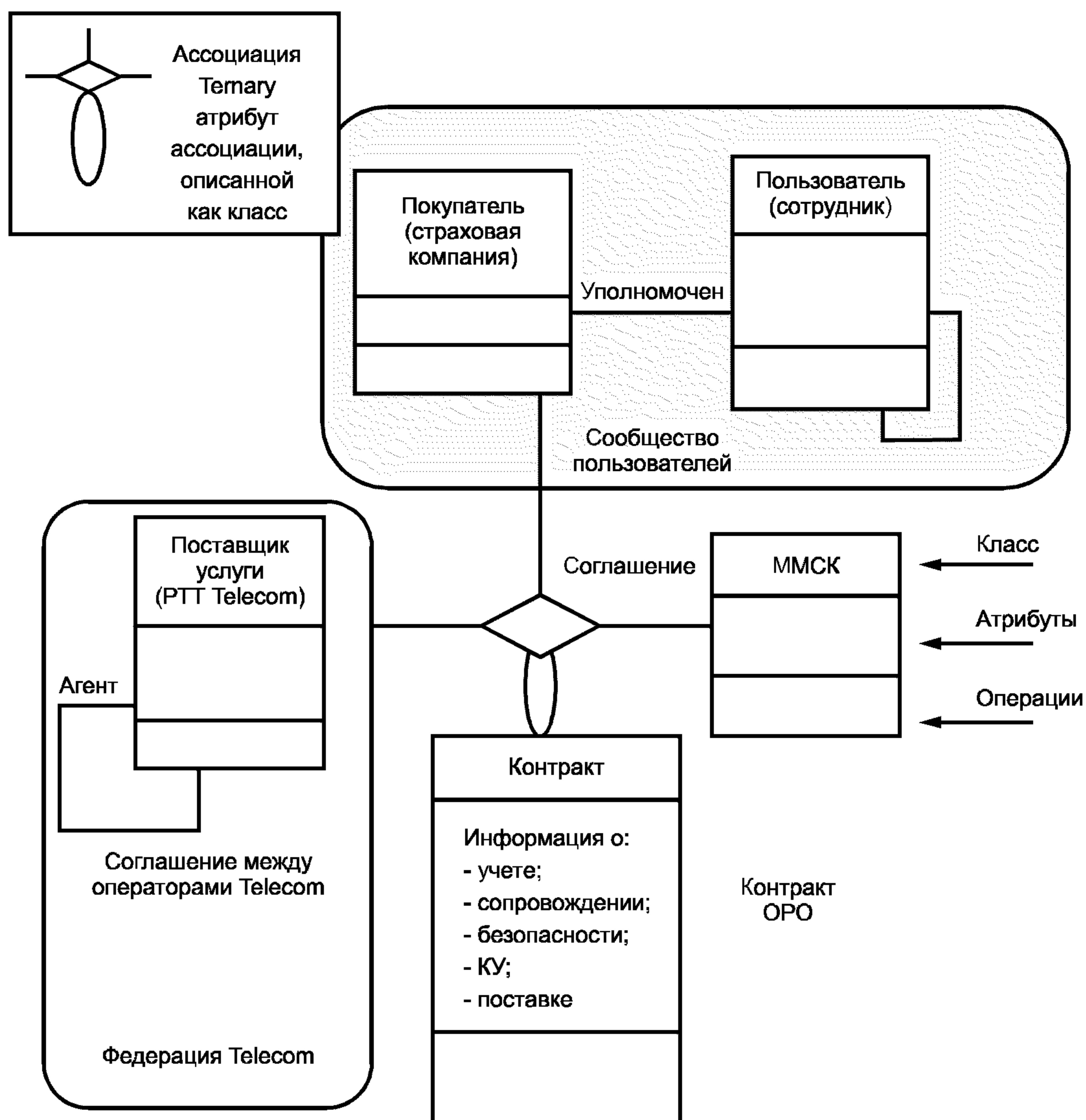
Рисунок 22 — Предпринимательская спецификация ОРО, использующая графические обозначения ММО
