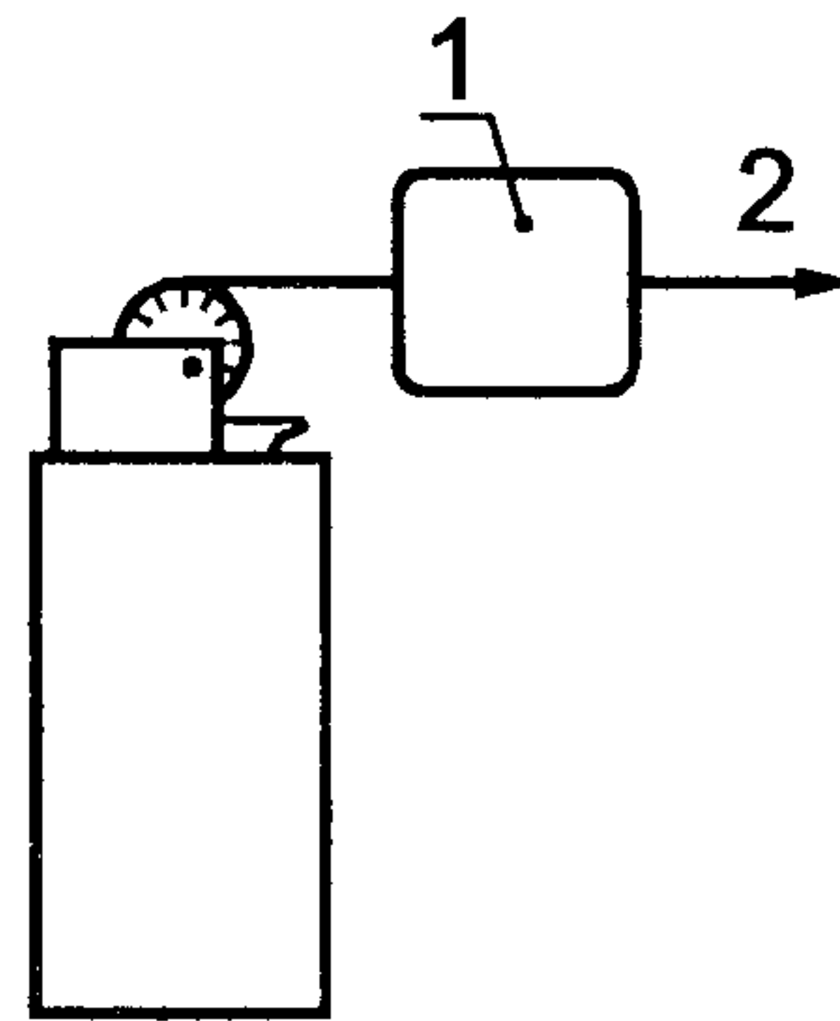
1 — динамометр; 2 — направление приложения усилия
