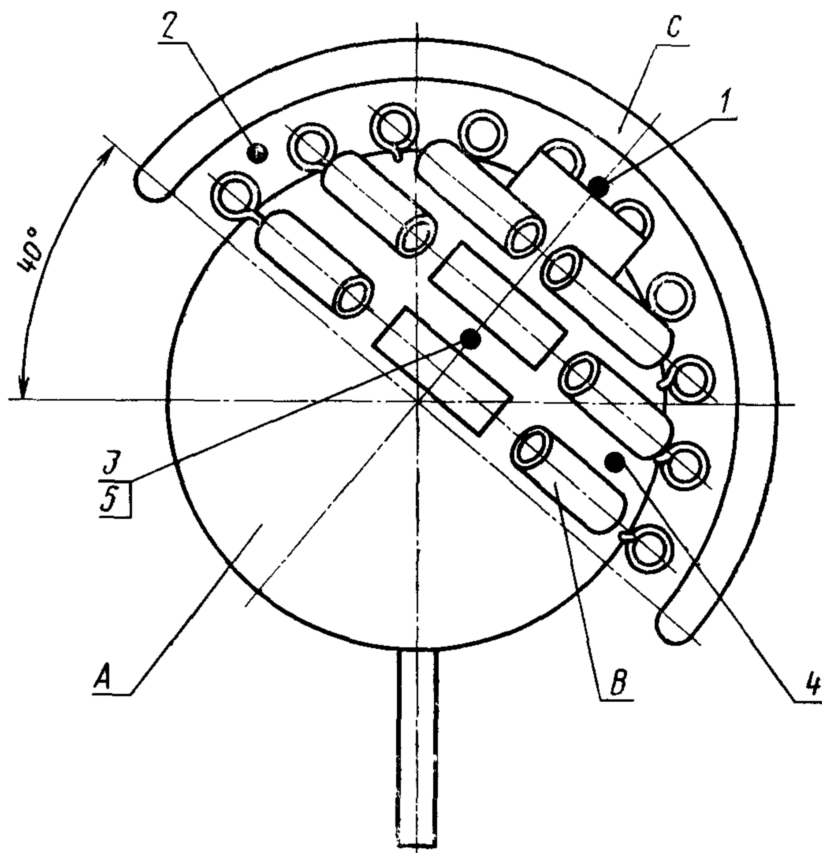
Измерительная головка
