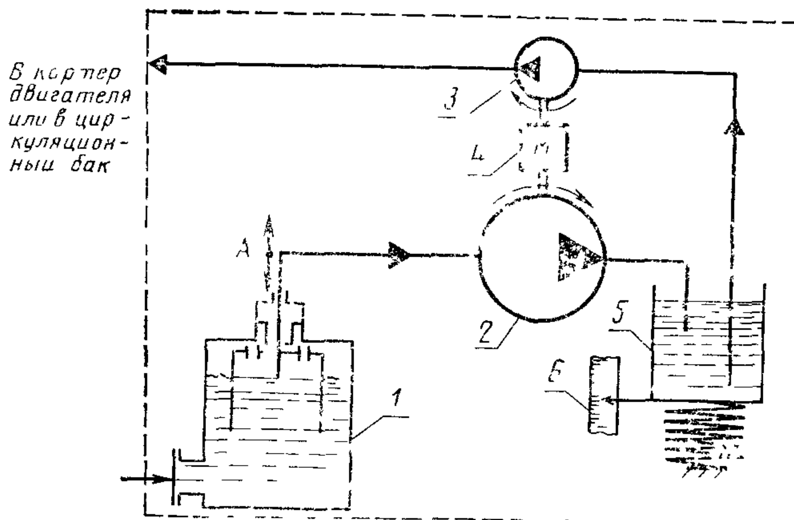
Схема устройства для определения расхода смазочного масла
